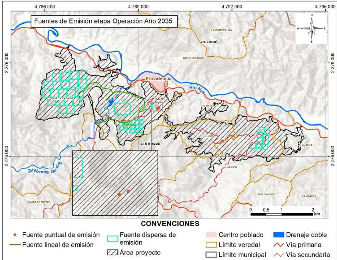
Figura 7.6.73 Fuentes de emisión de ruido año 2035
