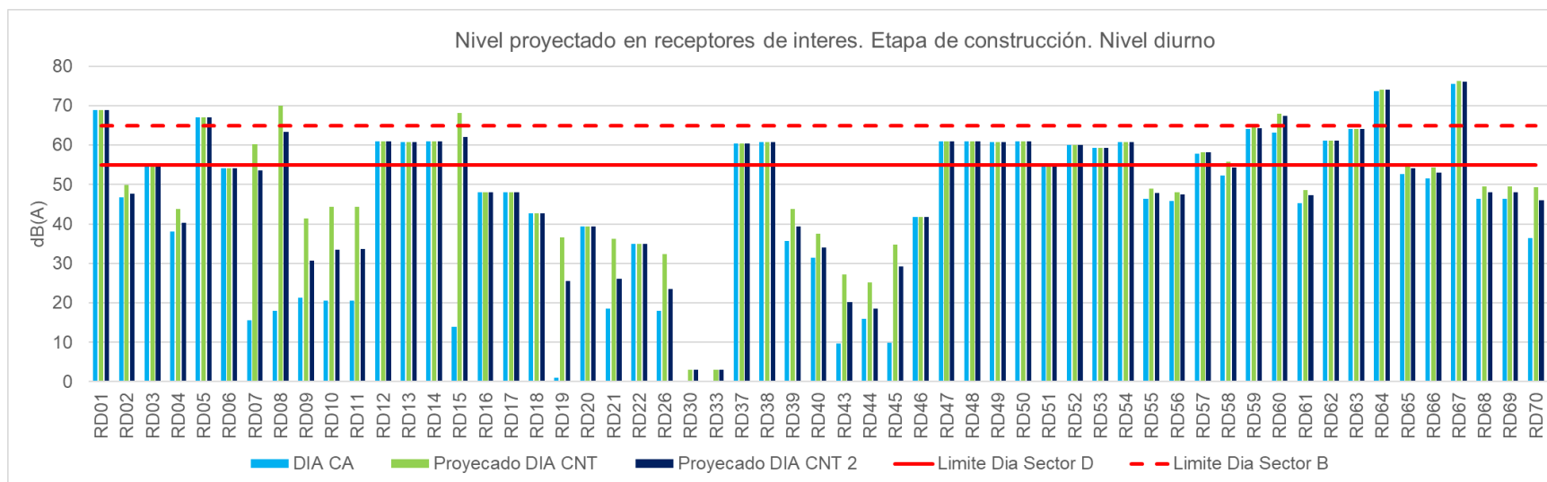
Figura 7.6.102 Niveles proyectados en receptores de interés. Etapa de construcción, periodo diurno
