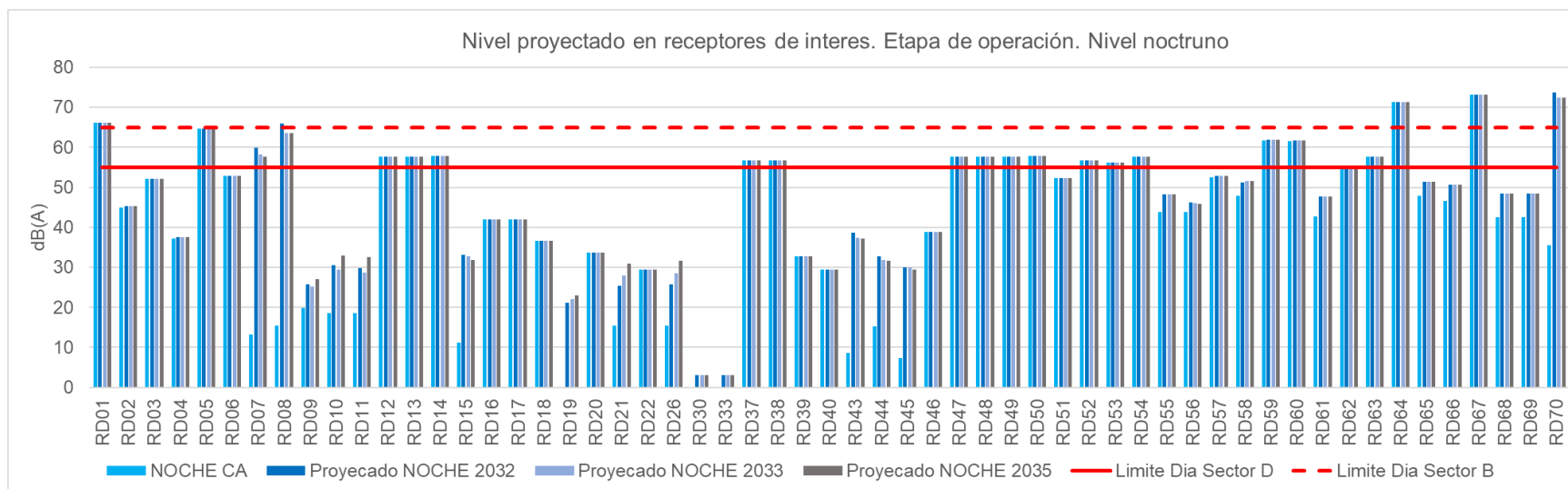
Figura 7.6.104 Niveles proyectados en receptores de interés. Etapa de operación, periodo nocturno
