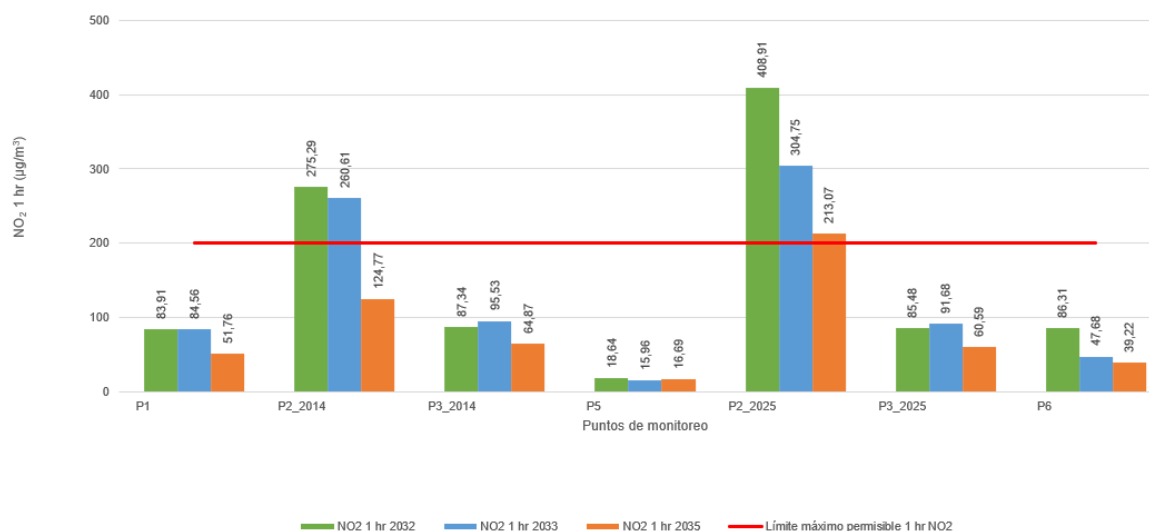
Figura 7.6.17 Aportes máximos 1 hr NO 2 etapa operativa (año 2032 – 2033 – 2035) – fondo incluido
