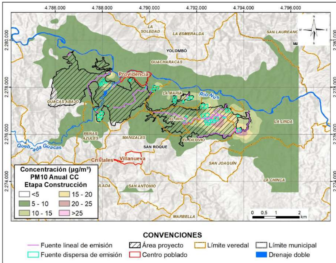
Figura 7.6.21 Isopleta PM10 con medidas de control – concentración promedio anual \mu\text{g}/\text{m}^3 – Etapa constructiva (año 2027)
