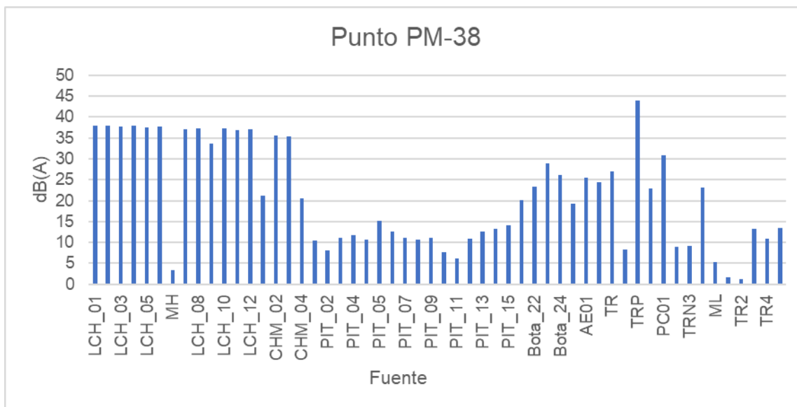
Figura 7.6.92 Nivel parcial de aporte por fuente. PM-38. Nivel nocturno, etapa de operación
