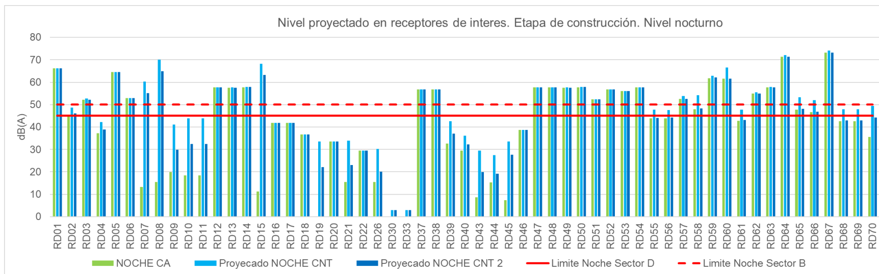
Figura 7.6.103 Niveles proyectados en receptores de interés. Etapa de construcción, periodo nocturno
