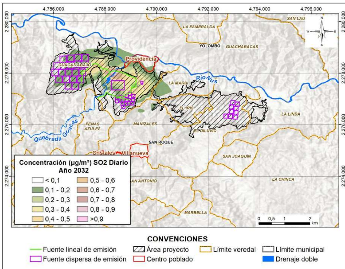
Figura 7.6.64 Isopleta \text{SO}_2 – concentración máxima diaria \mu\text{g}/\text{m}^3 – Etapa operativa (año 2032)
