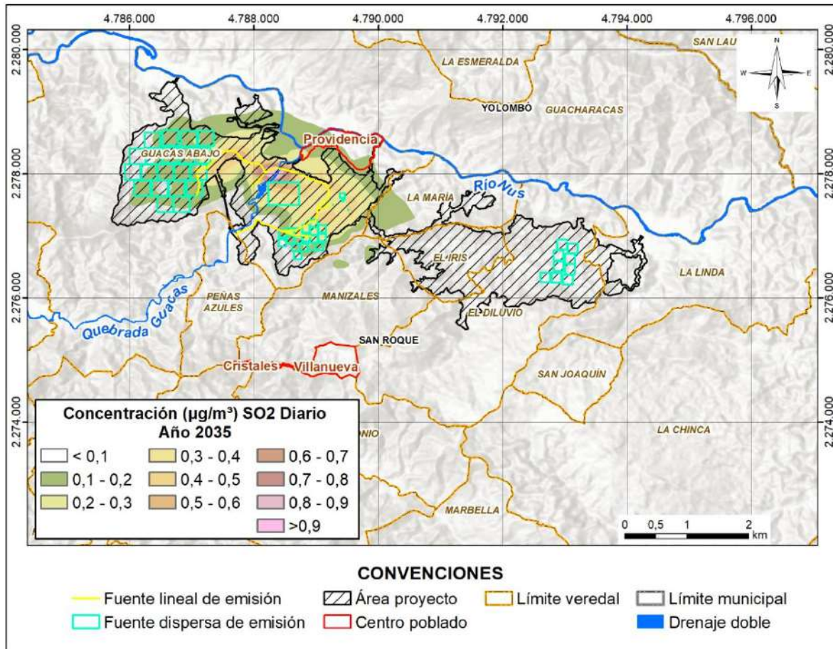
Figura 7.6.68 Isopleta SO 2 – concentración máxima diaria \mu\text{g}/\text{m}^3 – Etapa operativa (año 2035)
