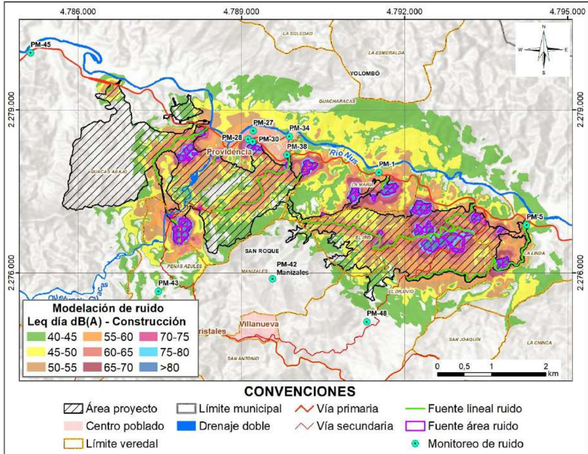
Figura 7.6.86 Leq Dia. Etapa de construcción
