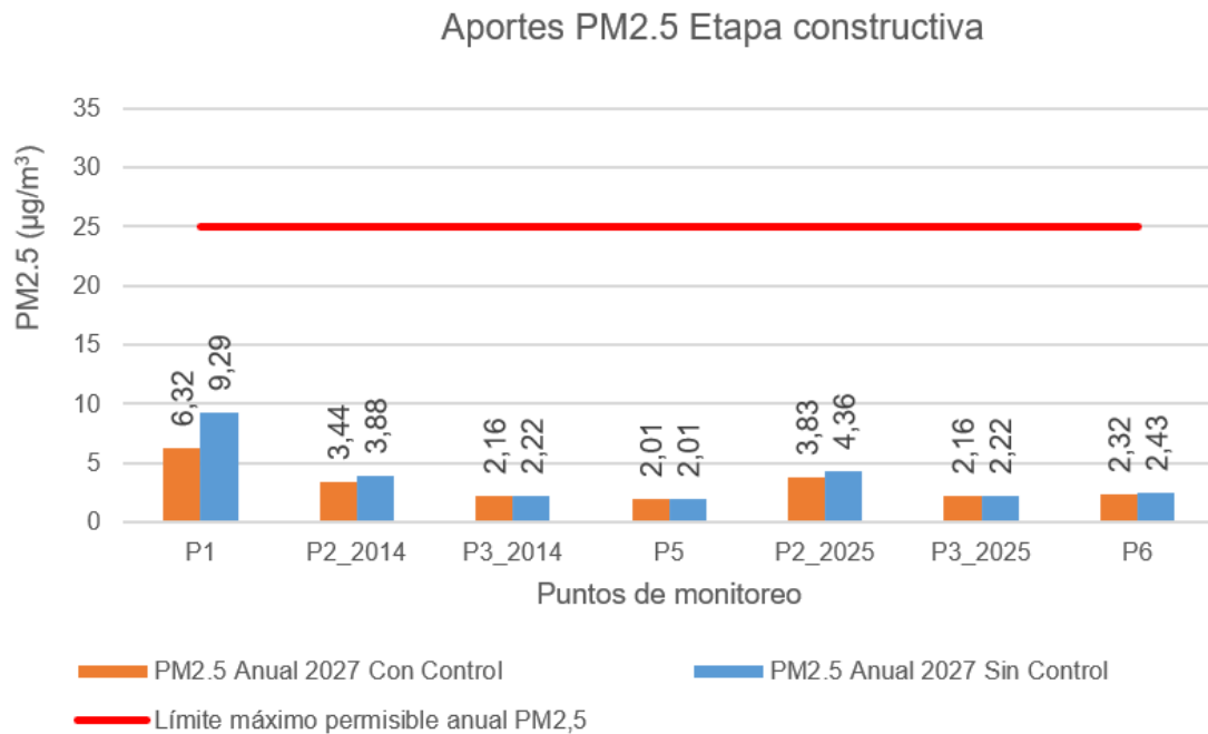
Figura 7.6.5 Aportes anuales PM2.5 etapa constructiva (año 2027) – fondo incluido
