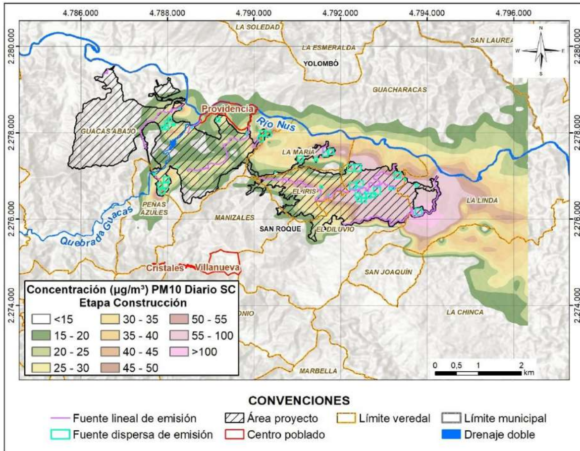
Figura 7.6.24 Isopleta PM10 sin medidas de control – concentración máxima diaria \mu\text{g}/\text{m}^3 – Etapa constructiva (año 2027)
