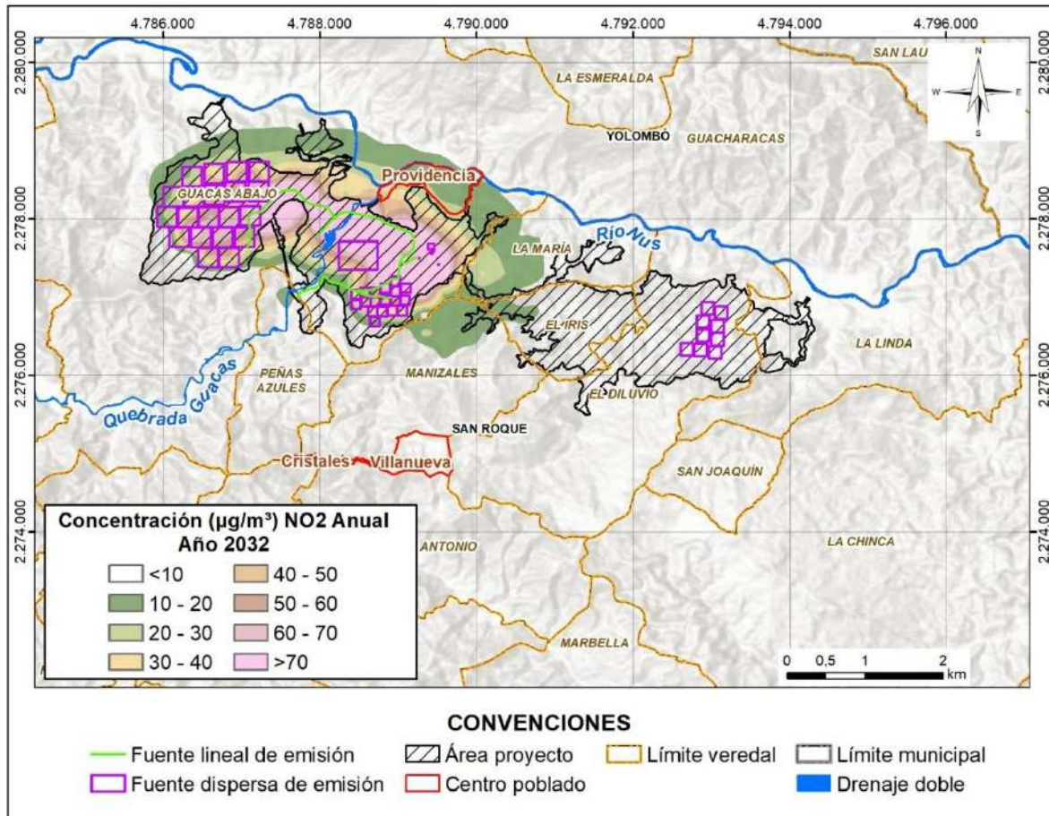
Figura 7.6.55 Isopleta \text{NO}_2 – concentración promedio anual \mu\text{g}/\text{m}^3 – Etapa operativa (año 2032)
