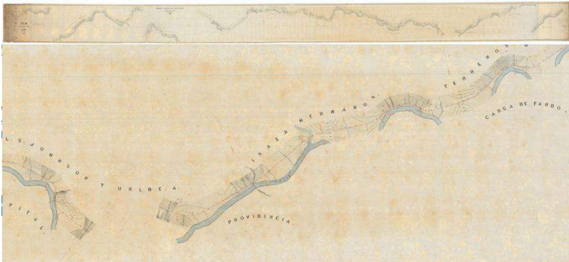
Figura 5.3.24 Plano general y detalle, trazado del Ferrocarril de Antioquia en su paso por el Río Nus, segmento entre lo que hoy es Guacharacas (L.G. Johnson y Uribe A.) y Providencia, 1892
