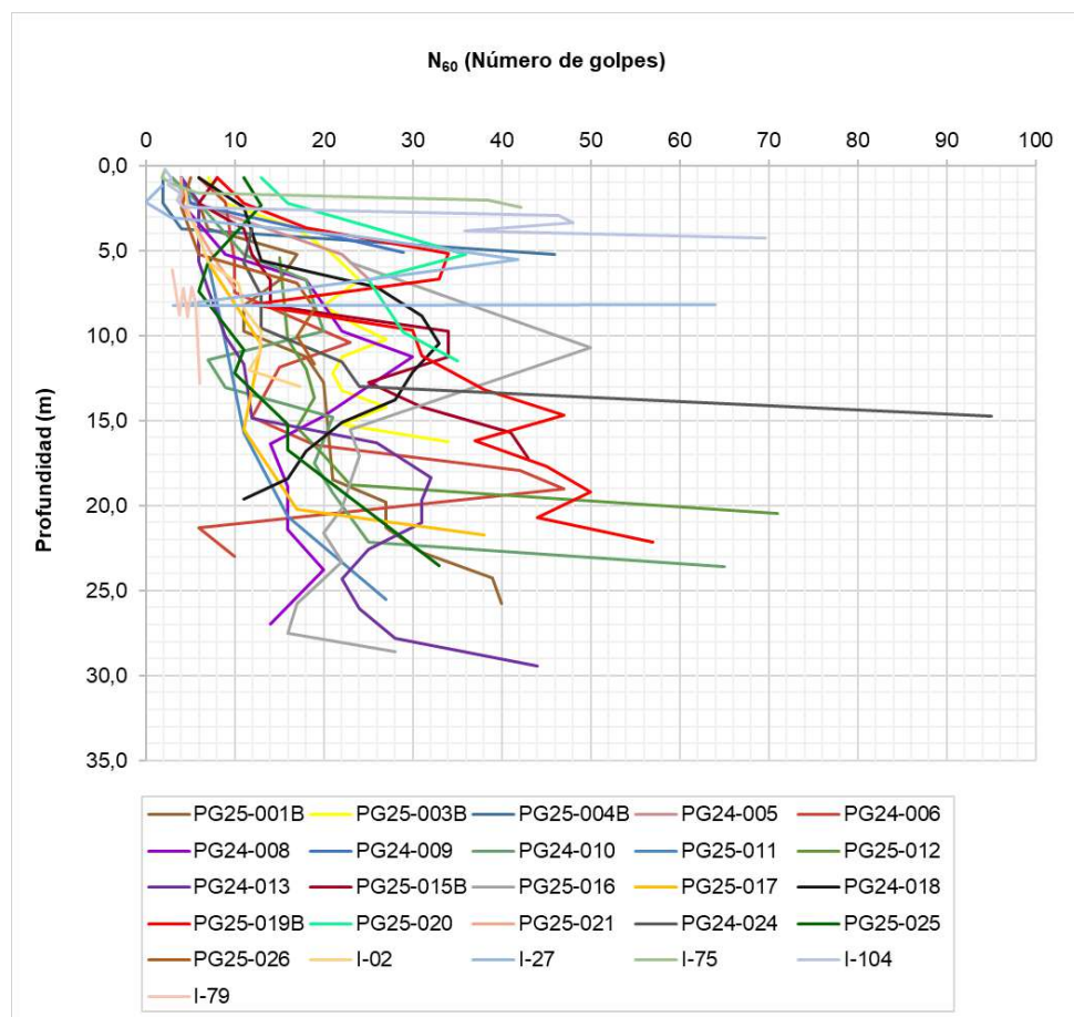
Figura 5.1.7.40 Análisis para las pruebas in situ SPT realizadas para los 26 sondeos en la zona de la Planta Principal.
