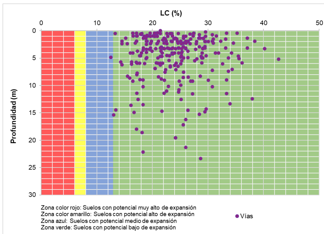
Figura 5.1.7.37 Resultados límites de contracción en los diferentes trazados viales
