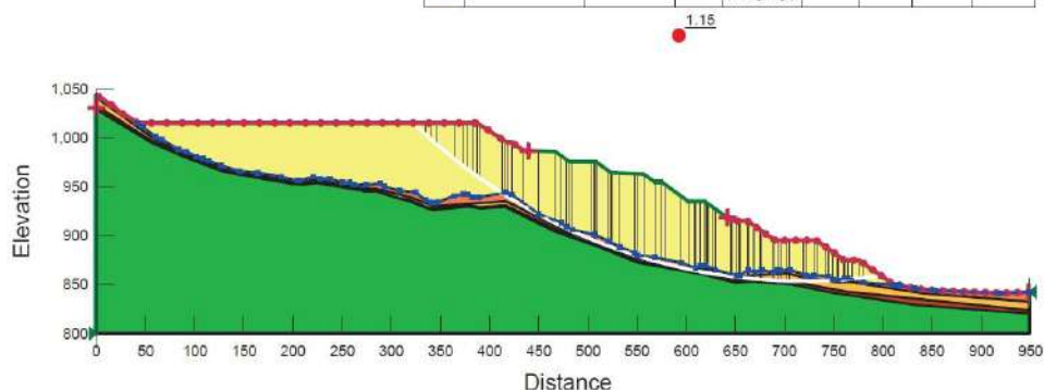
Figura 5.5.1.7.181 Análisis de estabilidad en condición pseudoestática de la Sección B – Depósito El Balsal, etapa de operación máxima
