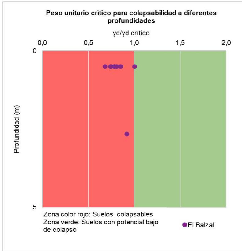
Figura 5.1.7.72 Resultados de colapsabilidad-Sector El Balsal
