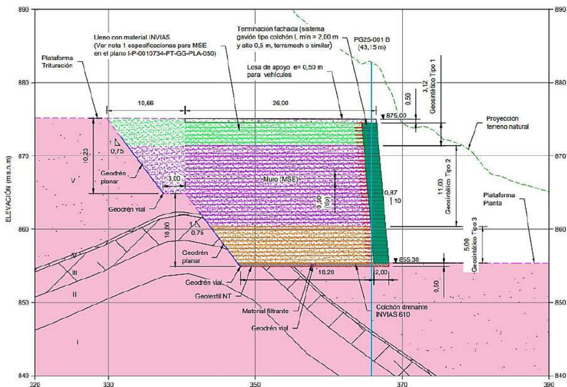
Figura 5.1.7.127 Esquema del muro en suelo mecánicamente estabilizado
