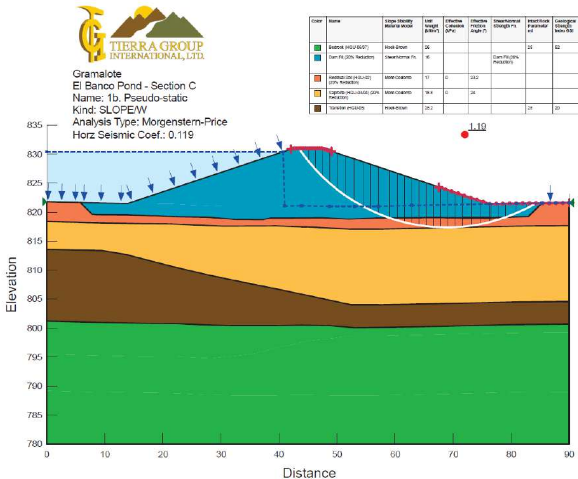
Figura 5.5.1.7.187 Análisis de estabilidad en condición pseudoestática de la Sección C – Presa del Sedimentador El Banco
