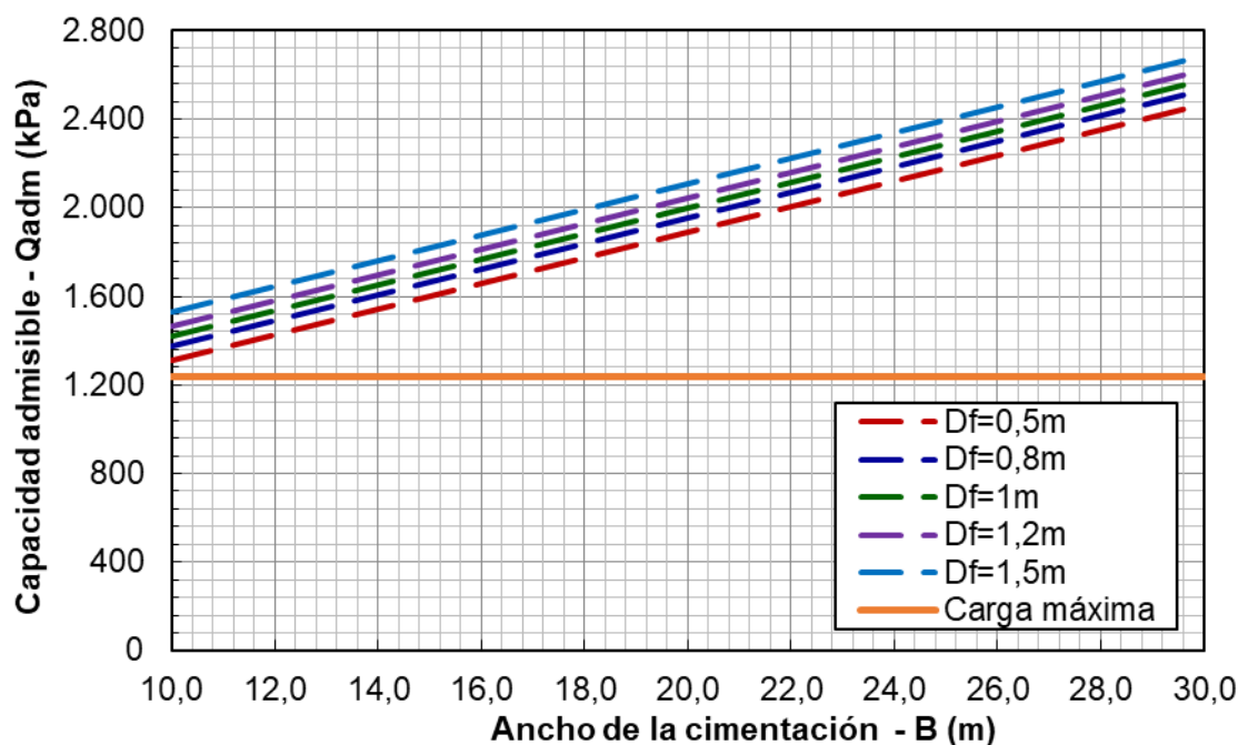
Figura 5.1.7.207 Ábaco capacidad de soporte admisible por cortante para el depósito K en condiciones de servicio
