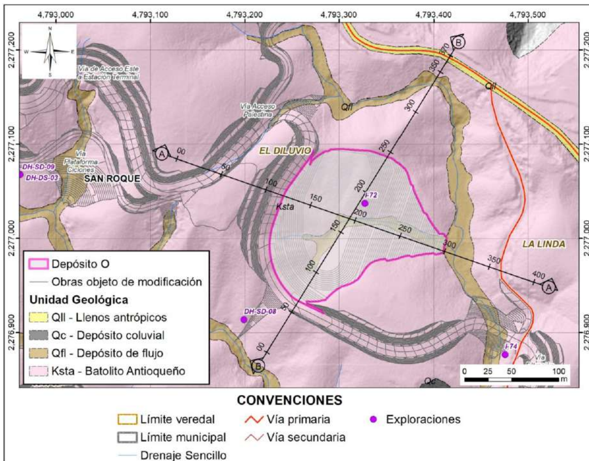
Figura 5.1.7.161 Localización en planta del depósito O con las secciones de interés para los análisis geotécnicos
