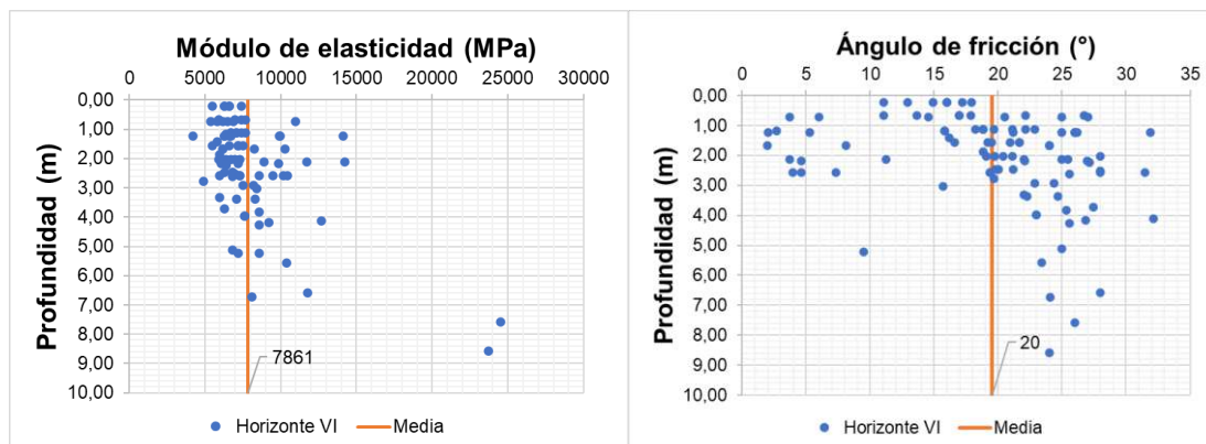
Figura 5.1.7.32 Horizonte VI: Análisis de las correlaciones entre el SPT y el módulo de elasticidad (izquierda); el SPT y el ángulo de fricción (derecha)
