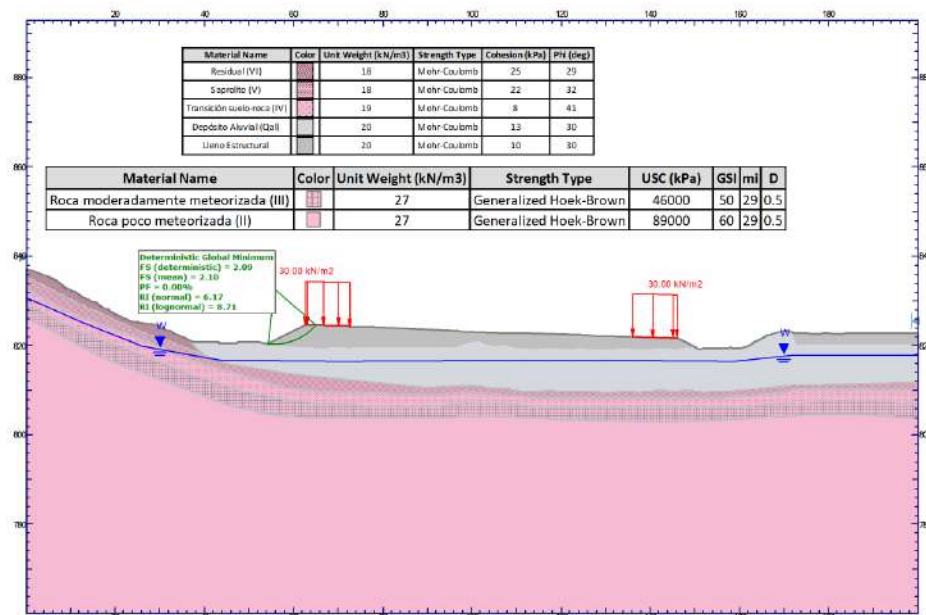
Figura 5.1.7.141 Análisis de estabilidad izquierdo en condición estática con nivel freático normal de la plataforma La Mayoría – Sección C
