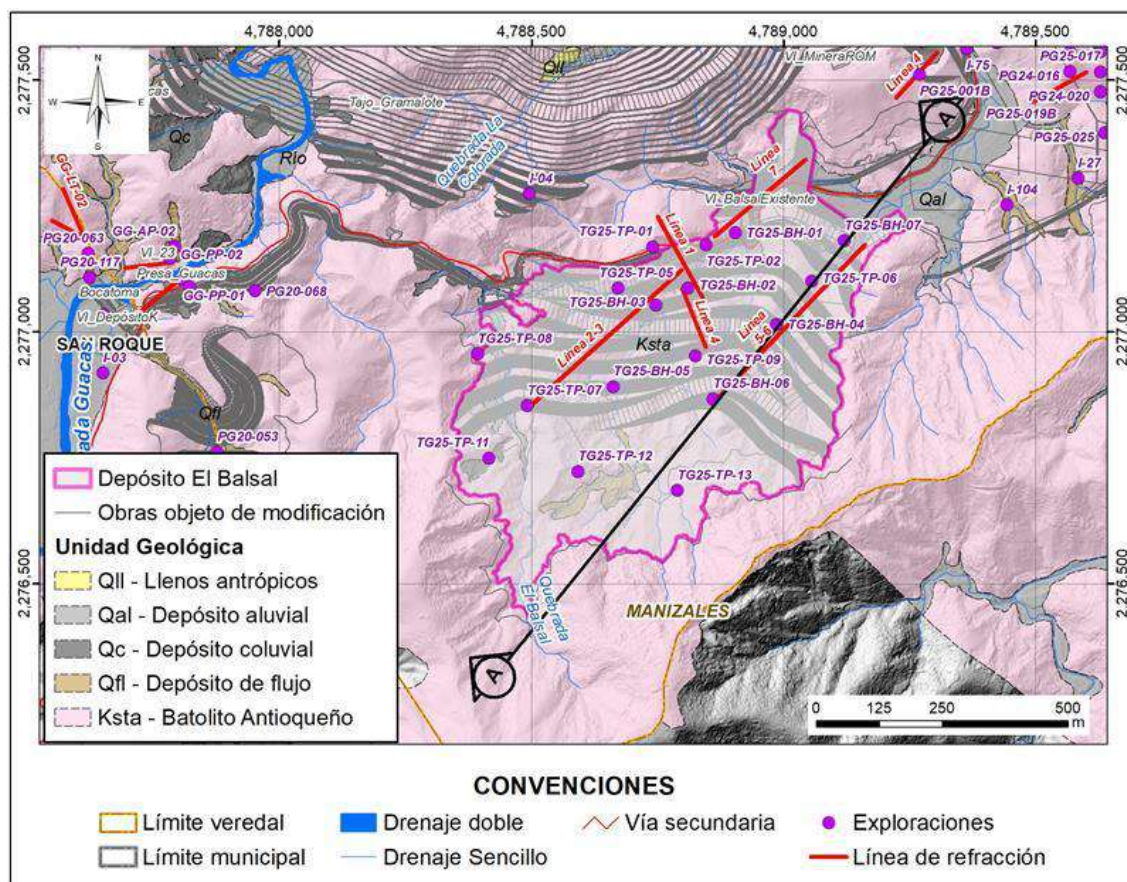
Figura 5.5.1.7.179 Localización en planta de la sección de interés para el análisis geotécnico – Depósito El Balsal
