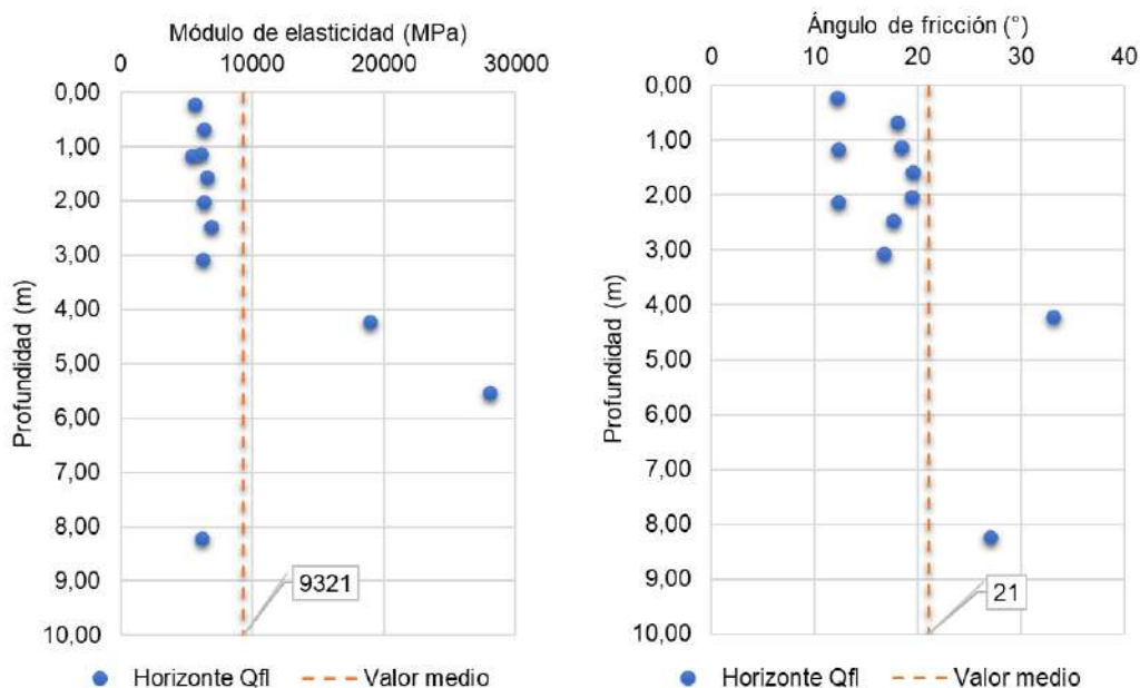
Figura 5.1.7.45 Depósito de flujo: Análisis de las correlaciones entre el SPT y el módulo de elasticidad (izquierda); el SPT y el ángulo de fricción (derecha)
