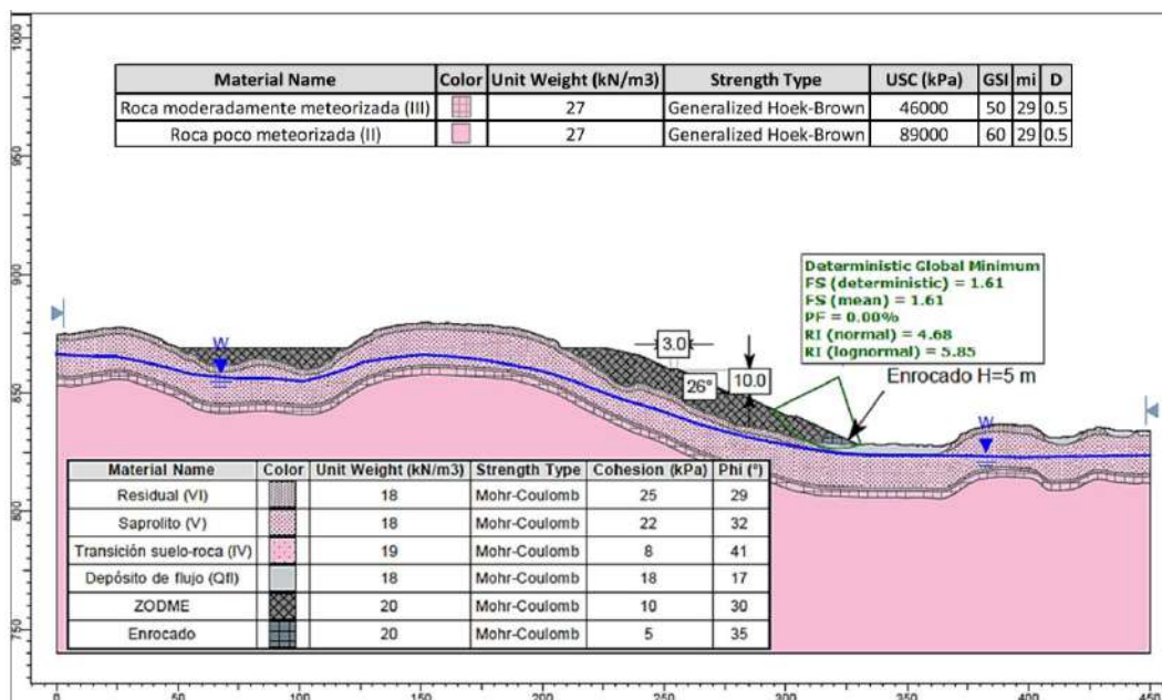
Figura 5.1.7.149 Análisis de estabilidad en condición estática con nivel freático normal de la Sección A – Depósito E
