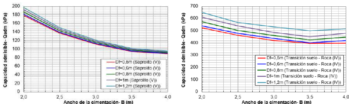
Figura 5.1.7.199 Ábaco capacidad de soporte admisible – Vertedero de excesos de la presa del sedimentador La Colorada – Servicio restringida por asentamiento en el horizonte V (izquierda) y IV (derecha)
