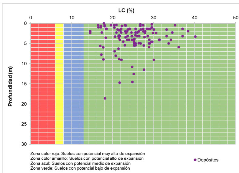
Figura 5.1.7.63 Resultados límites de contracción en los depósitos
