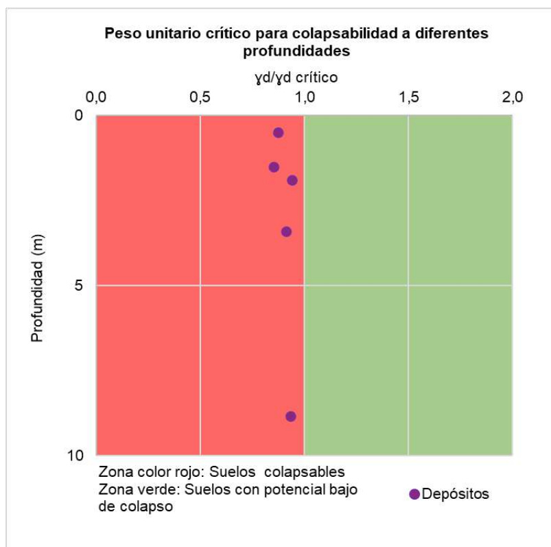
Figura 5.1.7.64 Resultados de colapsabilidad en los depósitos
