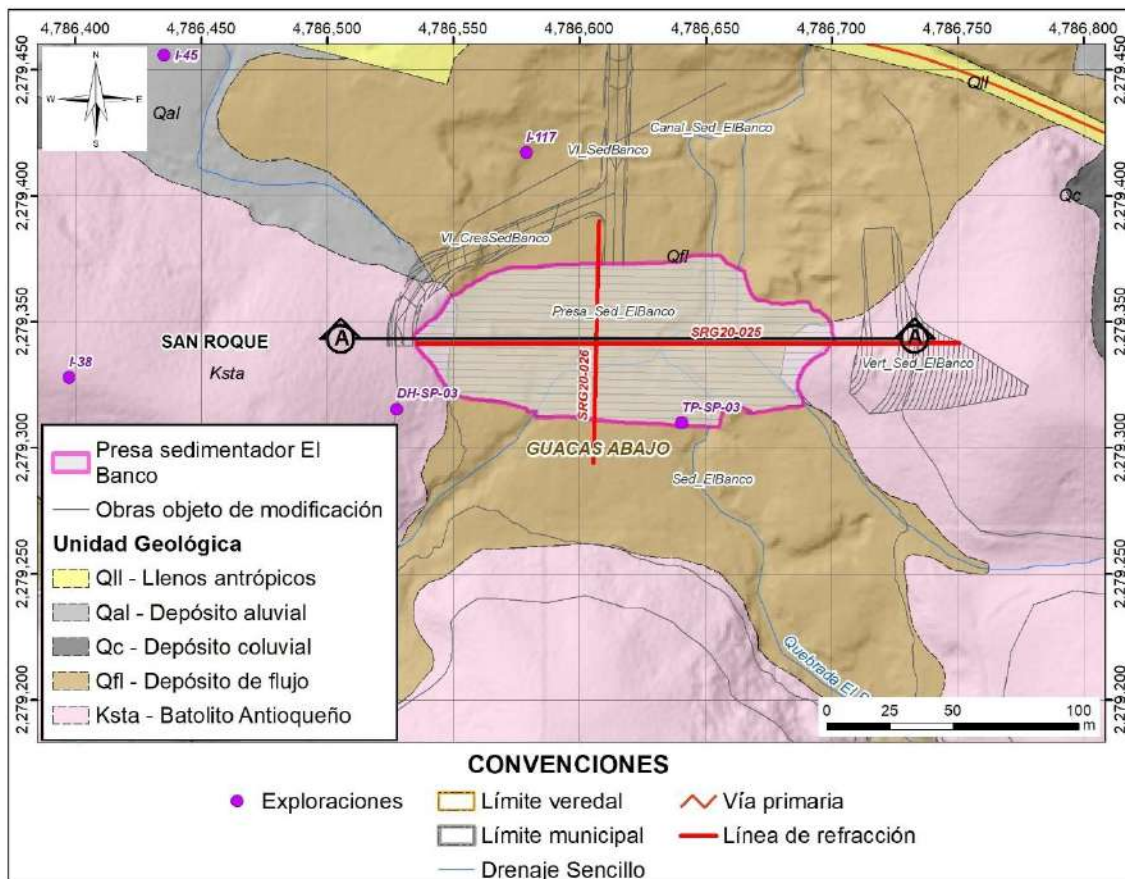
Figura 5.5.1.7.185 Localización en planta de la sección de interés para el análisis geotécnico – Presa del Sedimentador El Banco
