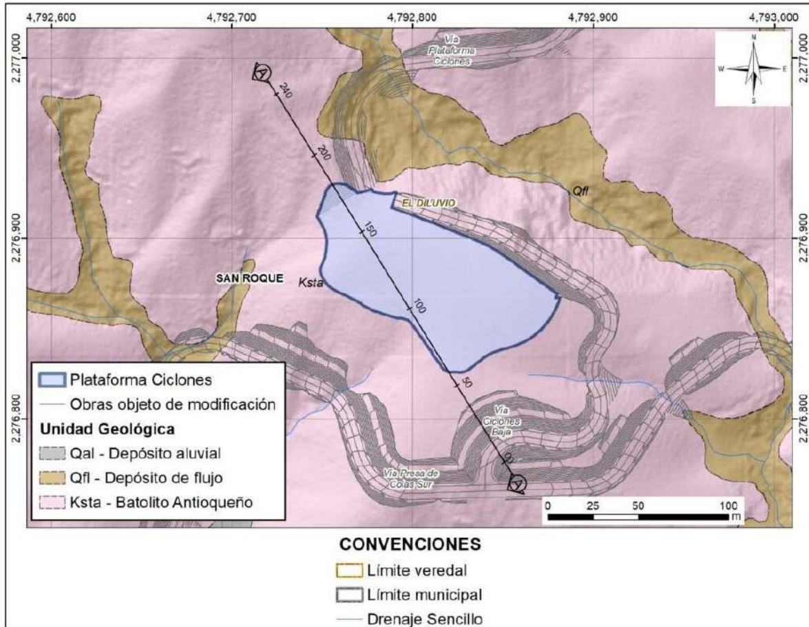
Figura 5.1.7.131 Localización en planta de la plataforma Ciclonés con la sección de interés para el análisis geotécnico
