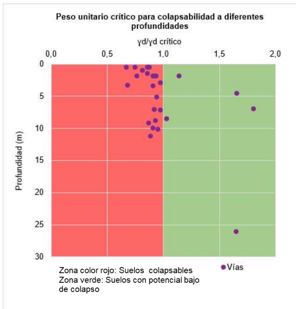
Figura 5.1.7.38 Resultados de colapsabilidad en la en los diferentes trazados viales.
