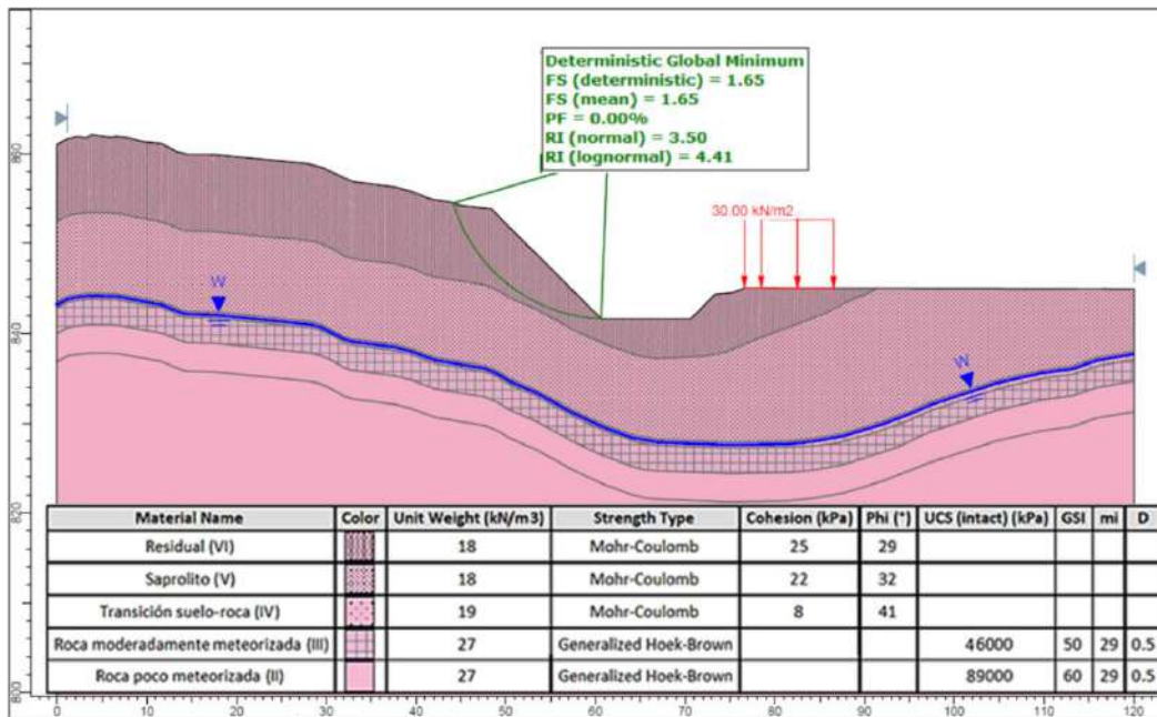
Figura 5.1.7.135 Análisis de estabilidad en condición estática con nivel freático normal del talud izquierdo de la plataforma de la EBAR
