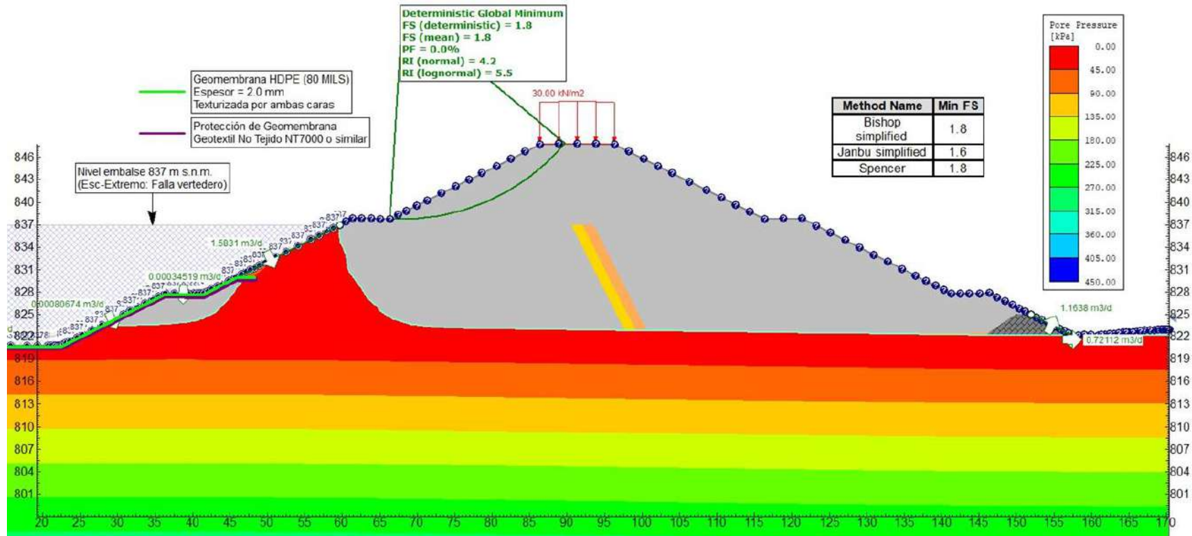
Figura 5.1.7.116 Comportamiento hidráulico de la presa del sedimentador La Colorada. Presiones de poros y condición de estabilidad espaldón aguas arriba. Condición extrema: fallo del vertedero de excesos. Sección B – km 0+820
