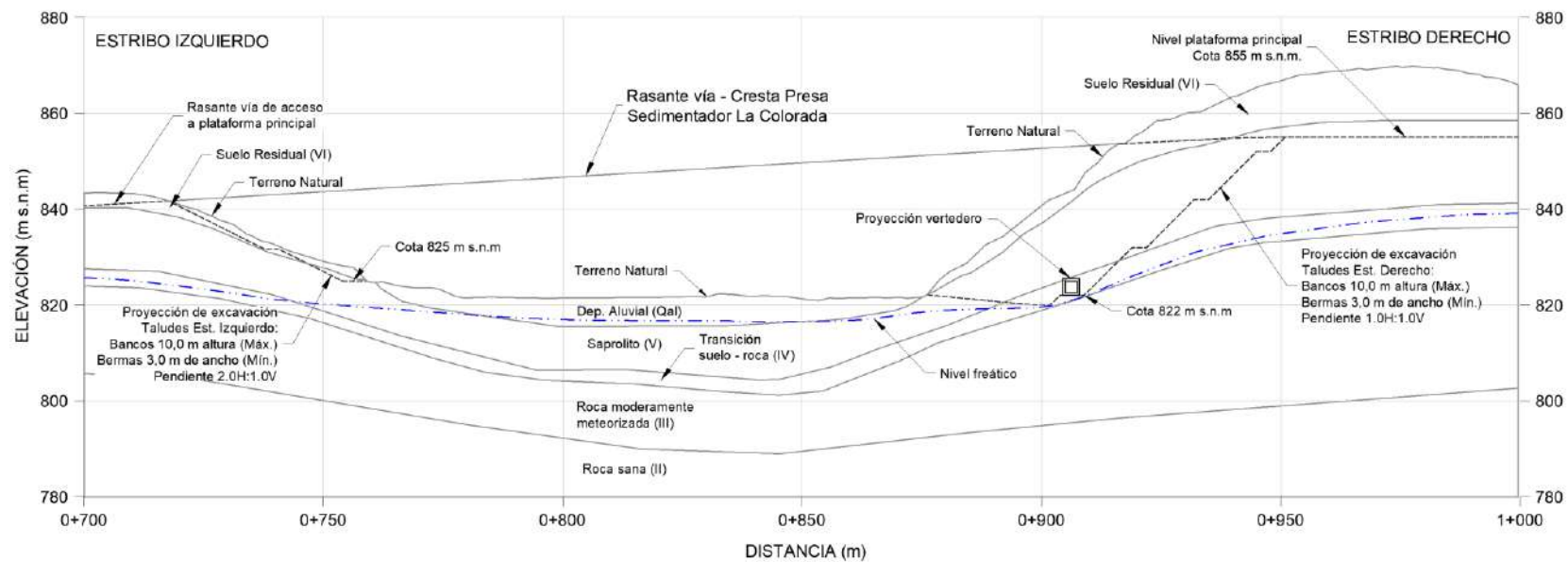
Figura 5.1.7.110 Perfil longitudinal Sección A-A'. Proyección de excavación de los estribos de la presa del sedimentador La Colorada
