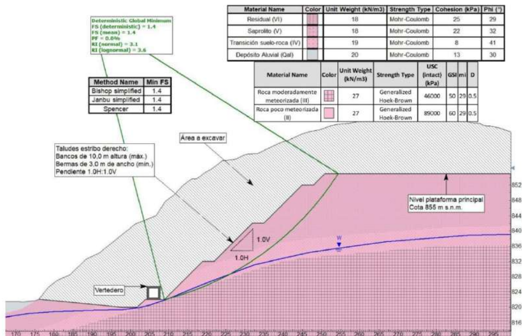
Figura 5.1.7.111 Análisis de estabilidad en condición estática con nivel freático normal. Estribo derecho presa del sedimentador La Colorada (Etapa 1 – Excavación temporal)
