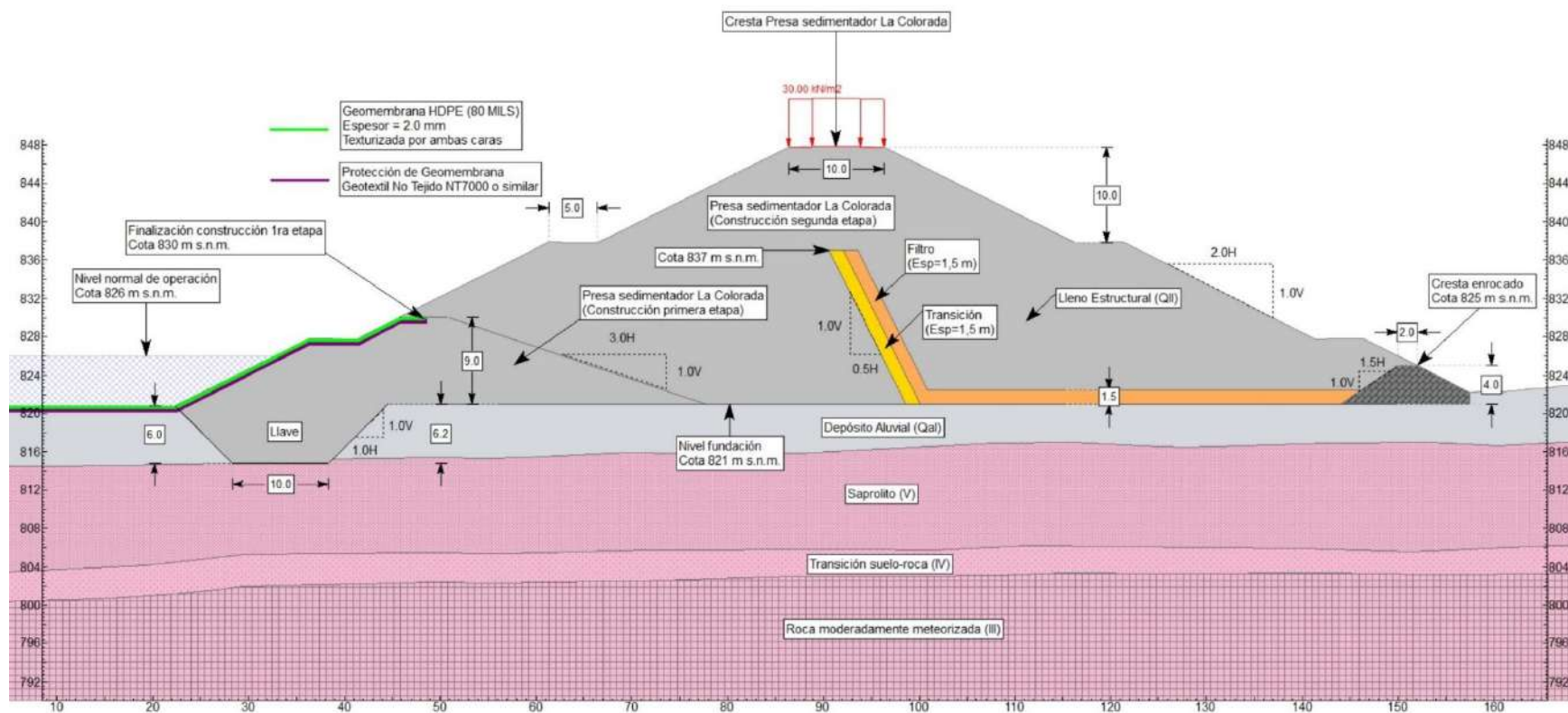
Figura 5.1.7.104 Sección transversal típica (Sec-B km 0+820) de la presa del sedimentador La Colorada
