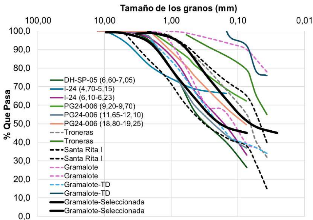
Figura 5.1.7.118 Límites granulométricos para el material de conformación de la presa La Colorada
