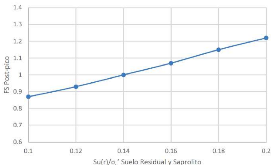
Figura 5.5.1.7.196 Análisis de sensibilidad post-pico – Presa Sedimentador El Banco
