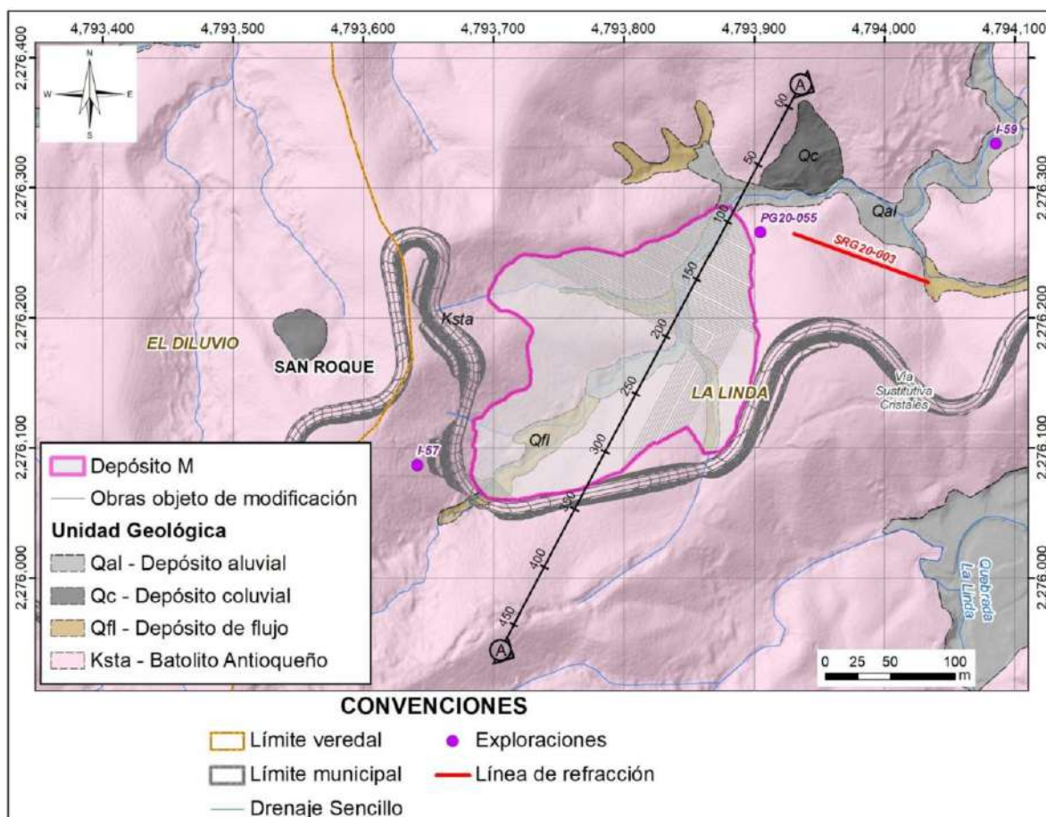
Figura 5.1.7.159 Localización en planta del depósito M con la sección de interés para el análisis geotécnico
