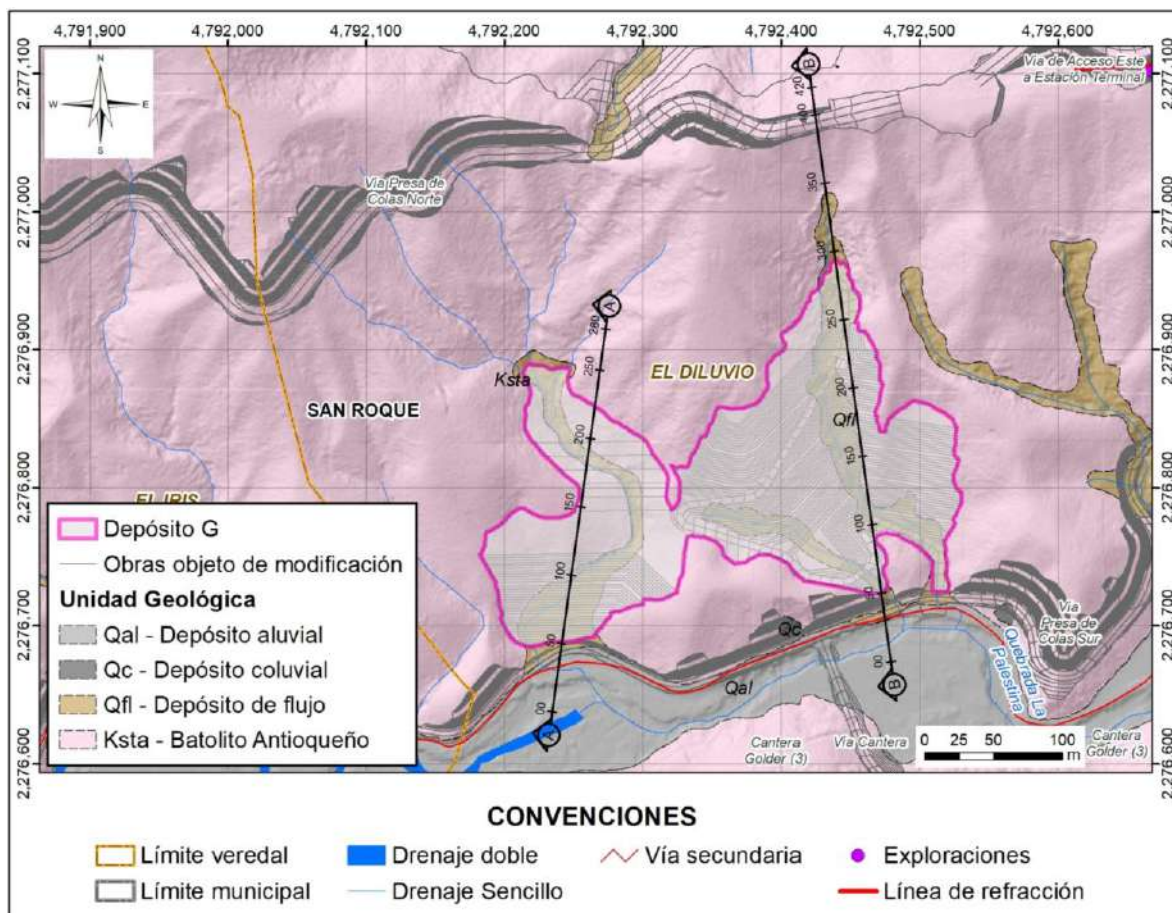
Figura 5.1.7.150 Localización en planta del depósito G con las secciones de interés para los análisis geotécnicos
