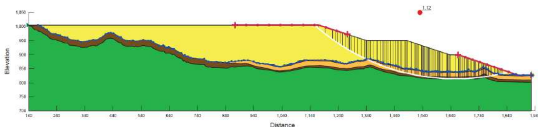
Figura 5.5.1.7.178 Análisis de estabilidad al cierre en condición pseudoestática de la Sección A – Depósito San Antonio, etapa de cierre
