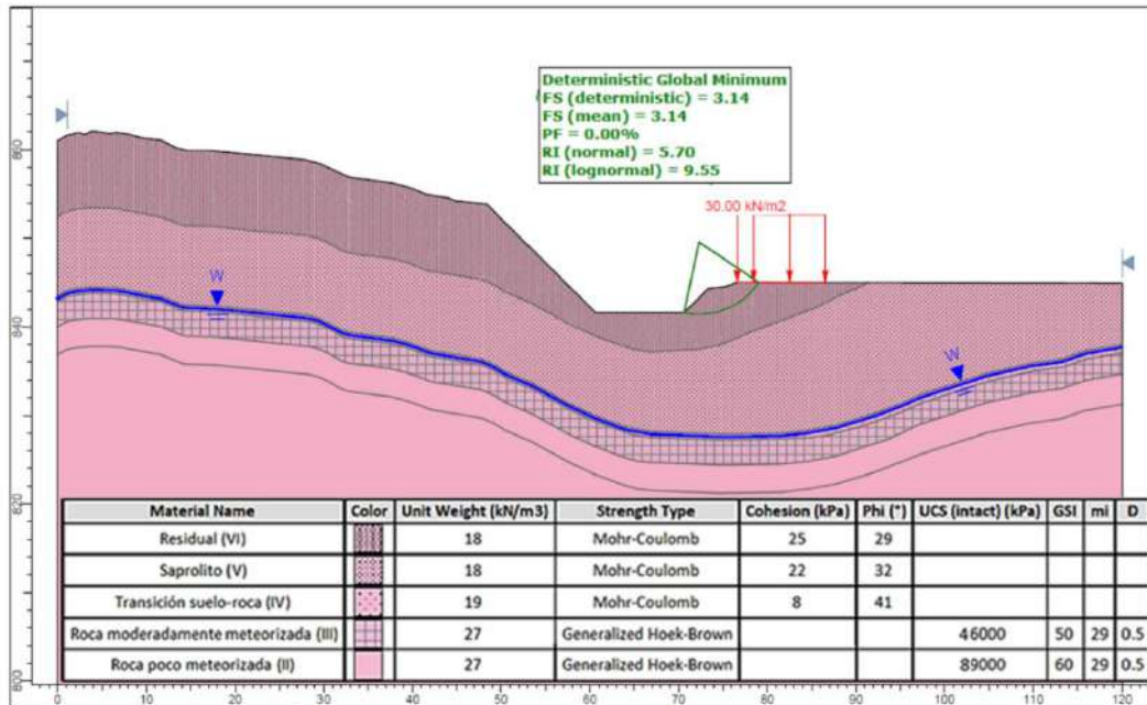
Figura 5.1.7.134 Análisis de estabilidad en condición estática con nivel freático normal del talud derecho de la plataforma de la EBAR
