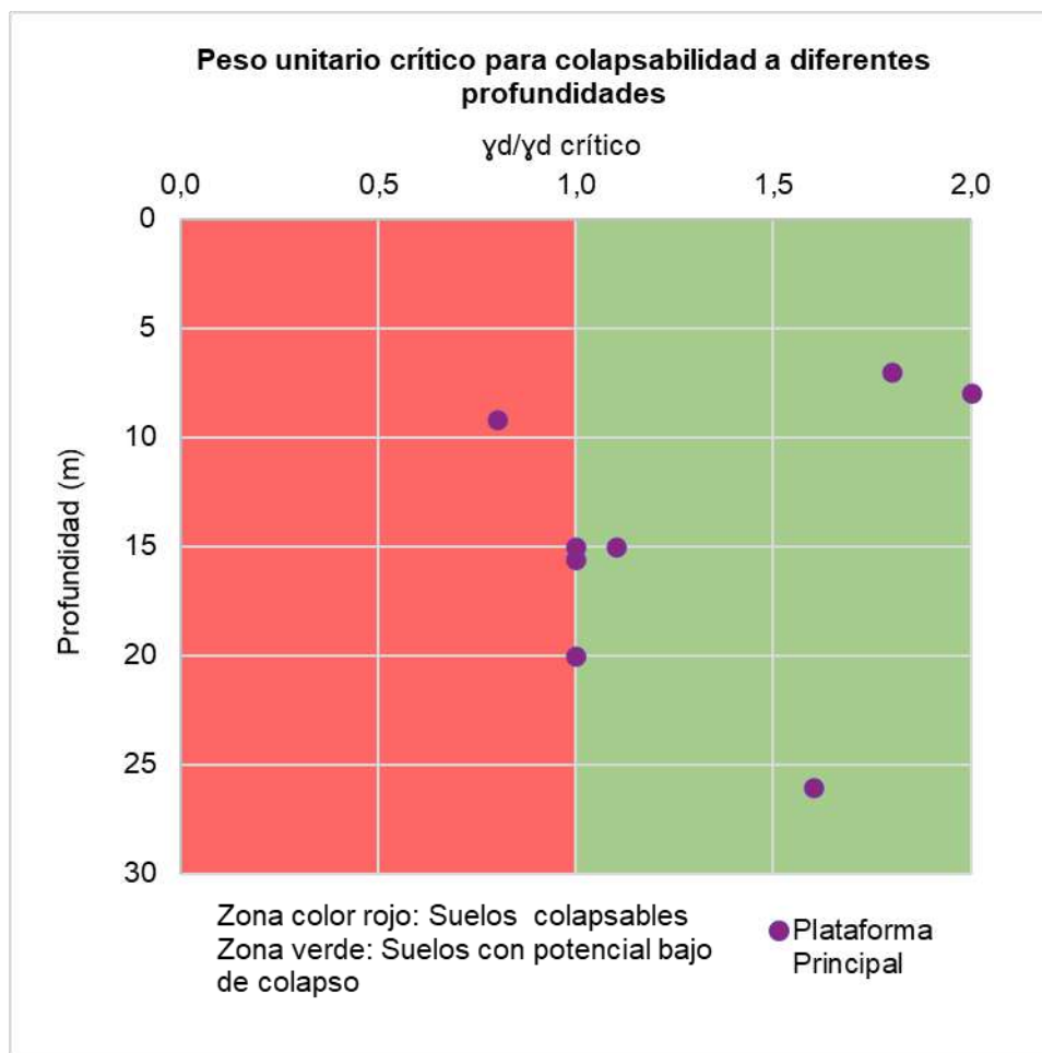
Figura 5.1.7.47 Resultados de colapsabilidad en la Plataforma Principal
