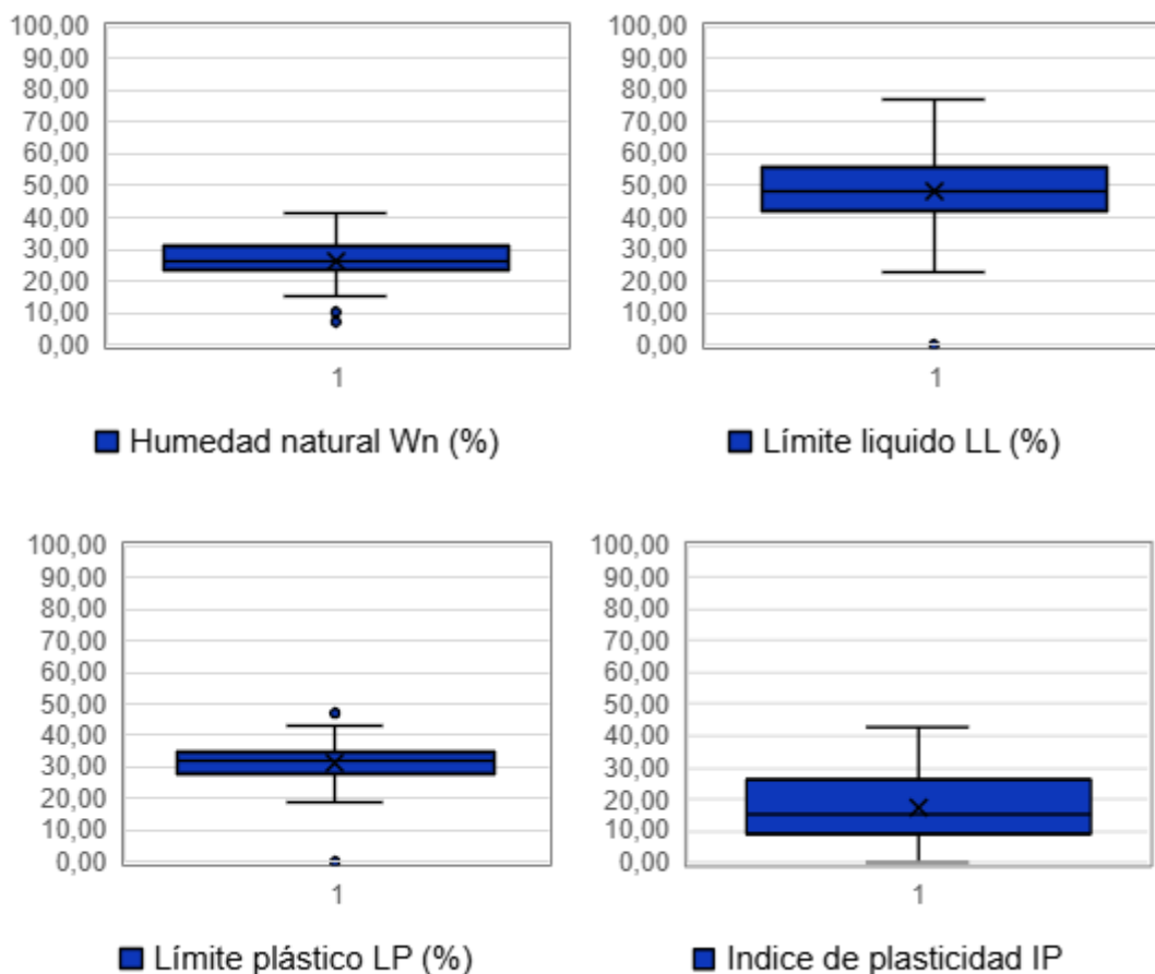
Figura 5.1.7.77 Horizonte VI: Análisis de humedad natural y límites de la base de datos general. Wn% (82 datos), LL (72 datos), LP (78 datos), IP (78 datos)
