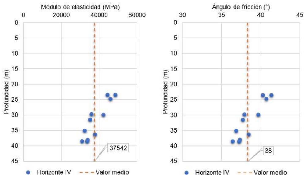
Figura 5.1.7.43 Horizonte IV: Análisis de las correlaciones entre el SPT y el módulo de elasticidad (izquierda); el SPT y el ángulo de fricción (derecha)
