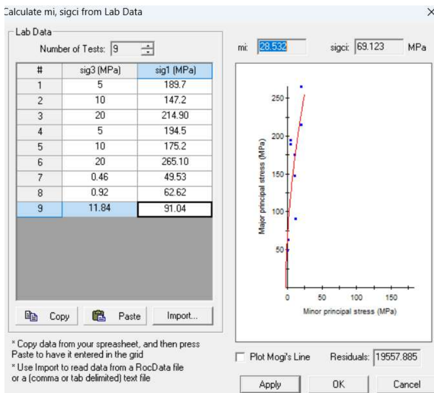
Figura 5.1.7.92 Estimación del parámetro m_i
