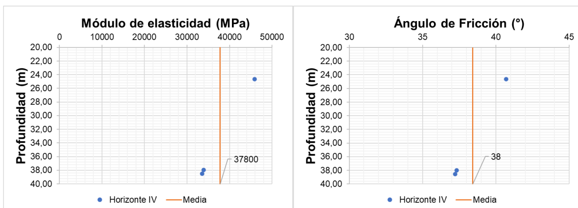
Figura 5.1.7.34 Horizonte IV: Análisis de las correlaciones entre el SPT y el módulo de elasticidad (izquierda); el SPT y el ángulo de fricción (derecha)
