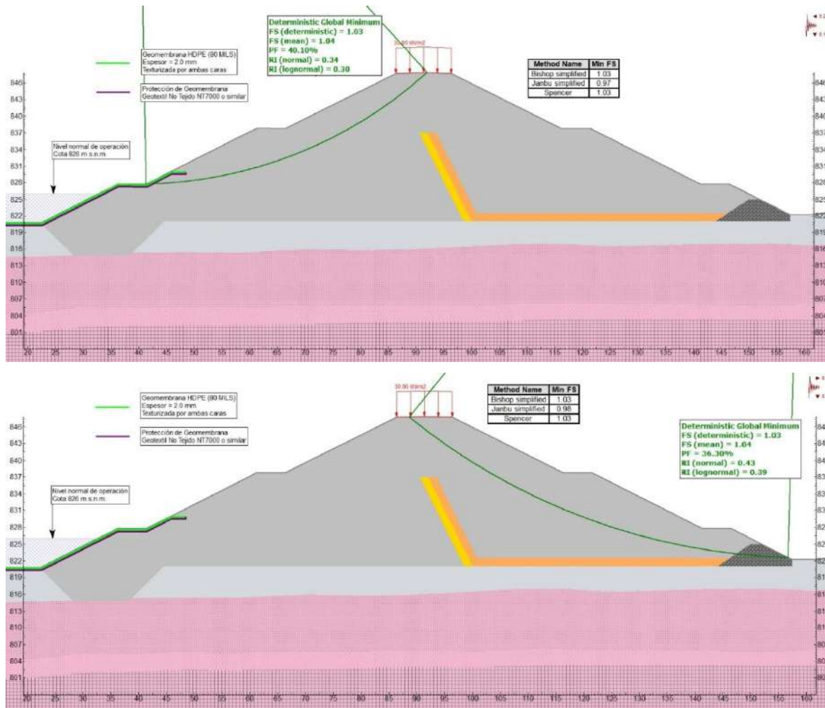
Figura 5.1.7.108 Condición largo plazo. Espaldón aguas arriba y aguas abajo de la presa del sedimentador La Colorada. Análisis pseudoestático (sismo Tr 2475 años) con el nivel normal de operación del embalse. Sección B – km 0+820
