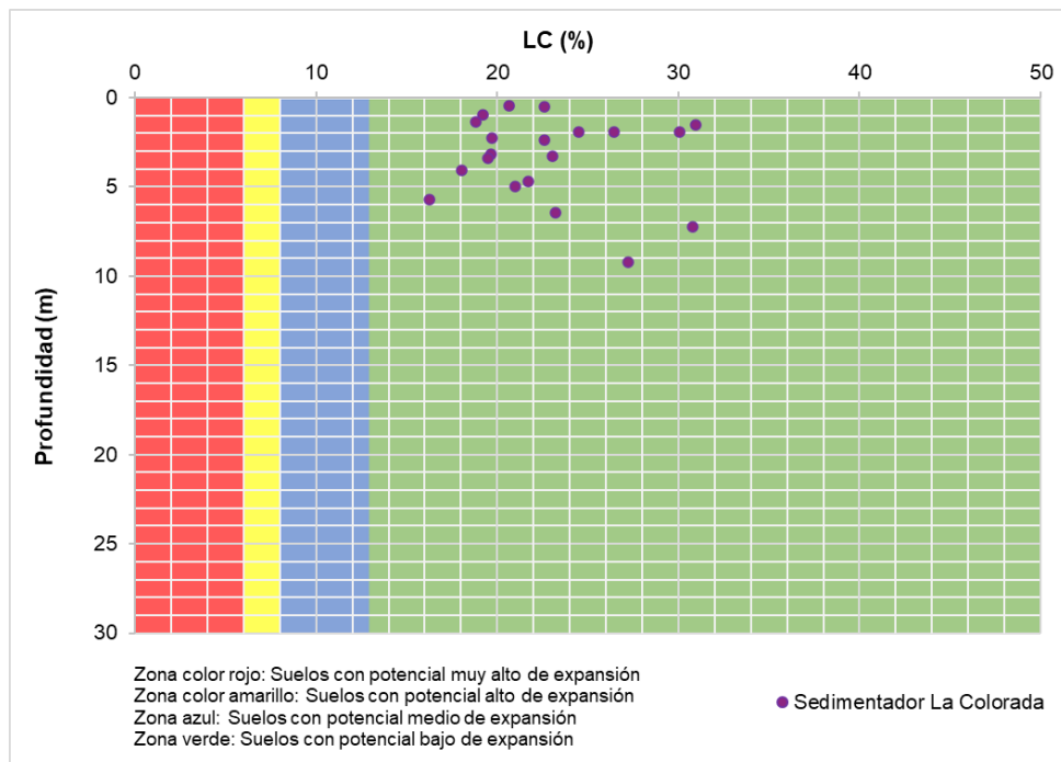
Figura 5.1.7.27 Resultados límites de contracción general del proyecto
