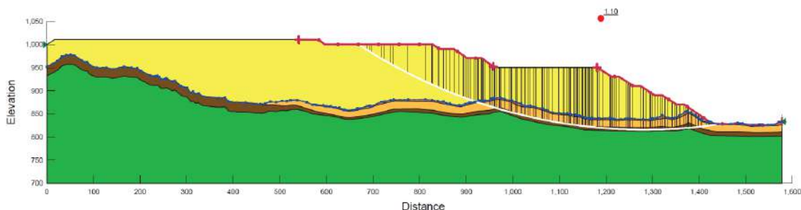
Figura 5.5.1.7.175 Análisis de estabilidad en condición pseudoestática de la Sección A – Depósito San Antonio, operación máxima
