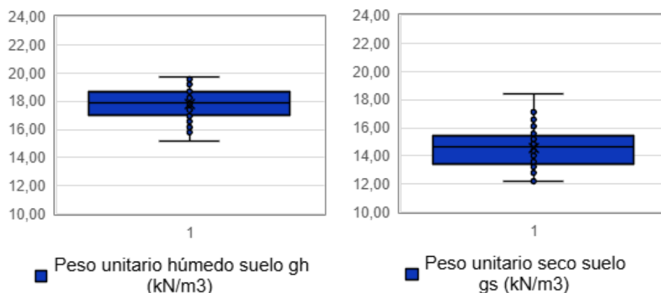
Figura 5.1.7.84 Horizonte V: Análisis de los pesos unitarios reportados en la base de datos general. Número de datos 38
