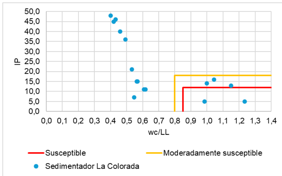
Figura 5.1.7.29 Análisis de licuación o licuefacción de muestras de suelo – Sedimentador La Colorada. Método de Bray y Sancio (2006)
