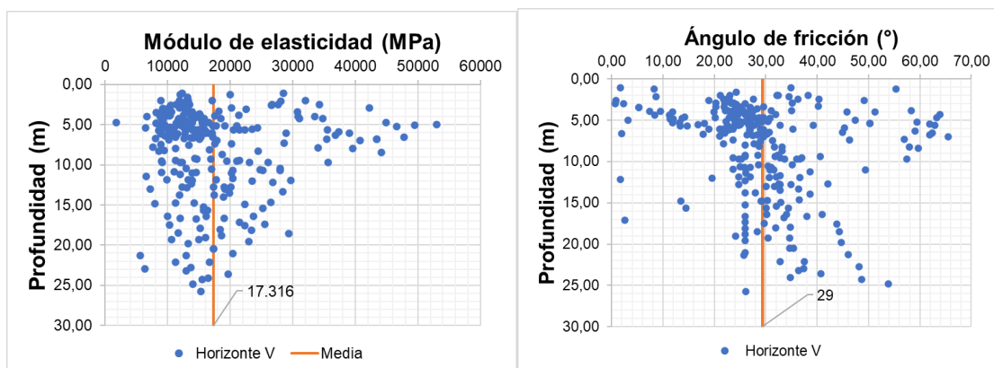
Figura 5.1.7.33 Horizonte V: Análisis de las correlaciones entre el SPT y el módulo de elasticidad (izquierda); el SPT y el ángulo de fricción (derecha)
