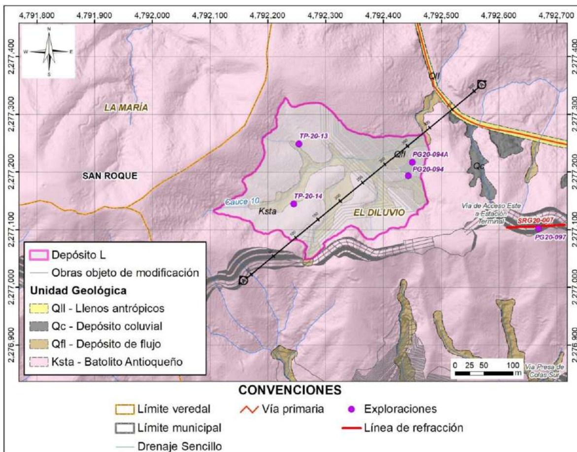
Figura 5.1.7.157 Localización en planta del depósito L con la sección de interés para el análisis geotécnico
