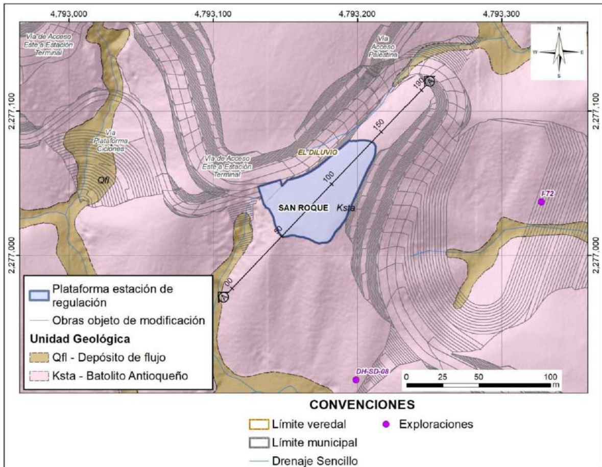
Figura 5.1.7.136 Localización en planta de la plataforma Estación de Regulación con la sección de interés para el análisis geotécnico
