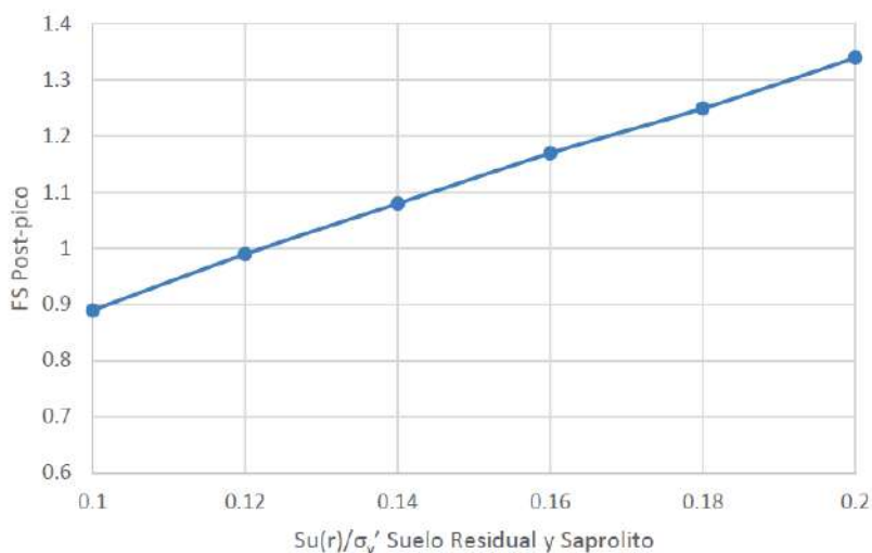
Figura 5.5.1.7.193 Análisis de sensibilidad post-pico – Depósito San Antonio
