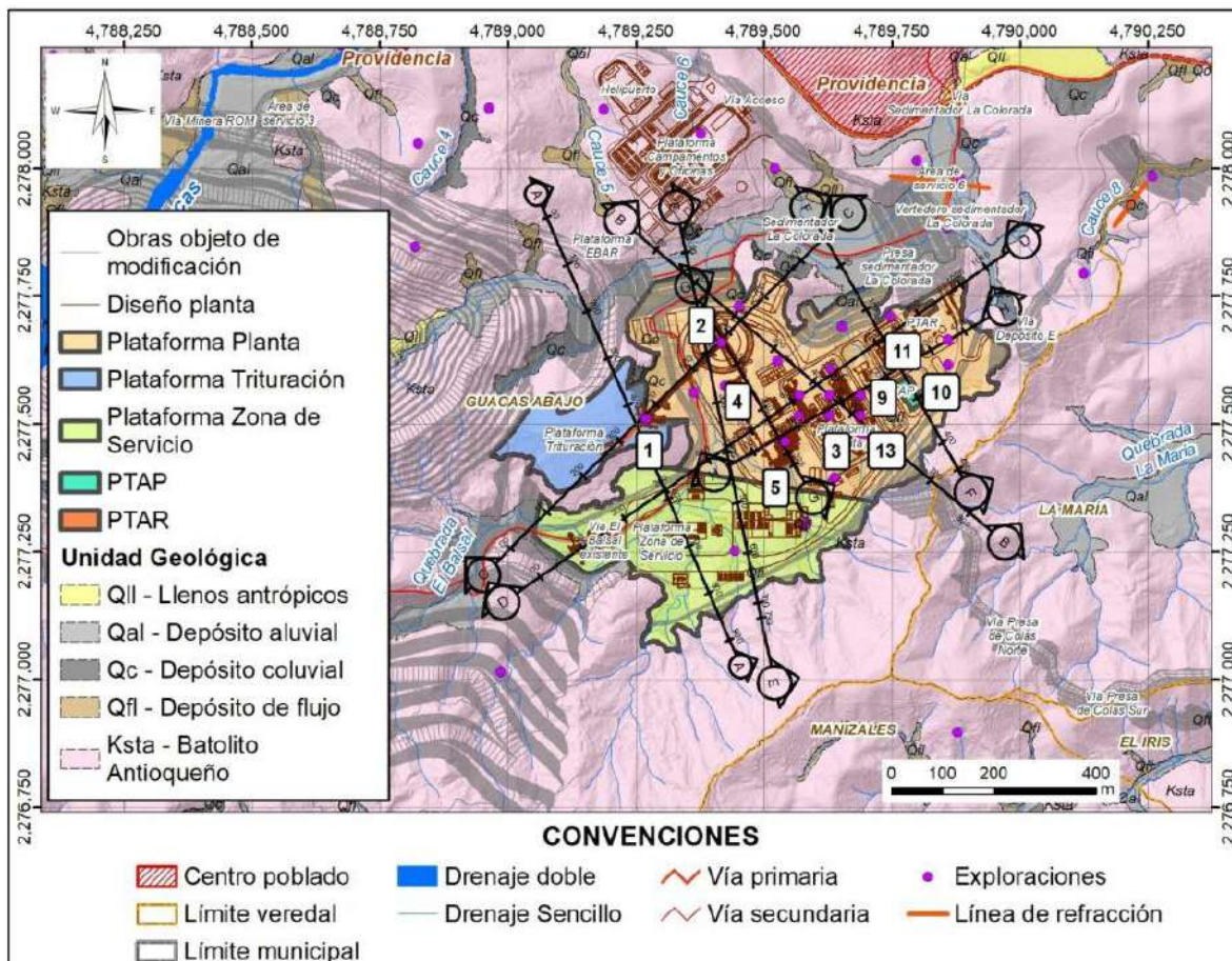
Figura 5.1.7.202 Ubicación de las obras en planta de la Plataforma Principal para los análisis de fundaciones
