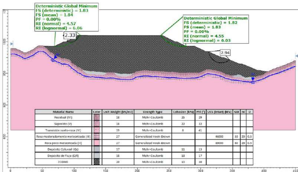
Figura 5.1.7.155 Análisis de estabilidad en condición estática con nivel freático normal de la Sección B – Depósito K
