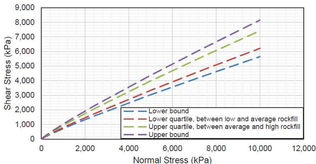
Figura 5.1.7.93 Funciones de resistencia al corte /normal del relleno de roca, tomado de Hawley & Cuning, 2017
