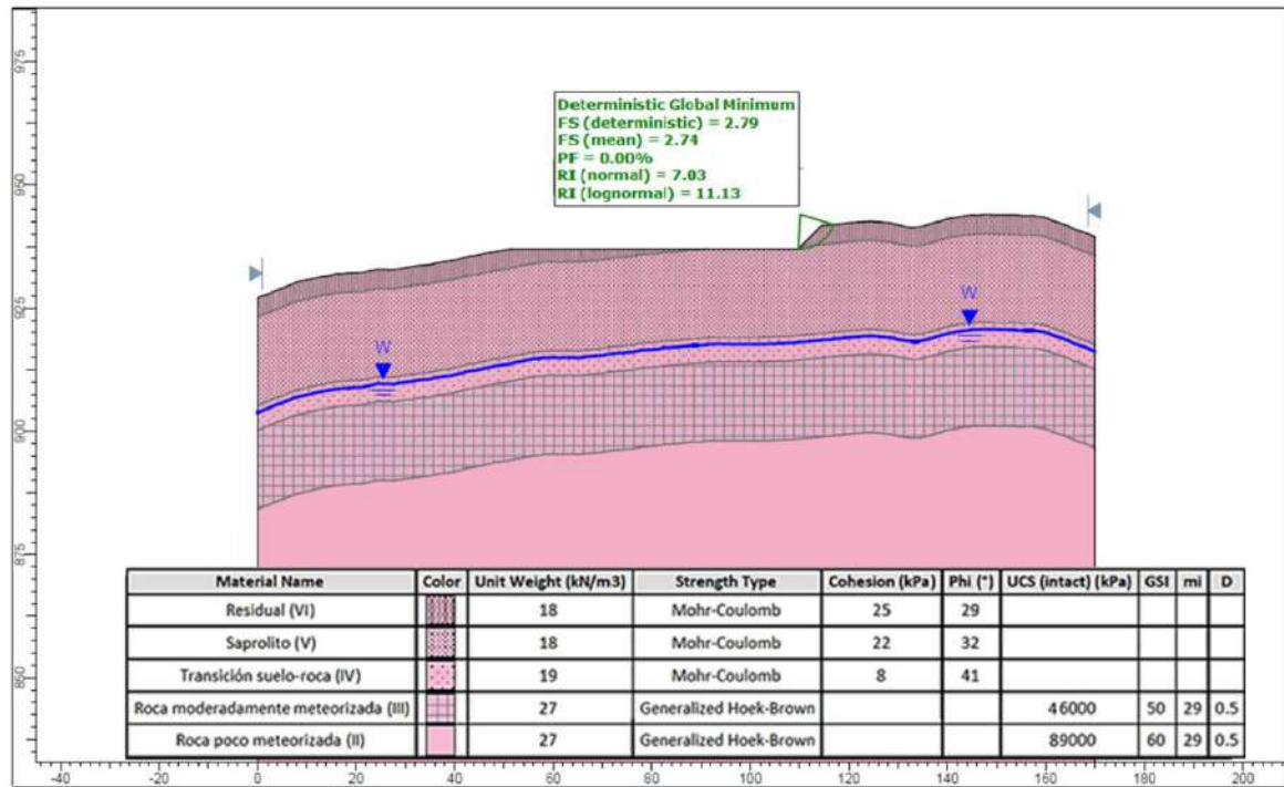
Figura 5.1.7.139 Análisis de estabilidad en condición estática con nivel freático normal de la plataforma de la Estación Terminal
