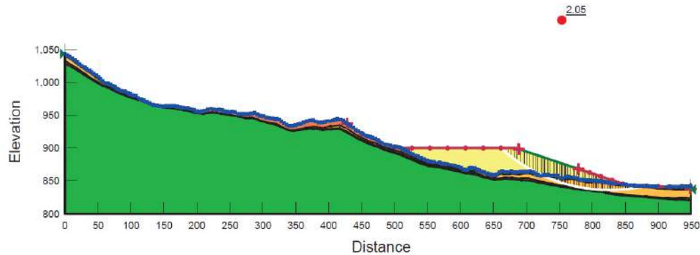
Figura 5.5.1.7.183 Análisis de estabilidad al cierre en condición estática de la Sección B – Depósito El Balsal, etapa de cierre
