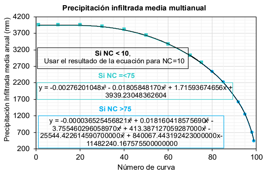
Figura 5.1.7.100 Curva de estimación de la precipitación infiltrada media multianual – Estación San Roque
