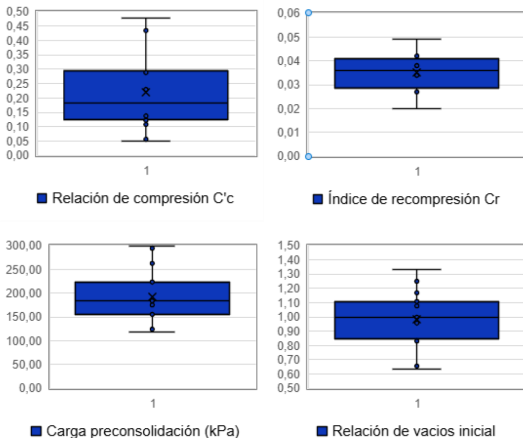
Figura 5.1.7.88 Horizonté V: Análisis de los resultados del análisis de consolidación. Número de datos 13 (Datos de C_r fueron reportados en 6 ensayos)
