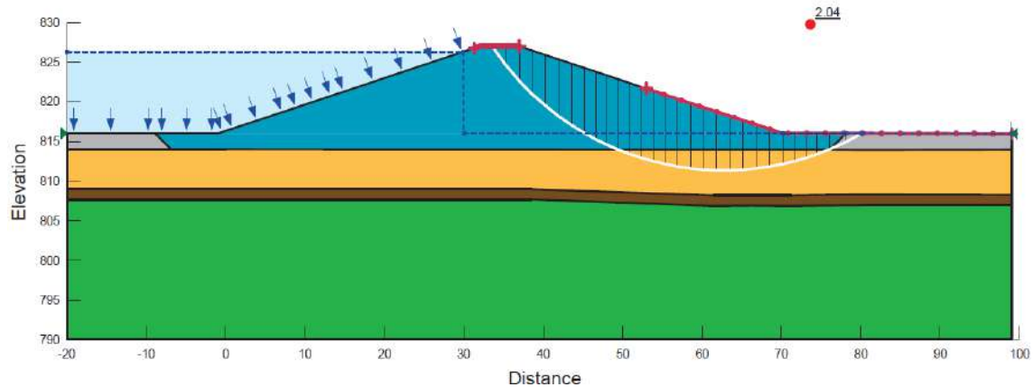
Figura 5.5.1.7.190 Análisis de estabilidad en condición estática de la Sección D – Presa Sedimentador San Antonio
