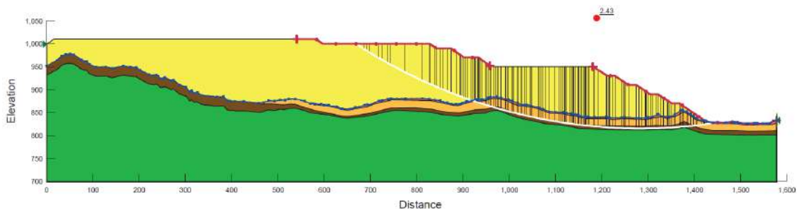
Figura 5.5.1.7.174 Análisis de estabilidad en condición estática de la Sección A – Depósito San Antonio, operación máxima
