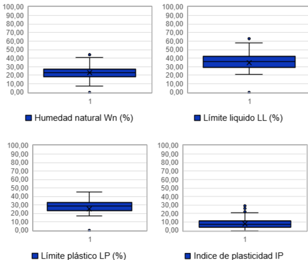
Figura 5.1.7.80 Horizonte V: Análisis de humedad natural y límites de la base de datos general. wn% (221 datos), LL (232 datos), LP (237 datos), IP (236 datos)
