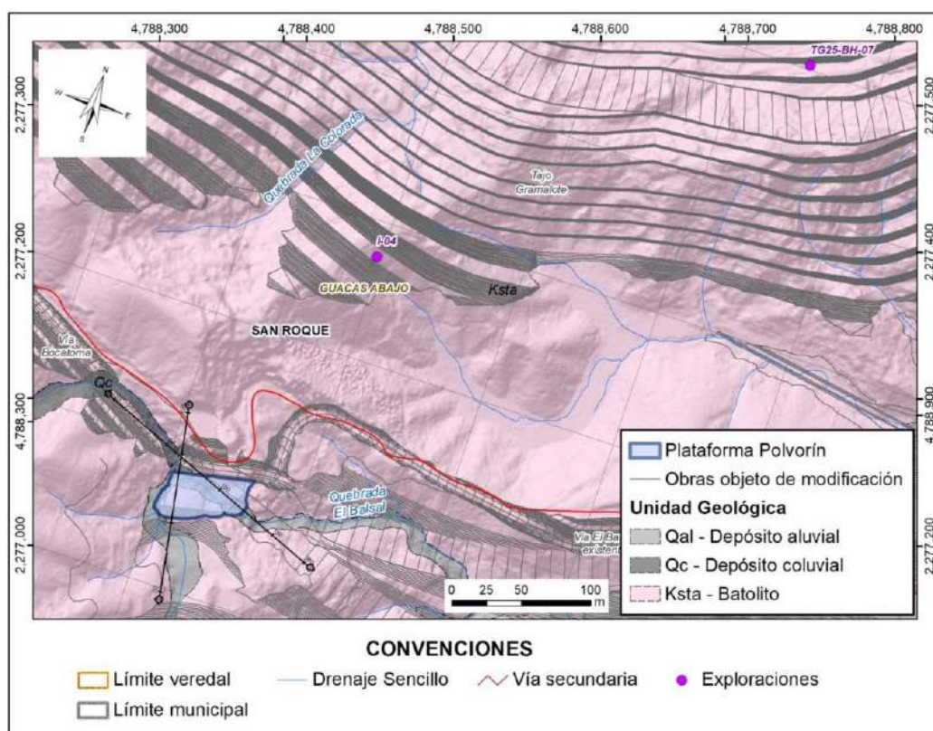
Figura 5.1.7.143 Localización en planta de la plataforma Polvorín con las secciones de interés para los análisis geotécnicos
