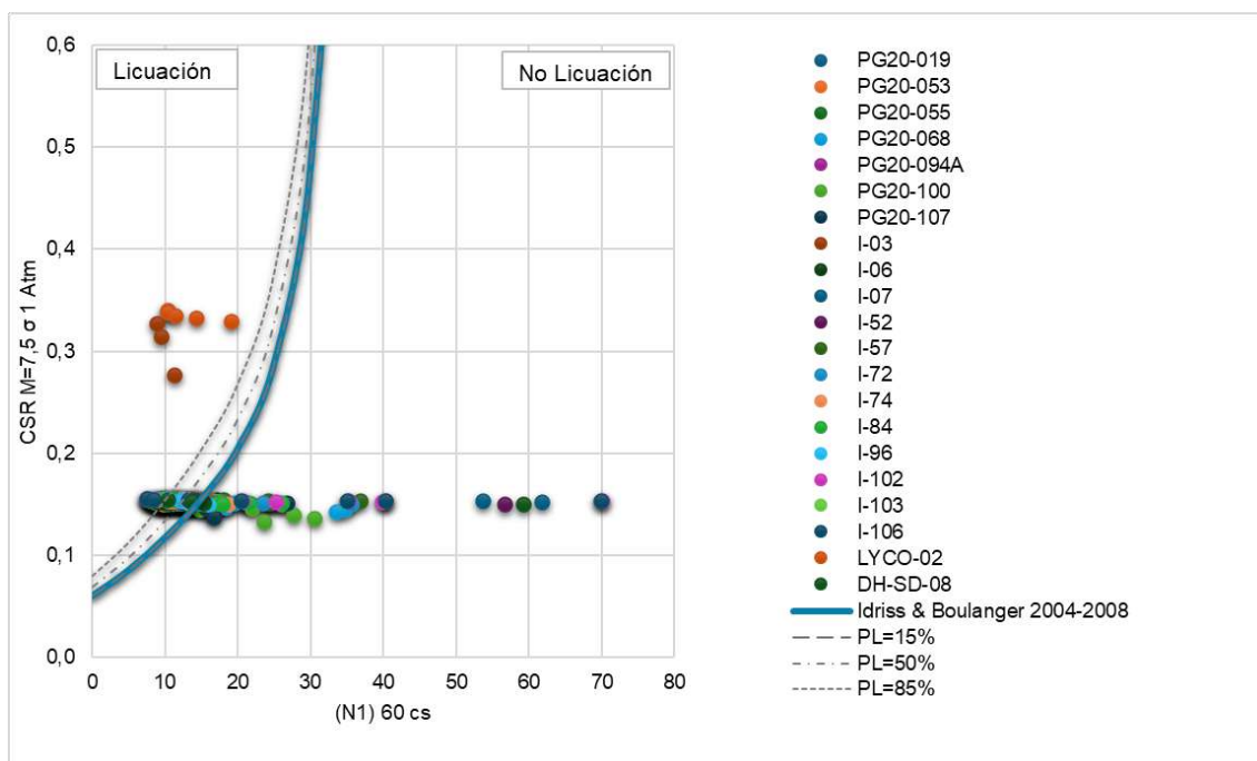
Figura 5.1.7.66 Análisis de licuación o licuefacción de muestras de suelo - Depósitos ZODME's. Método de Idriss y Boulanger (2010-2012) basado en el ensayo SPT
