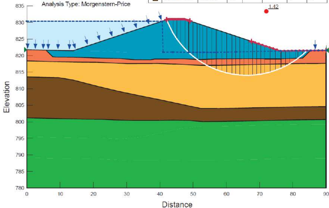
Figura 5.5.1.7.188 Análisis de estabilidad en condición post-pico de la Sección C – Presa del Sedimentador El Banco
