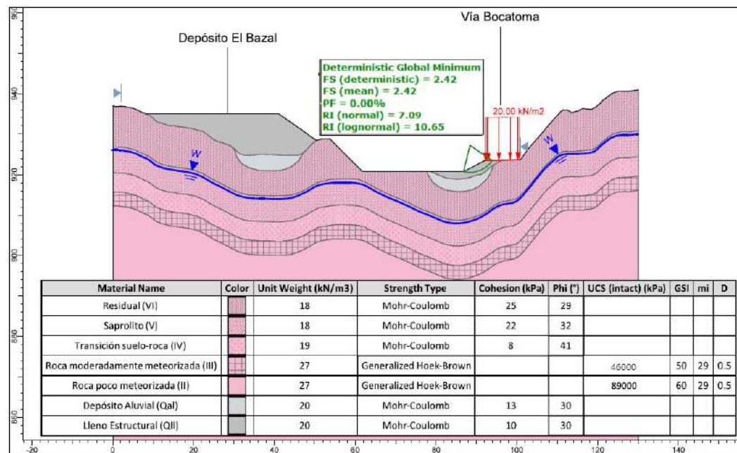
Figura 5.1.7.145 Análisis de estabilidad derecho en condición estática con nivel freático normal de la plataforma Polvorín
