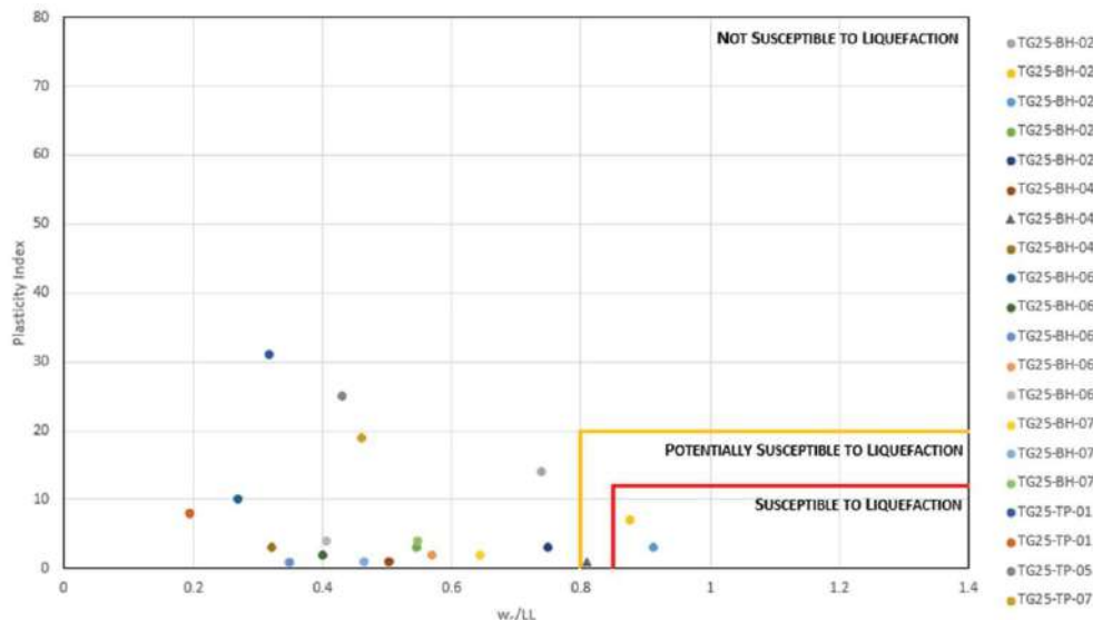
Figura 5.5.1.7.74 Análisis de licuación o licuefacción de muestras de saprolito – El Balsal. Método de Bray y Sancio (2006)
