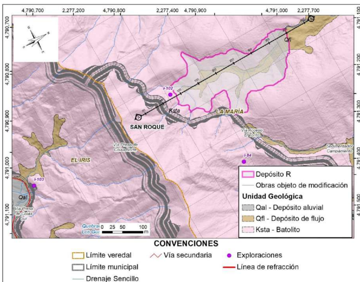
Figura 5.1.7.164 Localización en planta del depósito R con la sección de interés para el análisis geotécnico
