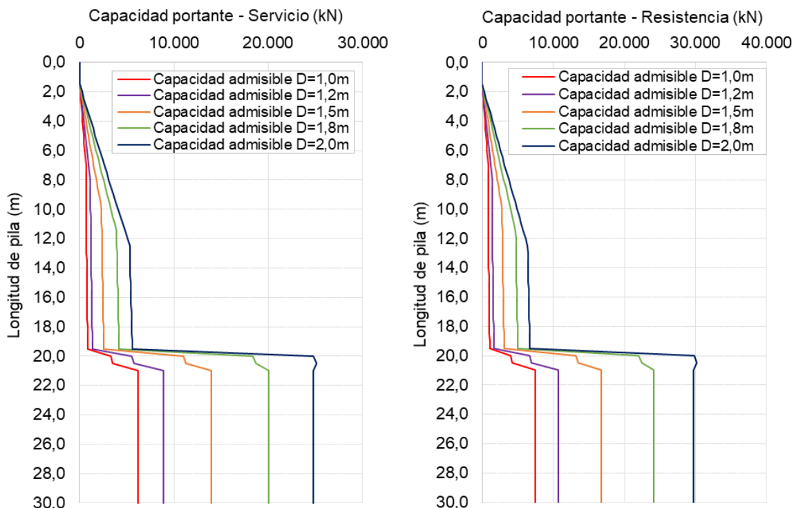
Figura 5.1.7.205 Capacidad de carga a compresión de una pila en estado de servicio y resistencia – CIP Tanks
