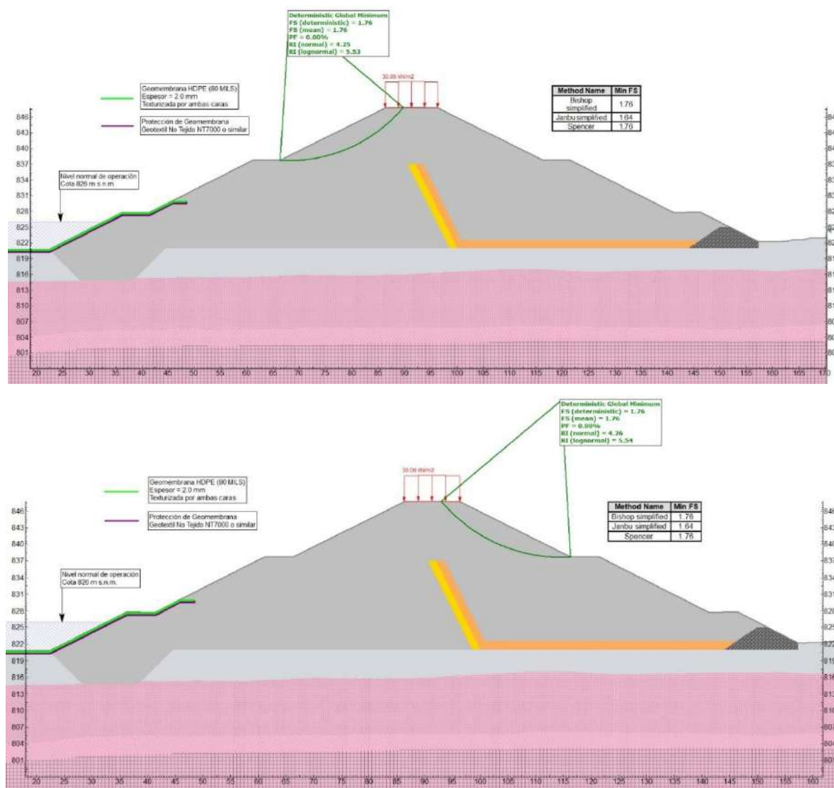
Figura 5.1.7.107 Condición largo plazo. Espaldón aguas arriba y aguas abajo de la presa del sedimentador La Colorada. Análisis estático con el nivel normal de operación del embalse. Sección B – km 0+820
