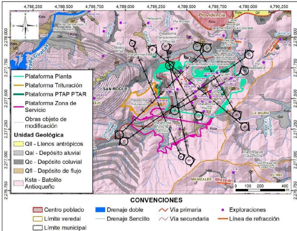
Figura 5.1.7.120 Localización en planta de la Plataforma Principal con las secciones de interés para los análisis geotécnicos
