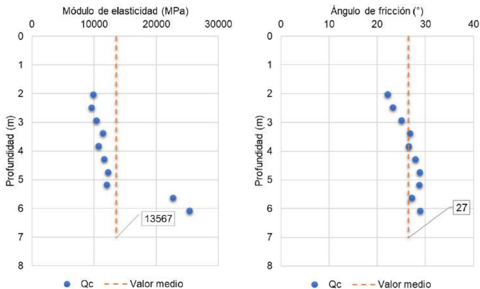
Figura 5.1.7.23 Depósito Coluvial (Qc): Análisis de las correlaciones entre el SPT y el módulo de elasticidad (izquierda); el SPT y el ángulo de fricción (derecha)
