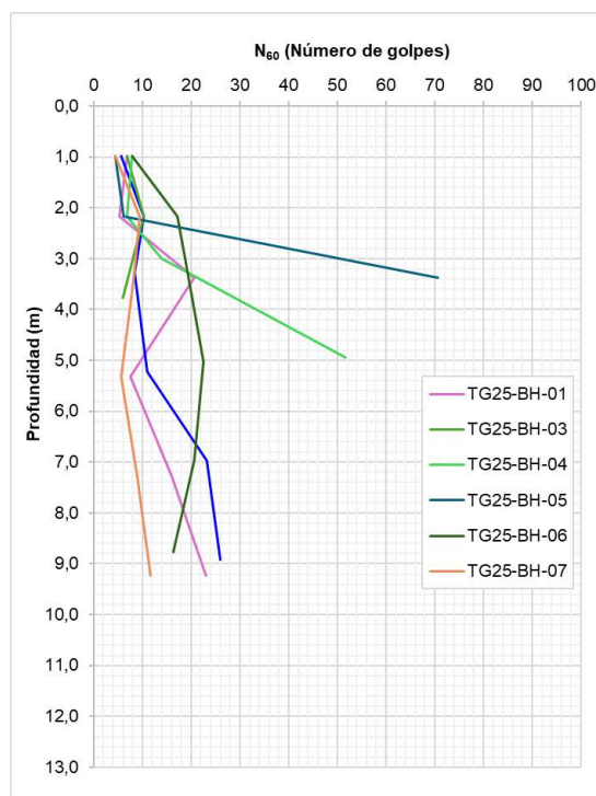
Figura 5.1.7.67 Análisis para las pruebas in situ SPT realizadas para El Balsal.
