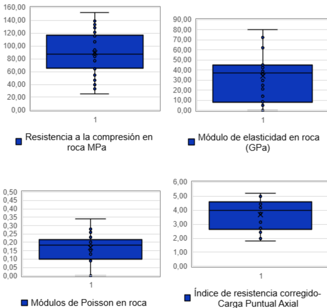
Figura 5.1.7.90 Horizonte II: Análisis de la compresión simple (datos 28), módulo de elasticidad (datos 28), relación de Poisson (datos 20), Índice de resistencia Carga Puntual Is 50 en MPa en la base de datos general (datos axiales 12 y datos diametrales 5)
