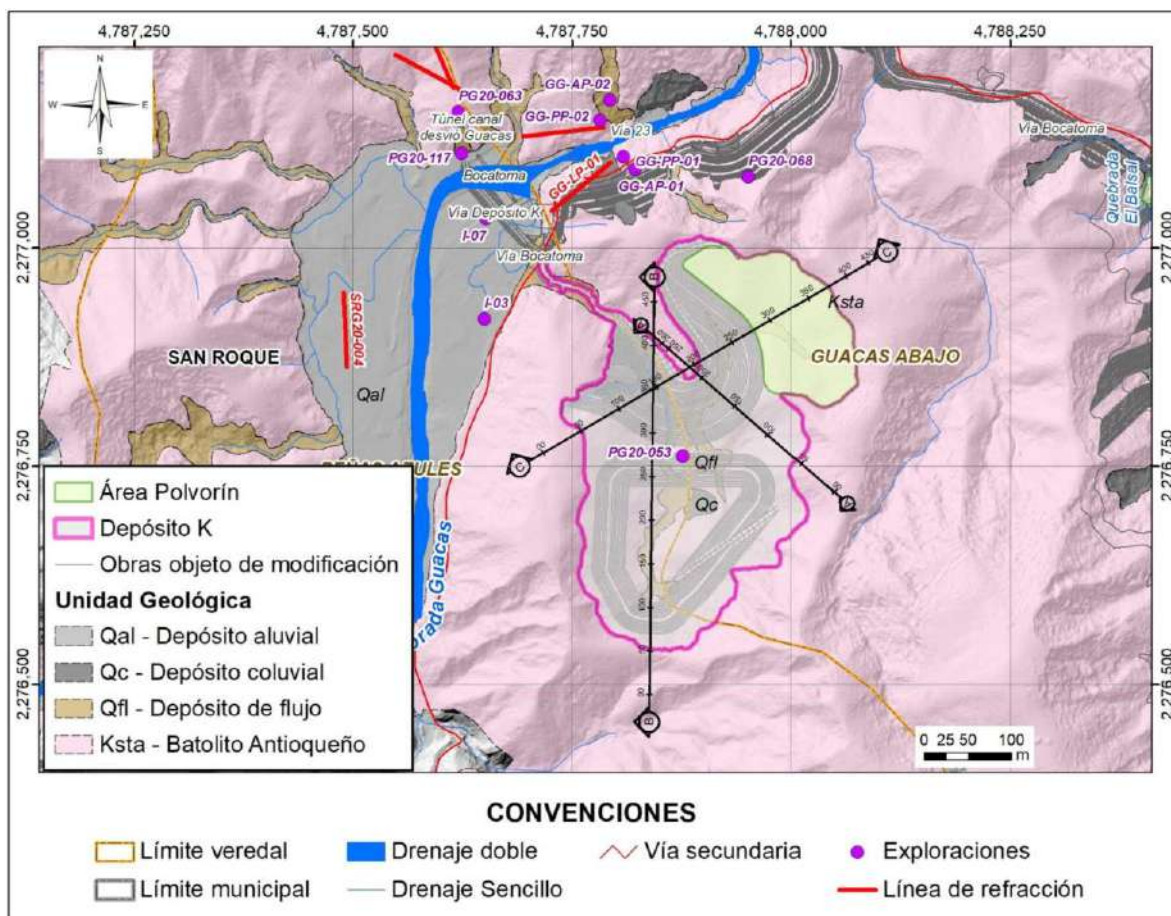
Figura 5.1.7.153 Localización en planta de la depósito K con las secciones de interés para los análisis geotécnicos
