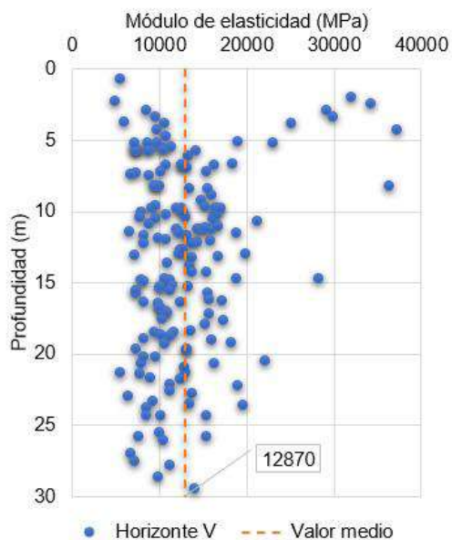
Figura 5.1.7.42 Horizonte V: Análisis de las correlaciones entre el SPT y el módulo de elasticidad
