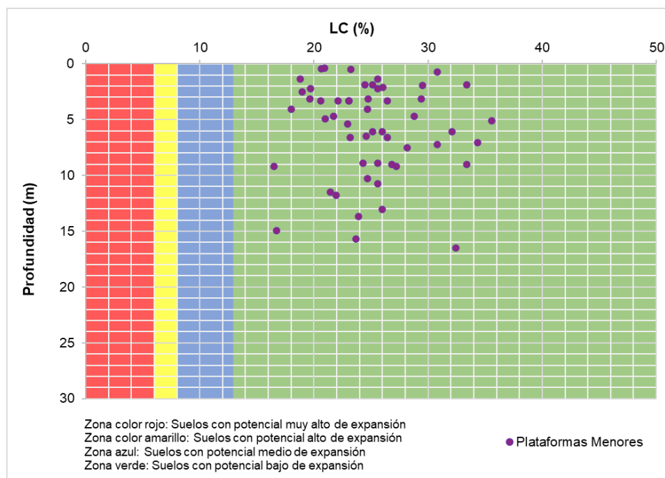
Figura 5.1.7.54 Resultados límites de contracción en las plataformas menores
