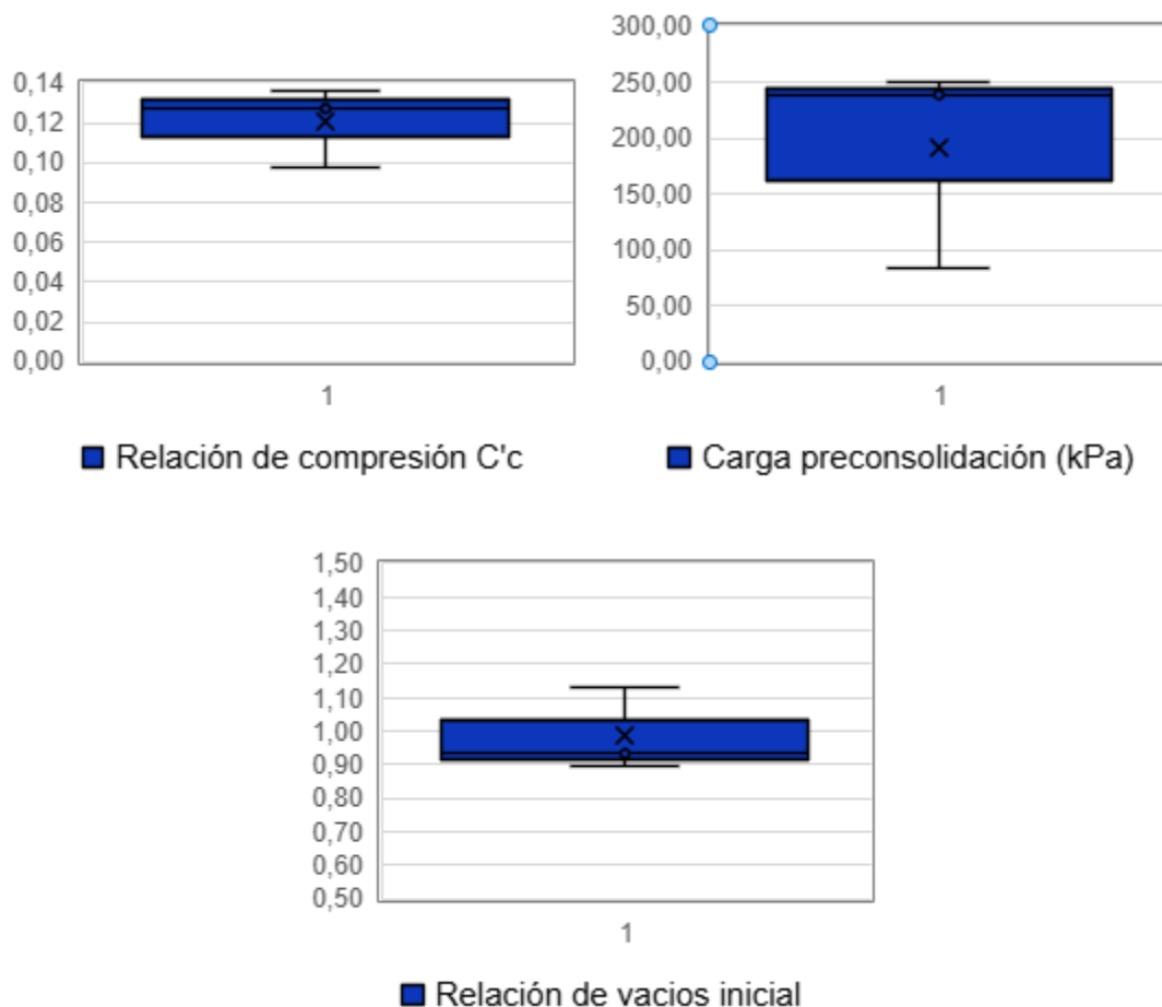
Figura 5.1.7.87 Horizonte VI: Análisis de los resultados del análisis de consolidación. Número de datos 3
