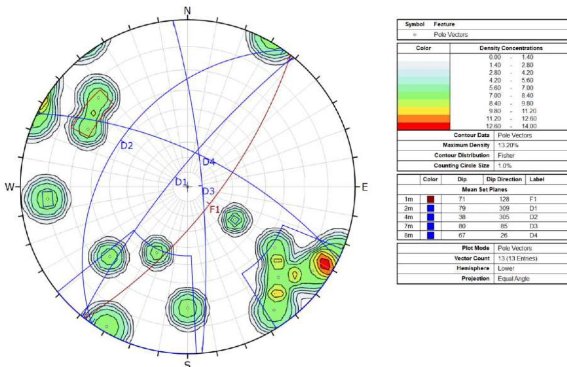
Figura 5.1.7.96 Estereograma de familias de discontinuidades
