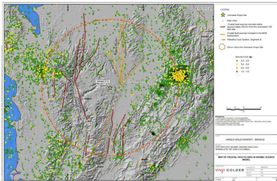
Figura 5.1.7.16 Fallas activas mapeadas en un radio de 200 km desde el punto central de análisis localizado en la mina Gramalote
