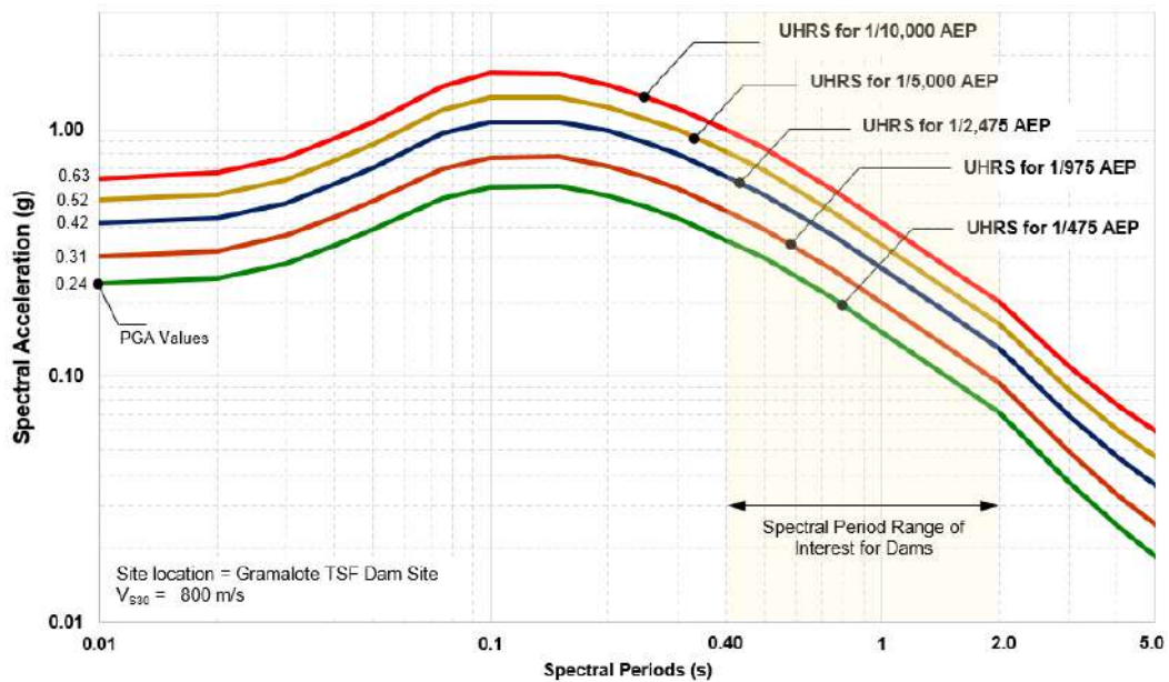
Figura 5.1.7.19 Espectros de Respuesta de Amenaza Uniforme (UHRs) (5% de amortiguamiento) en el sitio de la mina Gramalote. El valor de Vs30 usado es de 800 m/s
