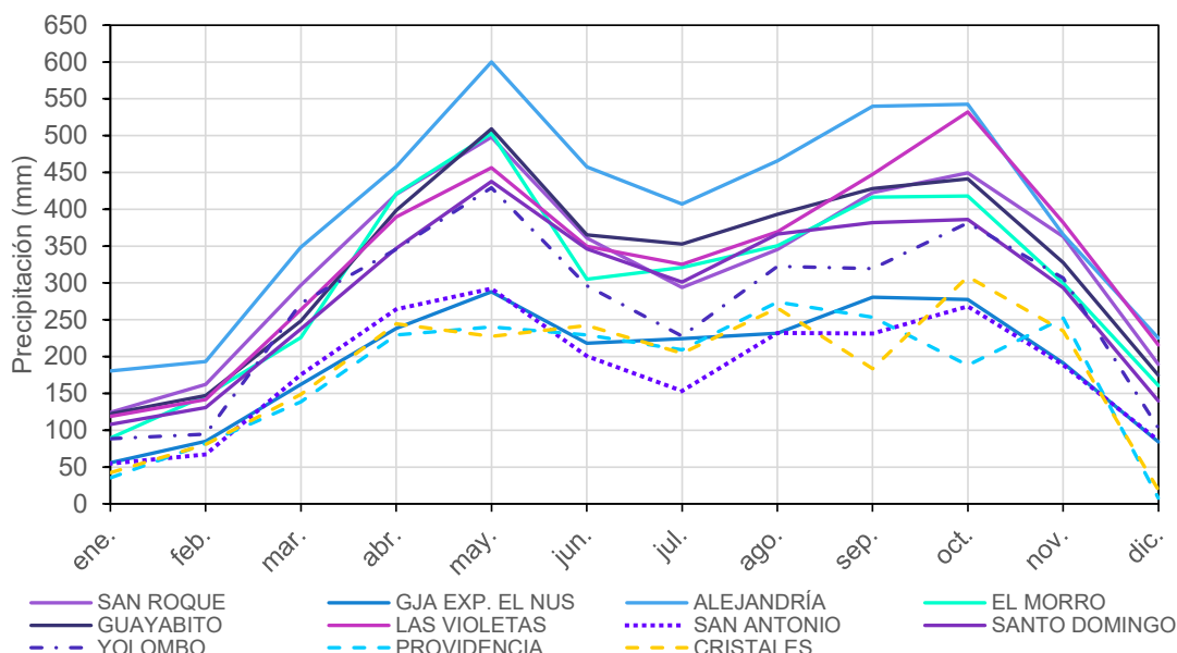
Figura 5.1.7.98 Ciclos característicos de la precipitación para cada una de las estaciones.
