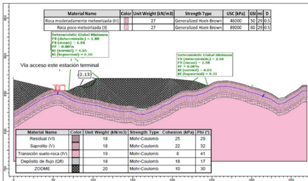
Figura 5.1.7.163 Análisis de estabilidad en condición estática con nivel freático normal de la Sección B – Depósito O
