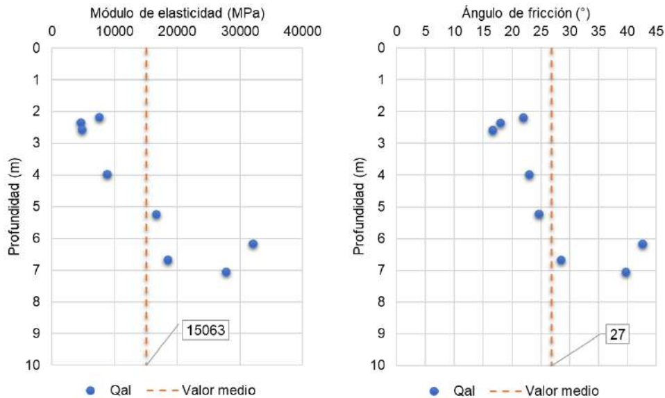
Figura 5.1.7.22 Depósito Aluvial (Qal): Análisis de las correlaciones entre el SPT y el módulo de elasticidad (izquierda); el SPT y el ángulo de fricción (derecha)
