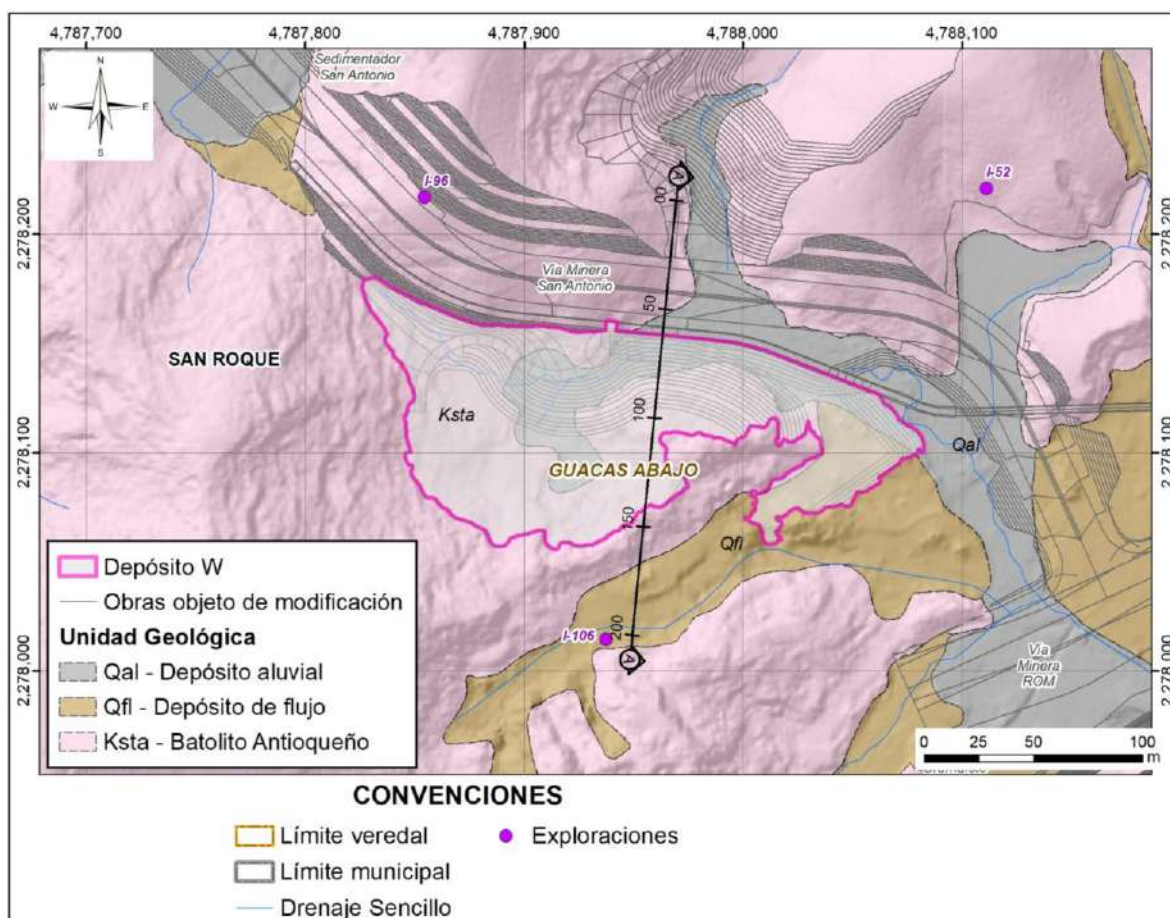
Figura 5.1.7.166 Localización en planta del depósito W con la sección de interés para el análisis geotécnico
