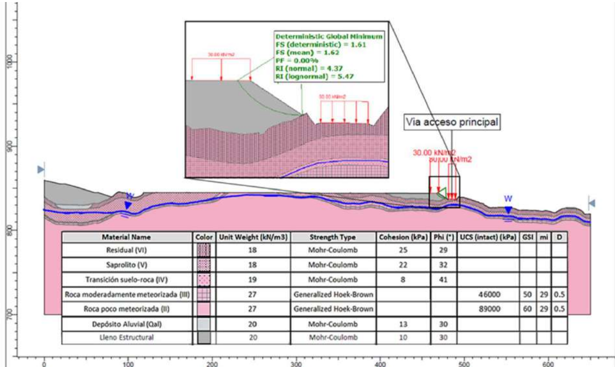
Figura 5.1.7.130 Análisis de estabilidad en condición estática con nivel freático normal de la plataforma de campamentos y oficinas
