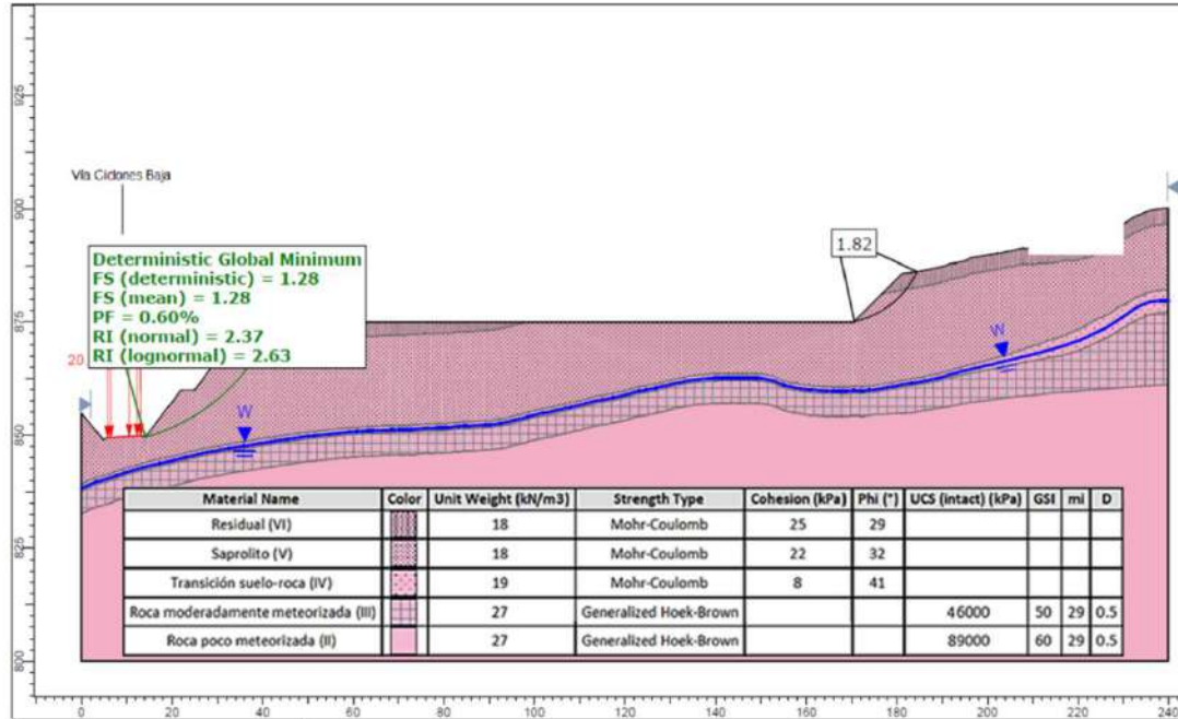
Figura 5.1.7.132 Análisis de estabilidad en condición estática con nivel freático normal de la plataforma Ciclones
