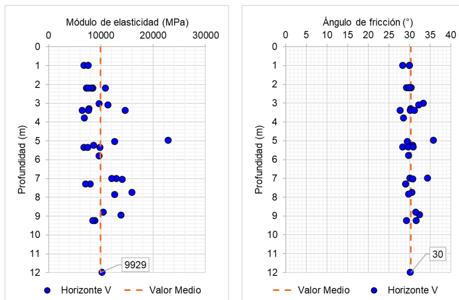
Figura 5.1.7.70 Horizonte V: Análisis de las correlaciones entre el SPT y el módulo de elasticidad (izquierda); SPT y el ángulo de fricción (derecha)
