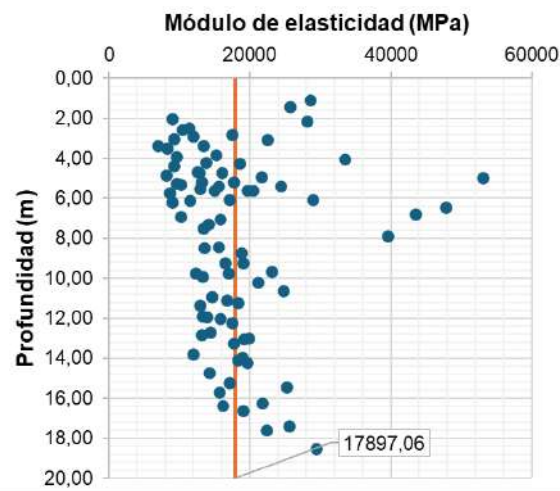
Figura 5.1.7.51 Horizonte V: Análisis de las correlaciones entre el SPT y el módulo de elasticidad
