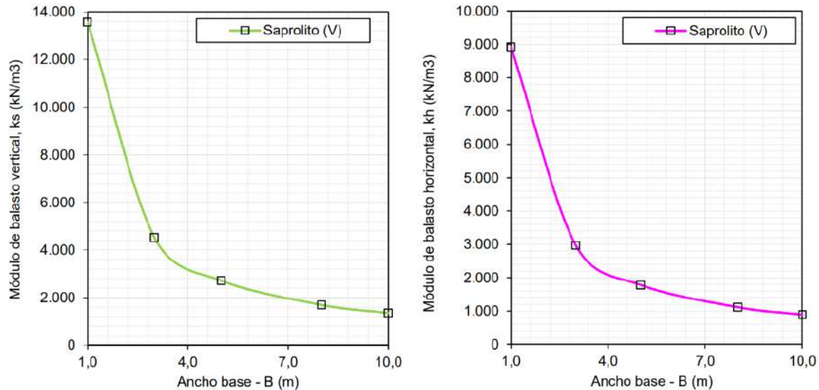
Figura 5.1.7.204 Ábaco de módulo de balasto para cimentaciones superficiales – CIP Tanks
