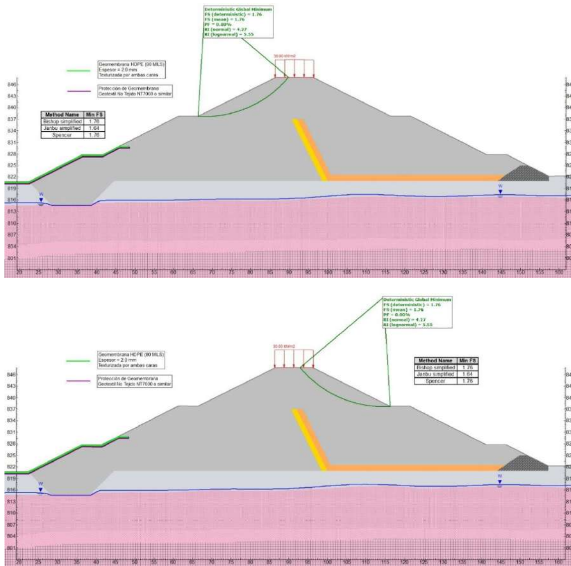
Figura 5.1.7.106 Condición fin de construcción. Espaldón aguas arriba y aguas abajo de la presa del sedimentador La Colorada. Análisis estático. Sección B – km 0+820
