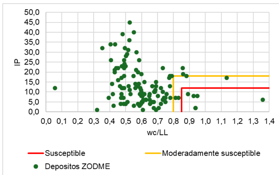
Figura 5.1.7.65 Análisis de licuación o licuefacción de muestras de suelo – Depósitos ZODME's. Método de Bray y Sancio (2006)
