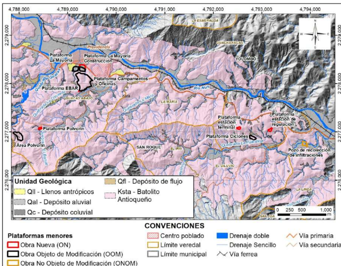
Figura 5.1.7.48 Localización en planta de las plataformas menores del proyecto Gramalote
