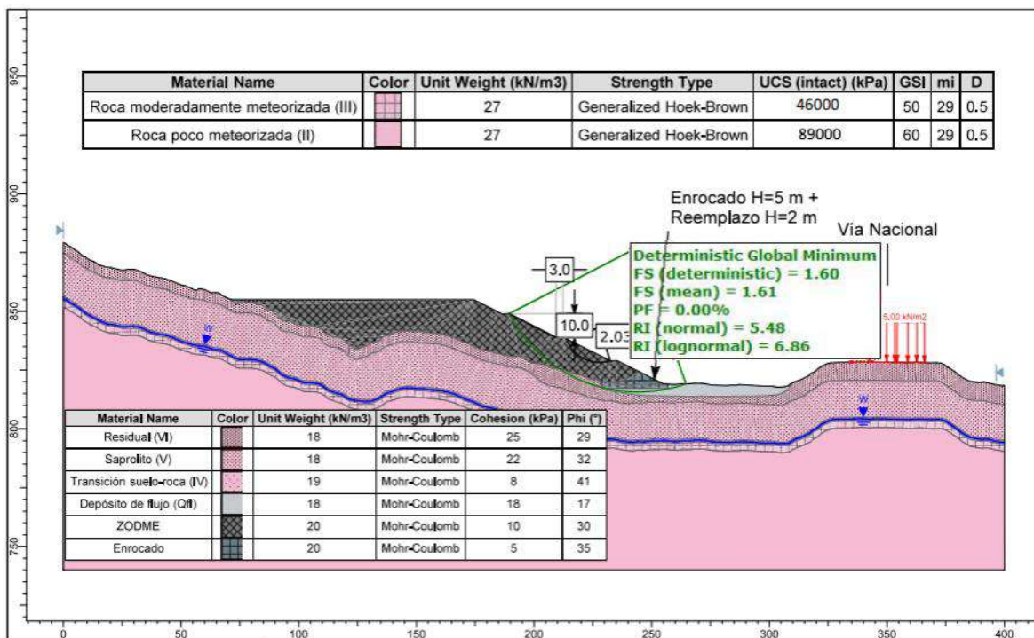
Figura 5.1.7.171 Análisis de estabilidad en condición estática con nivel freático normal de la Sección A – Depósito El Torito
