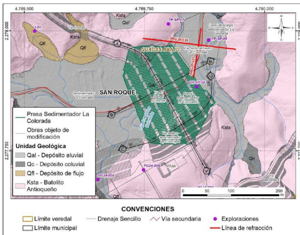
Figura 5.1.7.103 Localización en planta de las secciones de interés para el análisis geotécnico – Presa del sedimentador La Colorada
