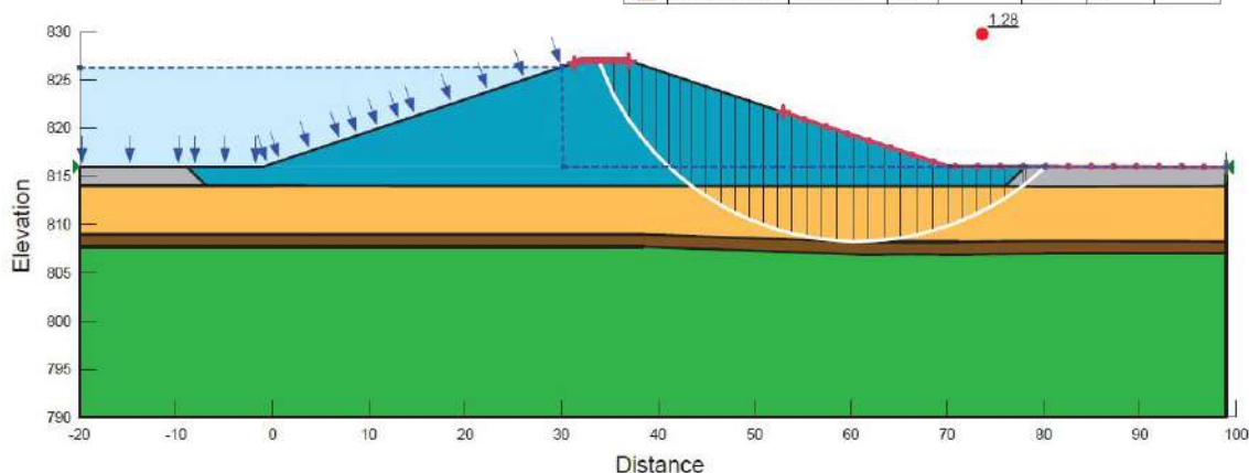
Figura 5.5.1.7.192 Análisis de estabilidad en condición post-pico de la Sección D – Presa Sedimentador San Antonio
