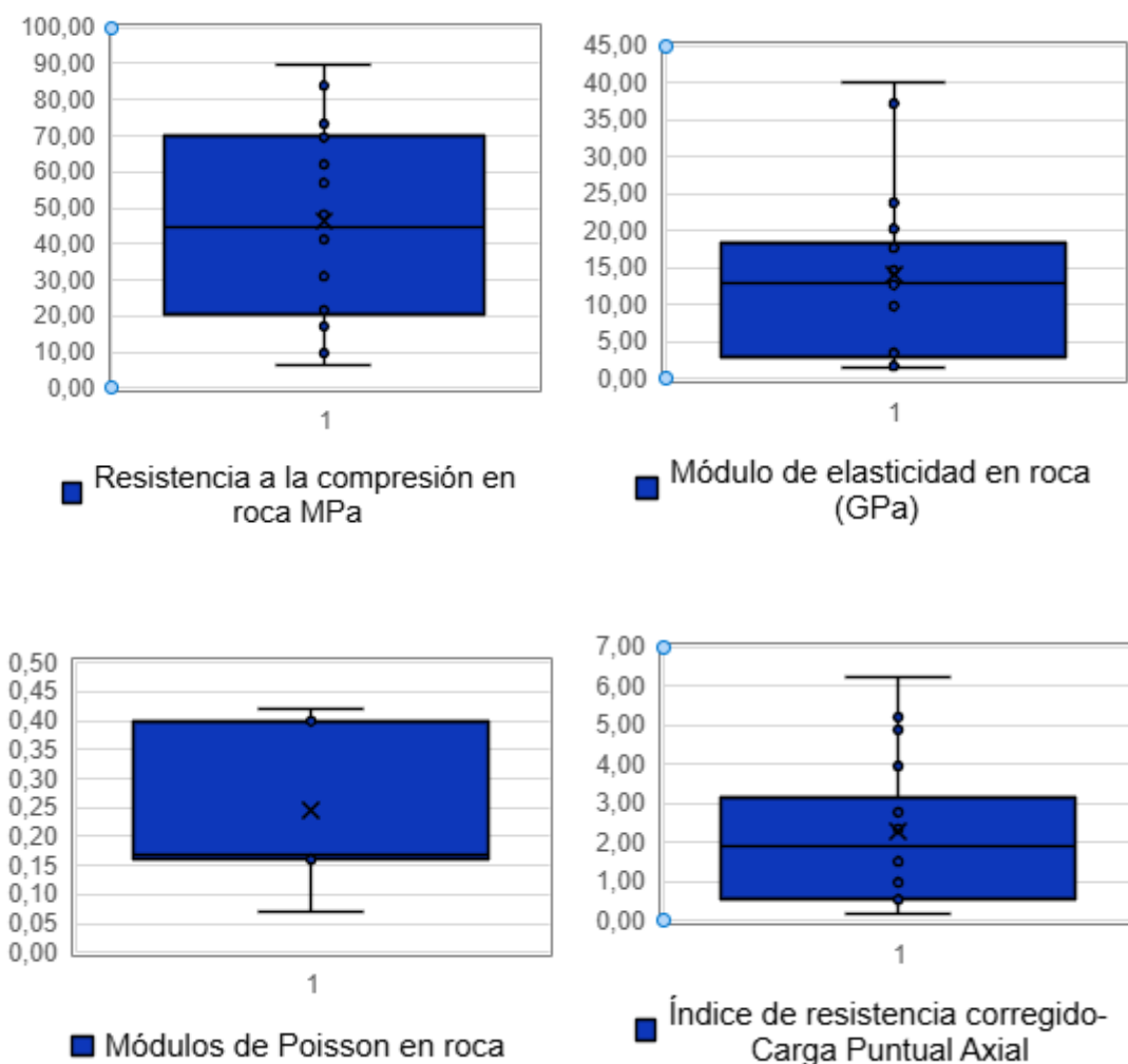
Figura 5.1.7.89 Horizonte III: Análisis de la compresión simple (datos 16), módulo de elasticidad (datos 16), relación de Poisson (datos 6), Índice de resistencia Carga Puntual I_{s(50)} en MPa en la base de datos general (datos 16 axial y 11 diametral)
