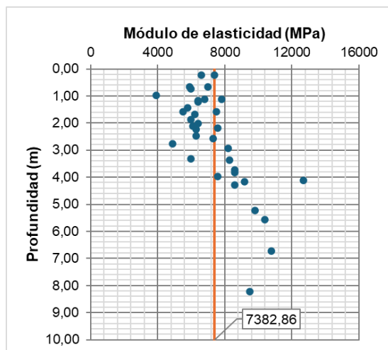
Figura 5.1.7.50 Horizonte VI: Análisis de las correlaciones entre el SPT y el módulo de elasticidad
