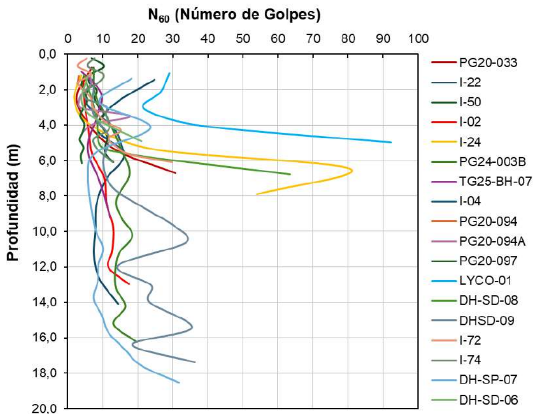
Figura 5.1.7.49 Análisis para las pruebas in situ SPT realizadas para los 18 sondajes en la zona de las plataformas menores
