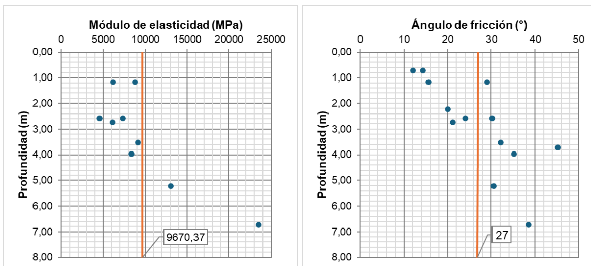
Figura 5.1.7.52 Depósito aluvial: Análisis de las correlaciones entre el SPT y el módulo de elasticidad (izquierda); el SPT y el ángulo de fricción (derecha)
