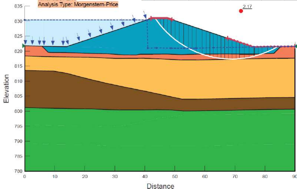
Figura 5.5.1.7.186 Análisis de estabilidad en condición estática de la Sección C – Presa del Sedimentador El Banco
