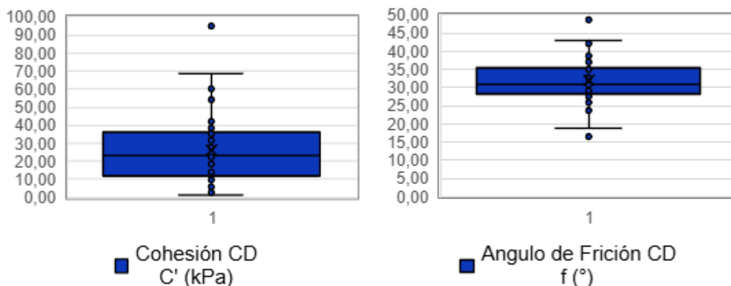
Figura 5.1.7.86 Horizonte V: Análisis del ángulo de fricción y cohesión en la base de datos general. Número de datos 35
