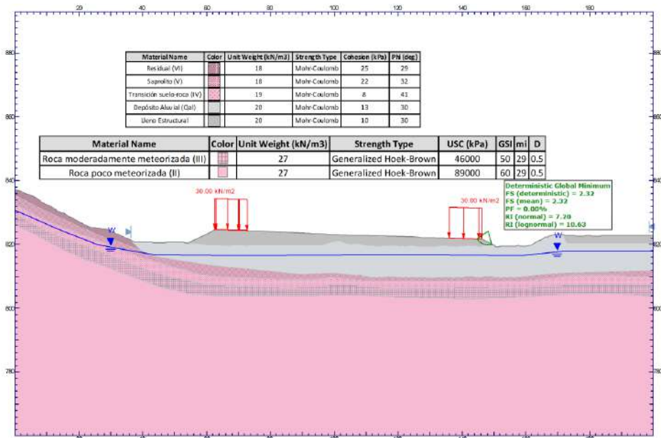
Figura 5.1.7.142 Análisis de estabilidad derecho en condición estática con nivel freático normal de la plataforma La Mayoría – Sección C
