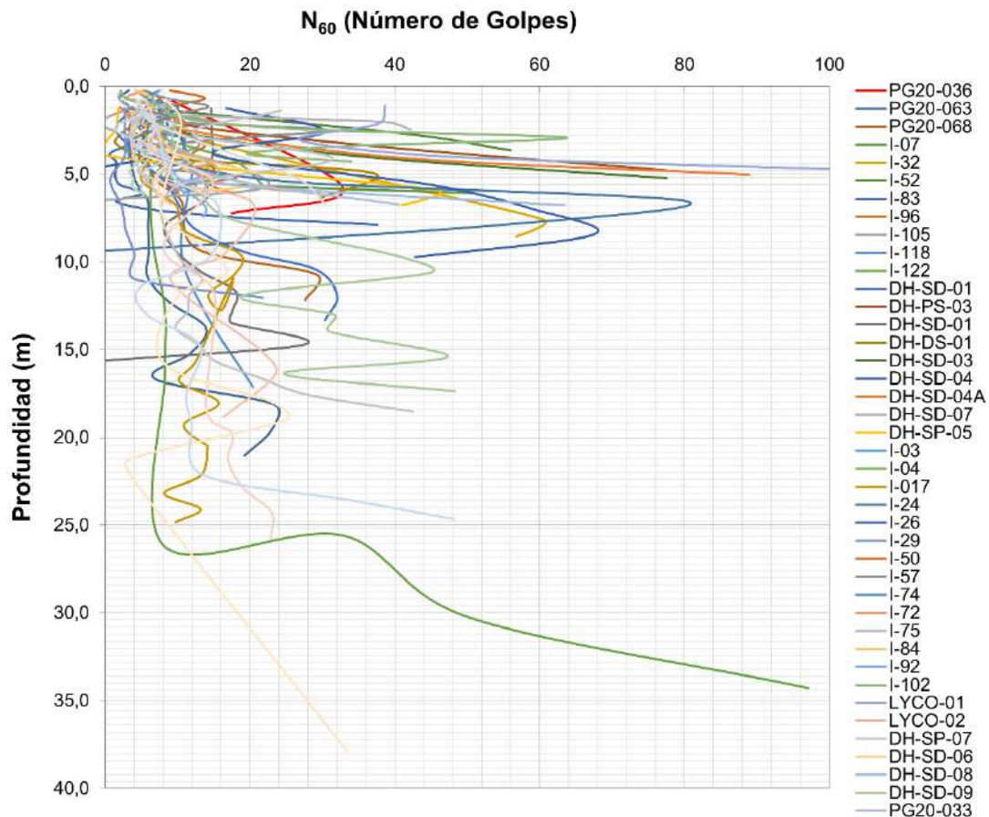
Figura 5.1.7.31 Análisis para las pruebas in situ SPT realizadas para los sondajes en la zona de influencia e intervención del sistema vial
