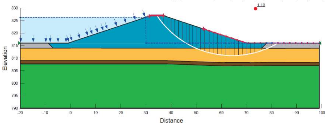
Figura 5.5.1.7.191 Análisis de estabilidad en condición pseudoestática de la Sección D – Presa Sedimentador San Antonio
