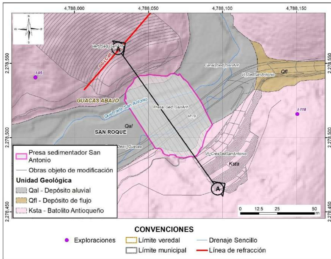
Figura 5.1.7.189 Localización en planta de las secciones de interés para el análisis geotécnico – Presa del sedimentador San Antonio
