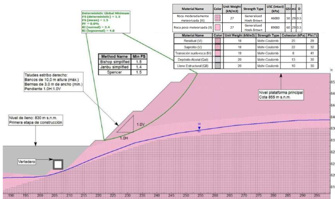
Figura 5.1.7.112 Análisis de estabilidad en condición estática con nivel freático normal. Estribo derecho presa del sedimentador La Colorada (Etapa 2 – Excavación permanente)
