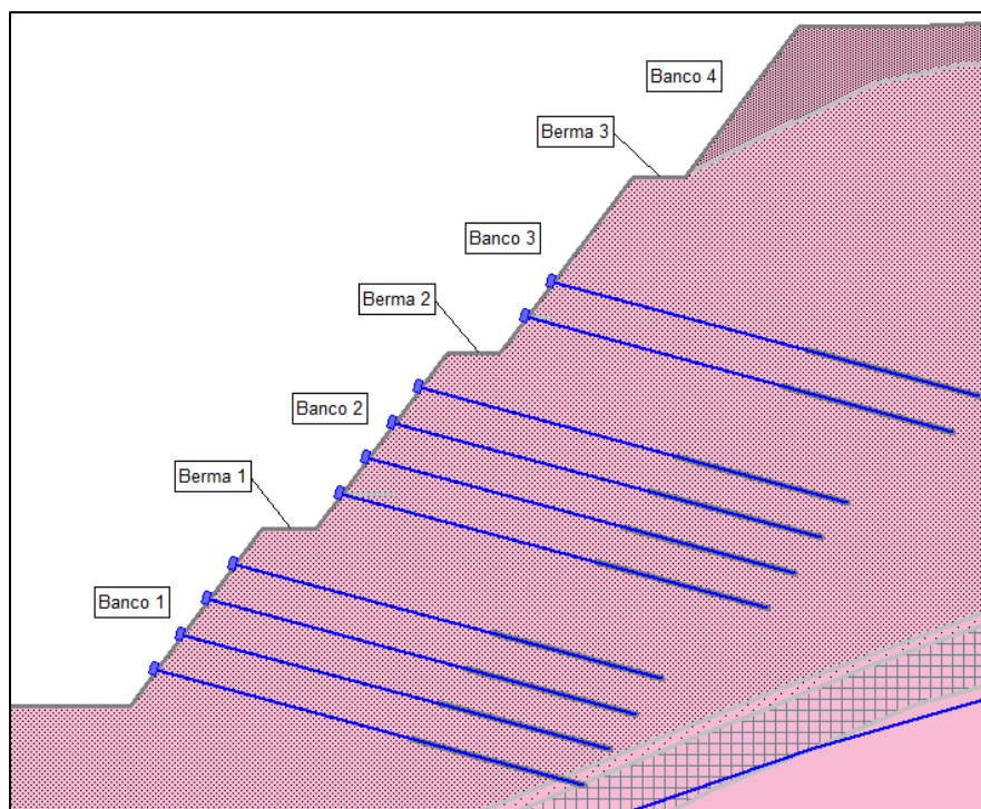
Figura 5.1.7.95 Enumeración de bancos y bermas de los taludes de corte (banco 1 es el más cercano a la rasante de la vía)
