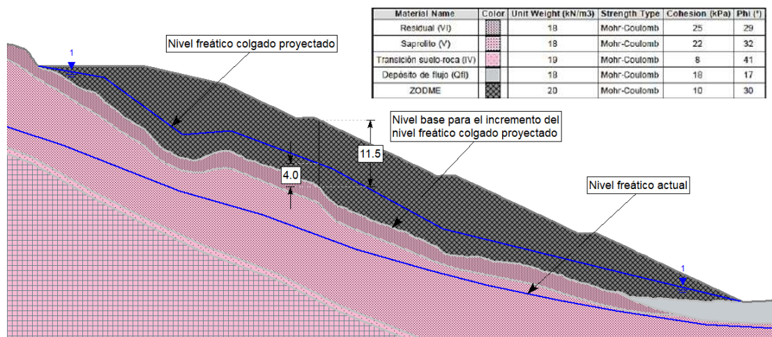
Figura 5.1.7.146 Ejemplo referencia considerada en medición de la profundidad del nivel freático promedio para el cálculo del incremento en el escenario extremo ( Tr=20 años) en el depósito
