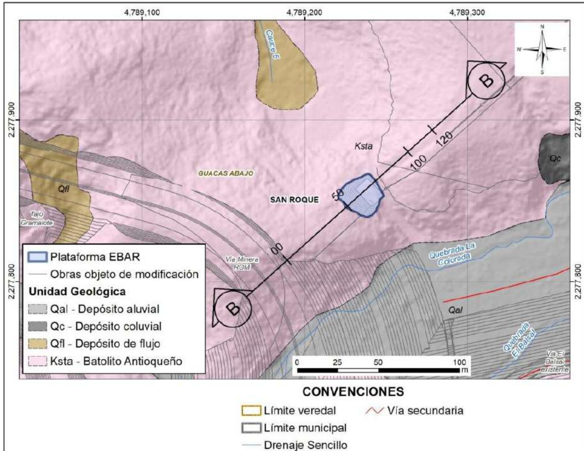
Figura 5.1.7.133 Localización en planta de la plataforma EBAR con la sección de interés para el análisis geotécnico
