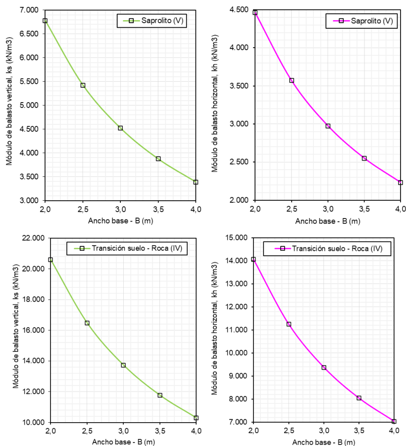
Figura 5.1.7.201 Módulo de balasto vertical y horizontal – Horizonte V (superior) y IV (inferior)
