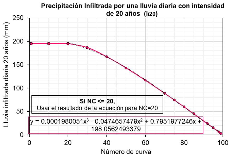
Figura 5.1.7.101 Curva de estimación de la precipitación infiltrada por una lluvia diaria con intensidad de 20 años – Estación San Roque
