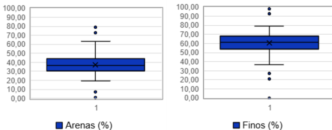
Figura 5.1.7.78 Horizonte VI: Análisis de humedad natural y límites de la base de datos general. Número de datos 78
