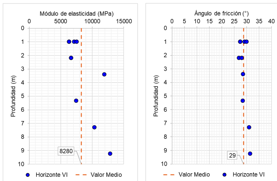
Figura 5.1.7.69 Horizonte VI: Análisis de las correlaciones entre el SPT y el módulo de elasticidad (izquierda); SPT y el ángulo de fricción (derecha)
