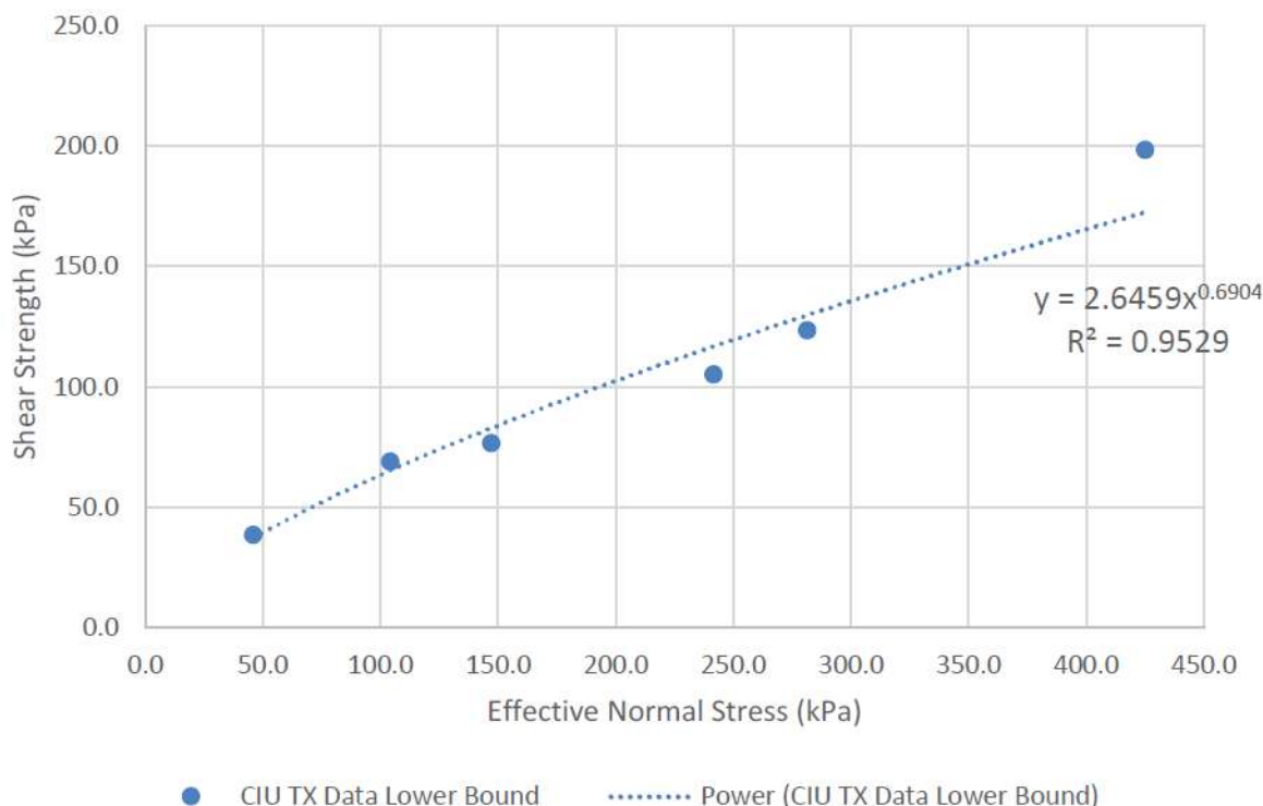
Figura 5.1.7.94 Funciones de resistencia al corte /normal del relleno de roca, para las presas de Sedimentadores El Banco y San Antonio
