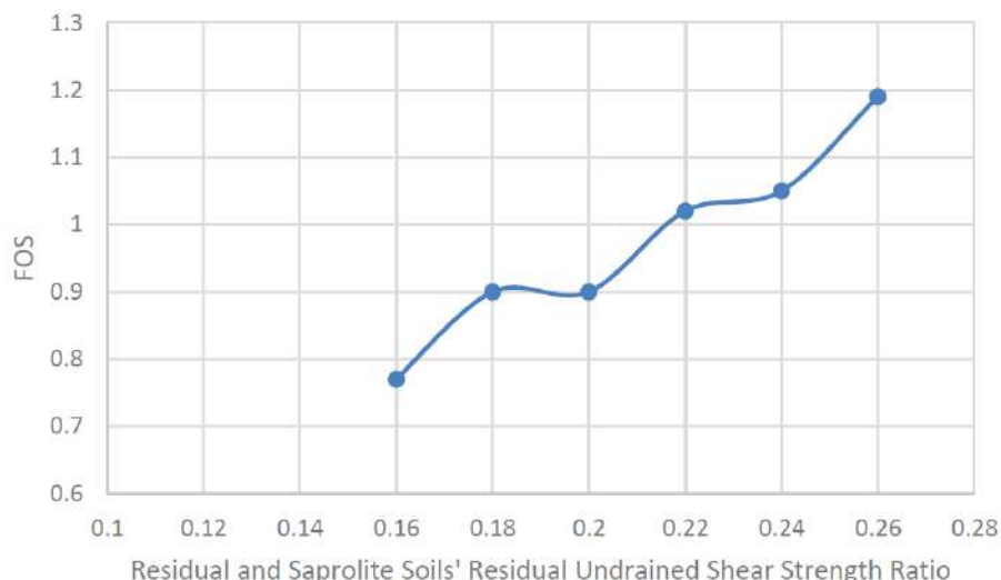
Figura 5.5.1.7.198 Análisis de sensibilidad post-pico al cierre– Depósito El Balsal
