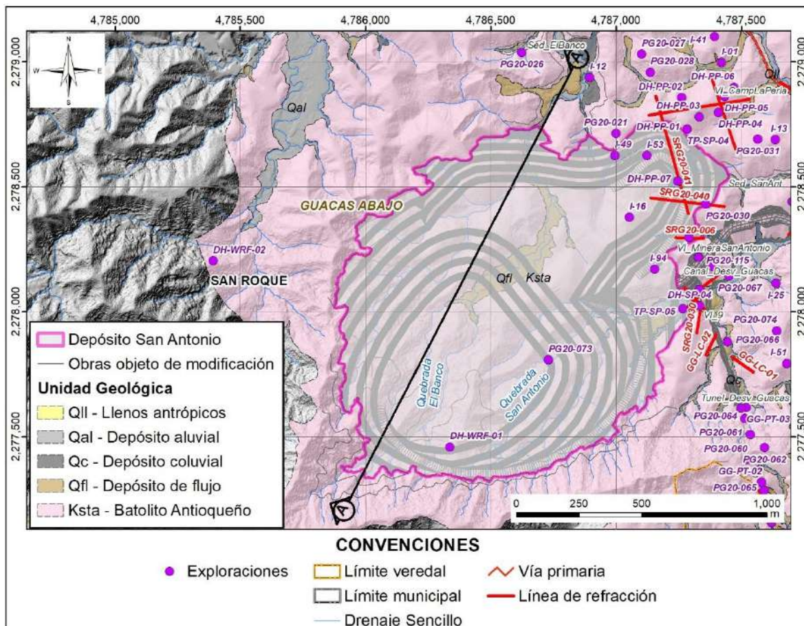
Figura 5.5.1.7.173 Localización en planta de la sección de interés para el análisis geotécnico – Depósito San Antonio
