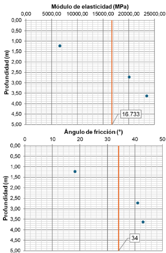
Figura 5.1.7.60 Depósito Aluvial: Análisis de las correlaciones entre el SPT y el módulo de elasticidad (izquierda); el SPT y el ángulo de fricción (derecha)
