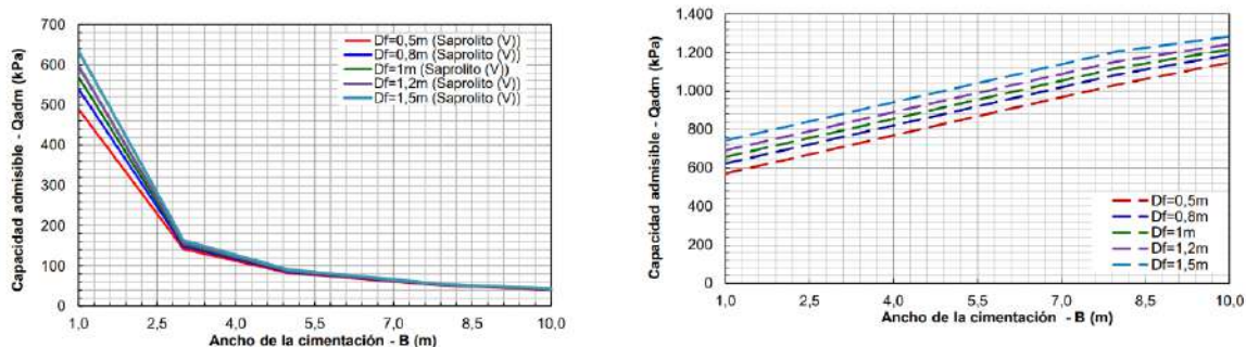
Figura 5.1.7.203 Ábaco capacidad de soporte admisible para cimentaciones superficiales en condiciones de servicio – CIP Tanks (izquierda: capacidad admisible por control de asentamientos, derecha: capacidad admisible por cortante)
