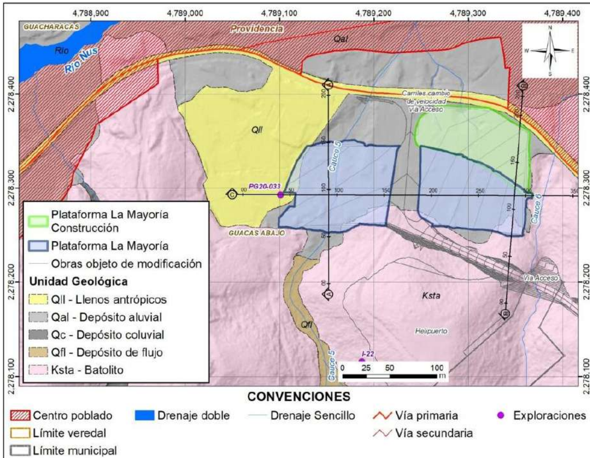
Figura 5.1.7.140 Localización en planta de la plataforma La Mayoría con las secciones de interés para los análisis geotécnicos
