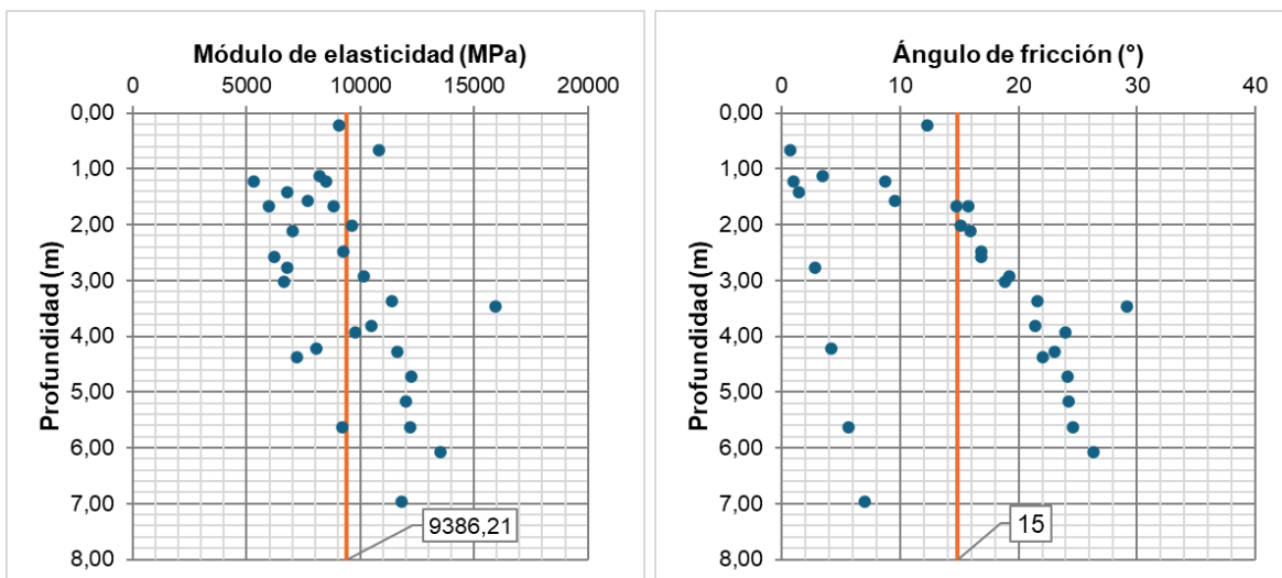
Figura 5.1.7.53 Depósito coluvial: Análisis de las correlaciones entre el SPT y el módulo de elasticidad (izquierda); el SPT y el ángulo de fricción (derecha)
