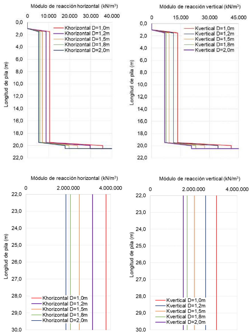
Figura 5.1.7.206 Módulo de balasto vertical y horizontal pilas – CIP Tanks. Las gráficas superiores representan los módulos de balasto hasta una longitud de 22,0 m y las gráficas inferiores los módulos de balasto para longitudes entre 22,0 m y 30,0 m
