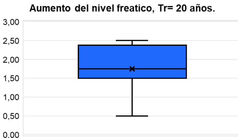
Figura 5.1.7.128 Análisis estadístico por medio del diagrama de cajas y bigotes de los datos obtenidos para el incremento del nivel freático extremo (Tr=20 años)
