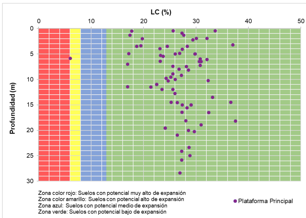
Figura 5.1.7.46 Resultados límites de contracción en la Plataforma Principal
