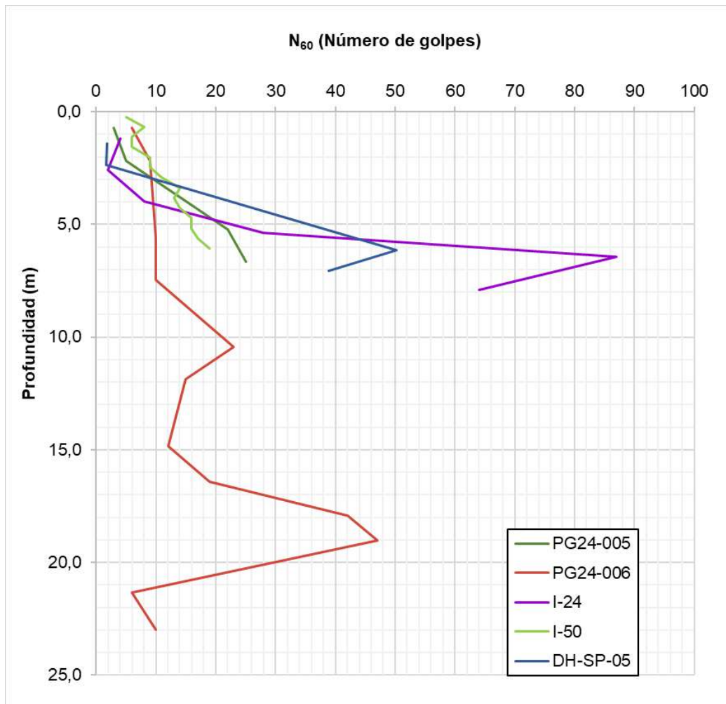
Figura 5.1.7.21 Análisis para las pruebas in situ SPT realizadas para los 5 sondajes en la zona de la presa del sedimentador La Colorada
