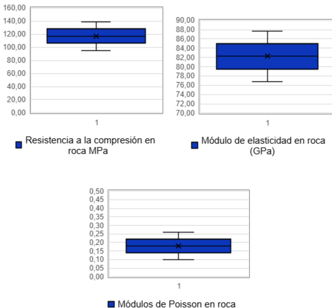
Figura 5.1.7.91 Horizonte I: Análisis de la compresión simple (datos 2), módulo de elasticidad (datos 2), relación de Poisson (datos 2)
