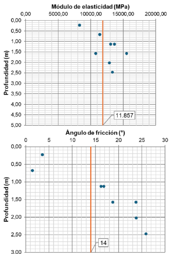
Figura 5.1.7.62 Depósito de Flujo: Análisis de las correlaciones entre el SPT y el módulo de elasticidad (izquierda); el SPT y el ángulo de fricción (derecha)
