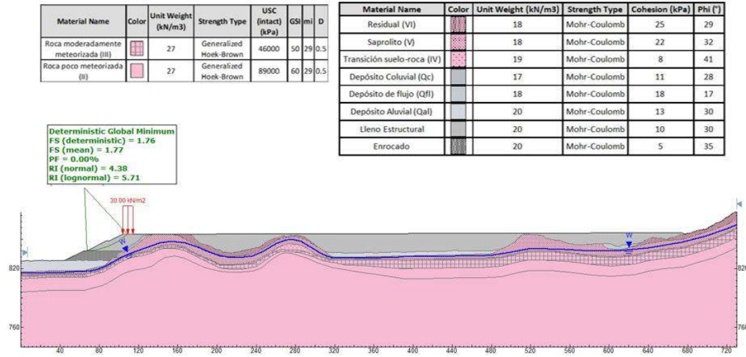
Figura 5.1.7.123 Análisis de estabilidad en condición estática con nivel freático normal de la sección E
