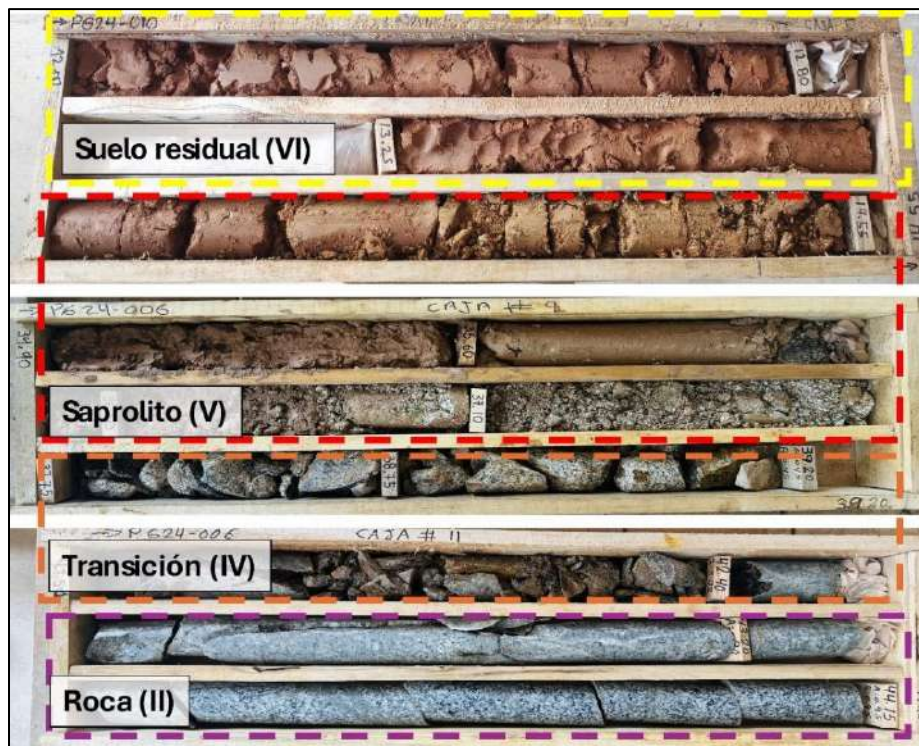
Figura 5.1.7.76 Perfil de meteorización típico en las granodioritas del Batolito Antioqueño, en el área de la Planta Principal (Perforación PG24-006)
