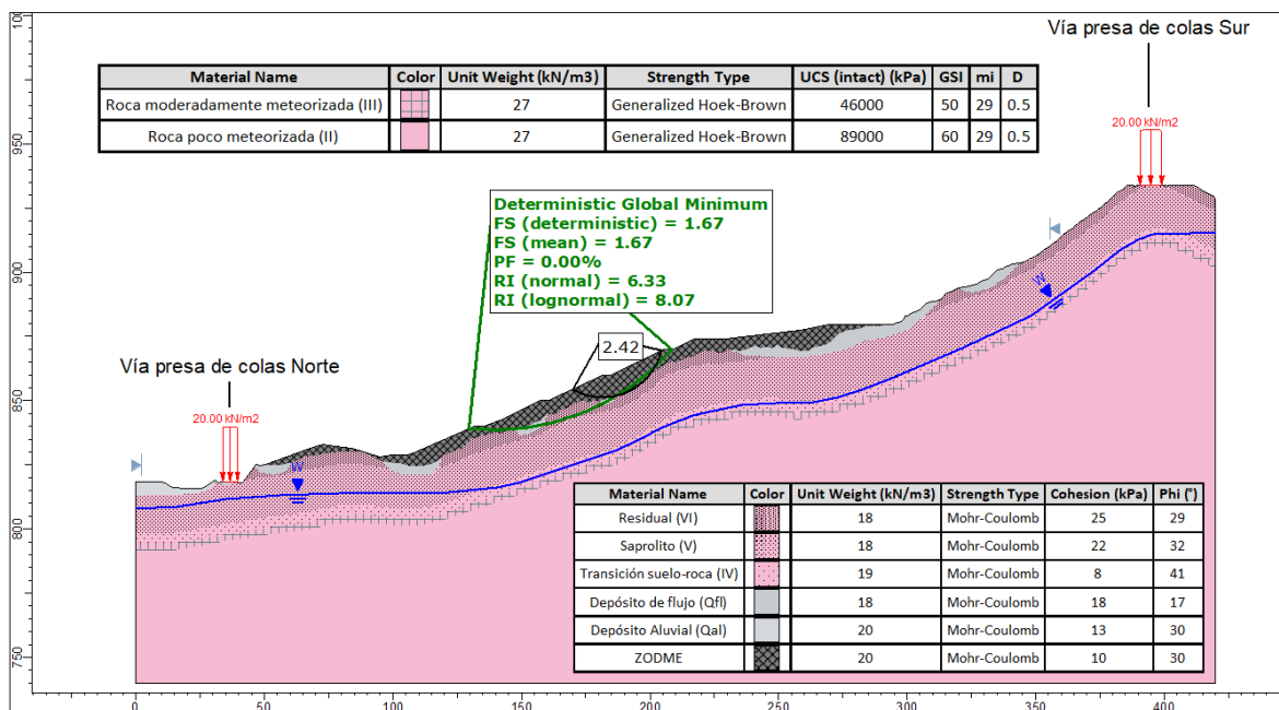
Figura 5.1.7.152 Análisis de estabilidad en condición estática con nivel freático normal de la Sección B – Depósito G
