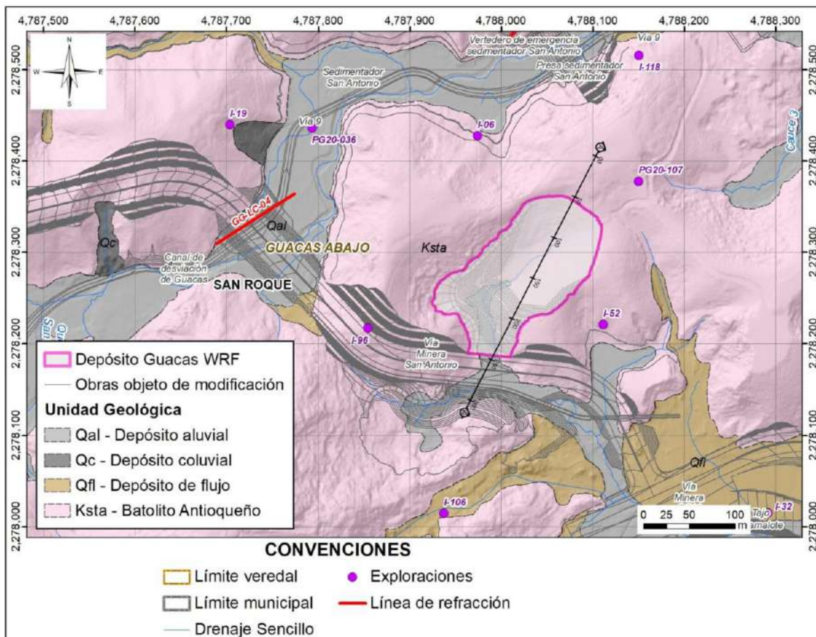
Figura 5.1.7.168 Localización en planta del depósito Guacas WRF con la sección de interés para el análisis geotécnico
