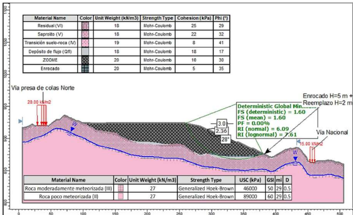
Figura 5.1.7.158 Análisis de estabilidad en condición estática con nivel freático normal de la Sección A – Depósito L
