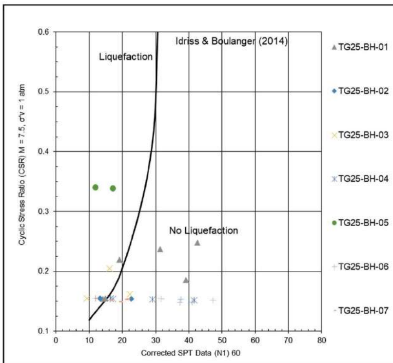
Figura 5.1.7.75 Análisis de licuación o licuefacción de muestras de suelo – Depósito El Balsal. Método de Idriss y Boulanger (2010-2012) basado en el ensayo SPT
