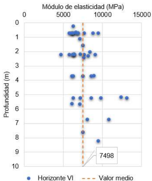
Figura 5.1.7.41 Horizonte VI: Análisis de las correlaciones entre el SPT y el módulo de elasticidad
