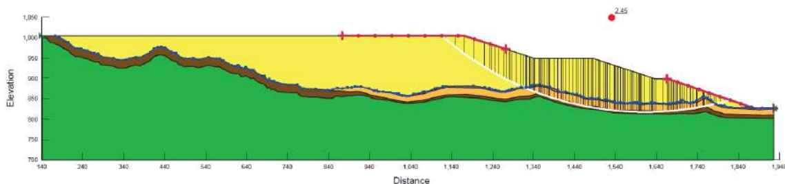
Figura 5.5.1.7.177 Análisis de estabilidad al cierre en condición estática de la Sección A – Depósito San Antonio, etapa de cierre
