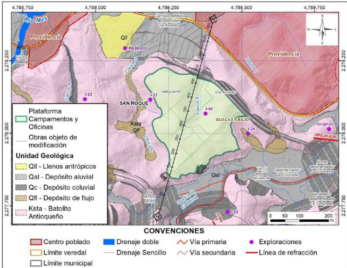
Figura 5.1.7.129 Localización en planta de la plataforma de campamentos y oficinas con la sección de interés para el análisis geotécnico
