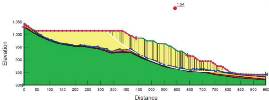
Figura 5.5.1.7.180 Análisis de estabilidad en condición estática de la Sección B – Depósito El Balsal, etapa de operación máxima
