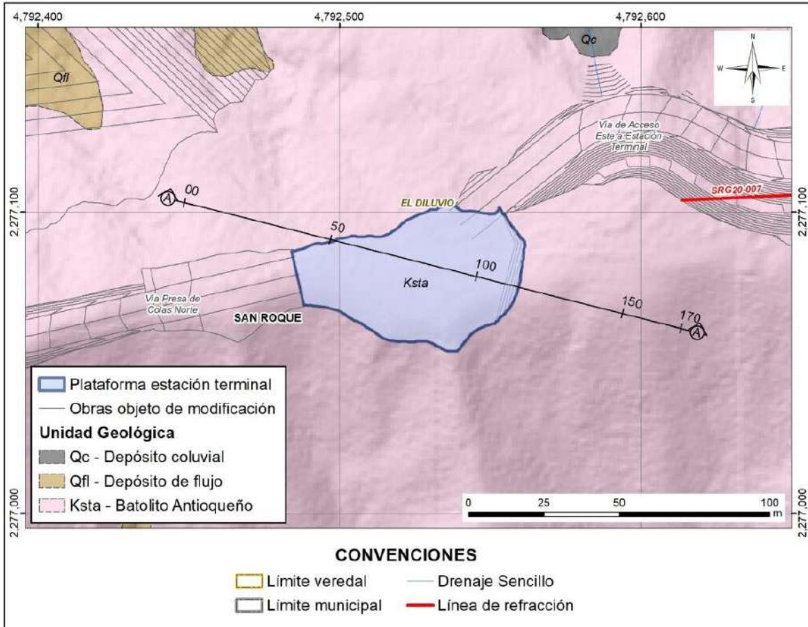
Figura 5.1.7.138 Localización en planta de la plataforma Estación Terminal con la sección de interés para el análisis geotécnico
