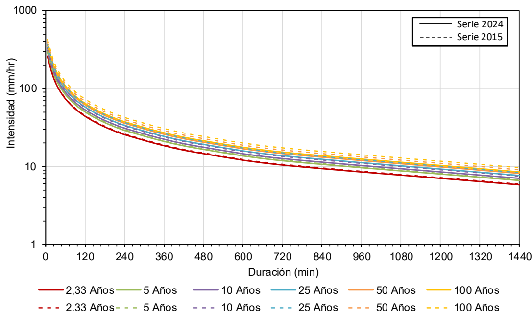
Figura 5.1.7.99 Comparación de IDF actual vs IDF EIA 2015 de la estación San Roque.
