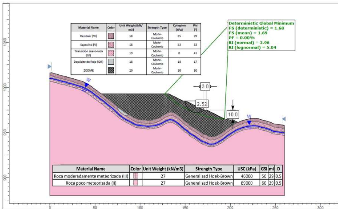
Figura 5.1.7.154 Análisis de estabilidad en condición estática con nivel freático normal de la Sección A – Depósito K
