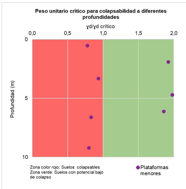
Figura 5.1.7.55 Resultados de colapsabilidad en las plataformas menores
