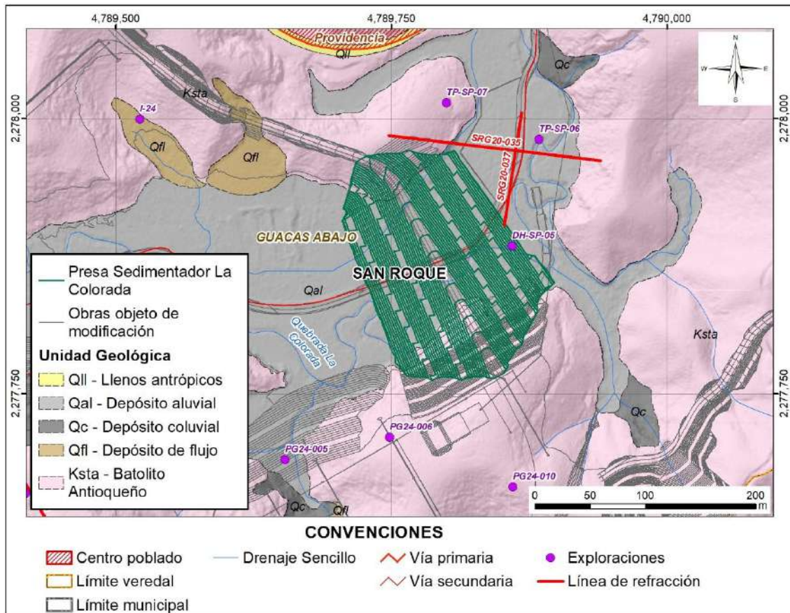
Figura 5.1.7.20 Localización en planta de la presa del sedimentador La Colorada
