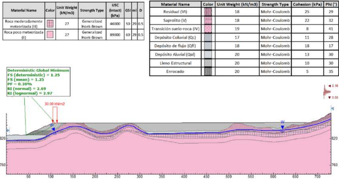
Figura 5.1.7.126 Análisis de estabilidad en condición seudo estática para un periodo de retorno de 475 años de la sección E
