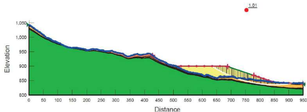
Figura 5.5.1.7.184 Análisis de estabilidad al cierre en condición pseudoestática de la Sección B – Depósito El Balsal, etapa de cierre
