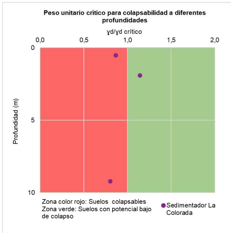
Figura 5.1.7.28 Resultados de colapsabilidad-Sector La Colorada
