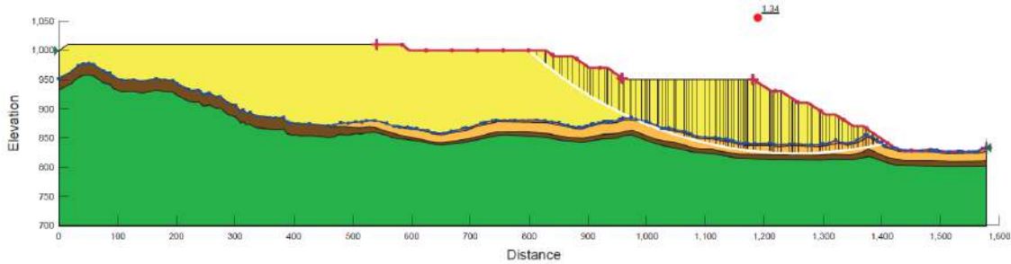
Figura 5.5.1.7.176 Análisis de estabilidad en condición post-pico de la Sección A – Depósito San Antonio, operación máxima
