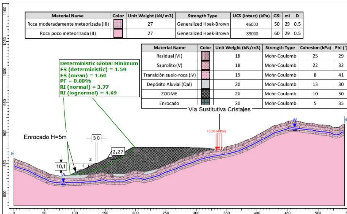
Figura 5.1.7.160 Análisis de estabilidad en condición estática con nivel freático normal de la Sección A – Depósito M
