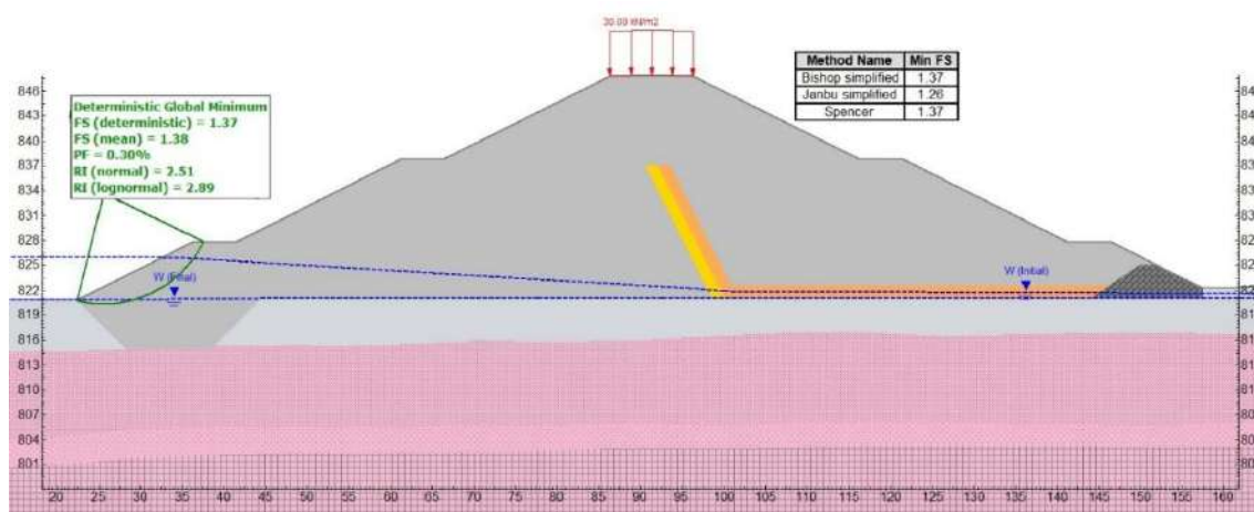
Figura 5.1.7.109 Grado de estabilidad del espaldón aguas arriba de la presa del sedimentador La Colorada ante el escenario de desembalse rápido
