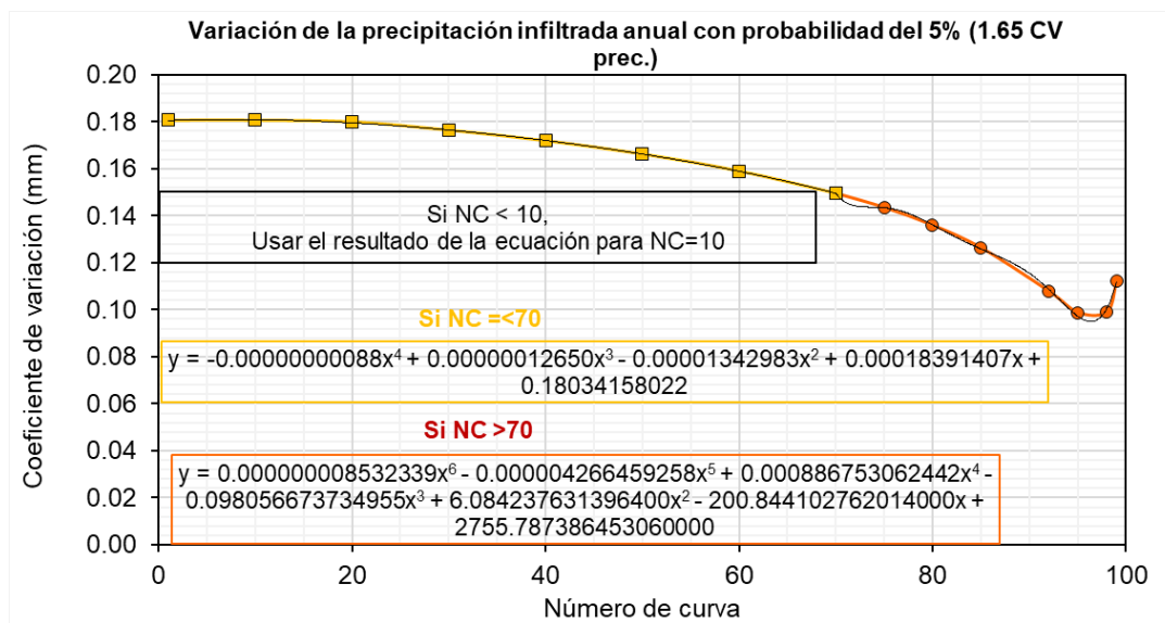
Figura 5.1.7.102 Curva de estimación de la variación de la precipitación infiltrada anual con probabilidad del 5% - Estación San Roque
