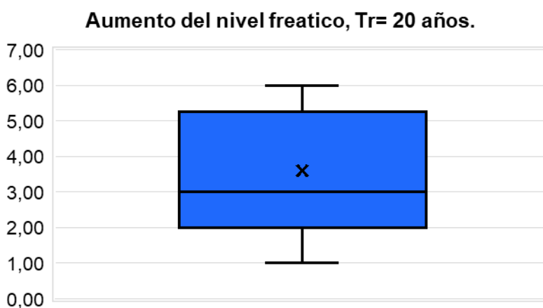
Figura 5.1.7.147 Análisis estadístico por medio del diagrama de cajas y bigotes de los datos obtenidos para el incremento del nivel freático extremo ( T_r=20 años)
