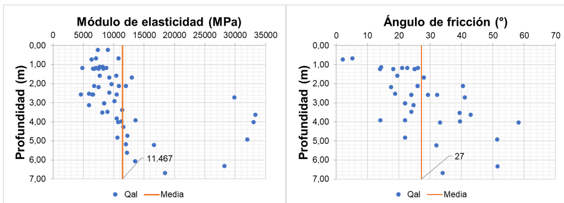
Figura 5.1.7.35 Depósito aluvial: Análisis de las correlaciones entre el SPT y el módulo de elasticidad (izquierda); el SPT y el ángulo de fricción (derecha)
