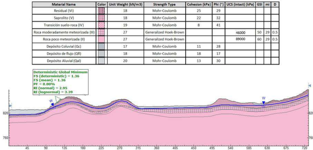
Figura 5.1.7.122 Análisis de estabilidad en condición estática del terreno natural de la sección E
