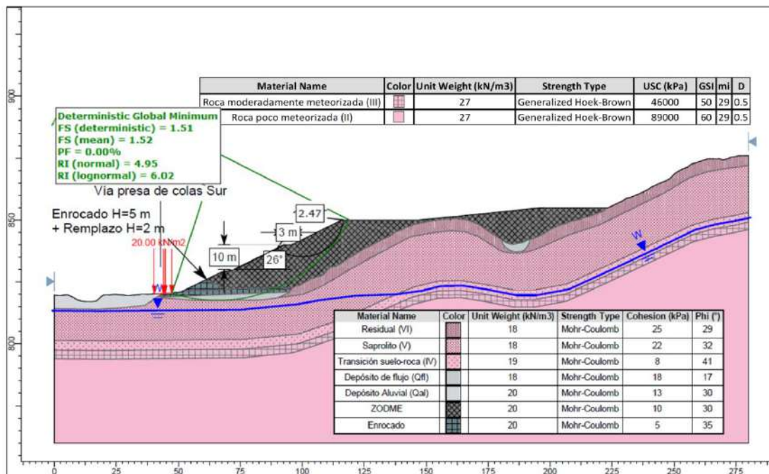
Figura 5.1.7.151 Análisis de estabilidad en condición estática con nivel freático normal de la Sección A – Depósito G
