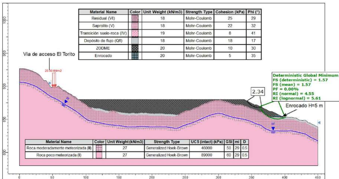
Figura 5.1.7.165 Análisis de estabilidad en condición estática con nivel freático normal de la Sección A – Depósito R
