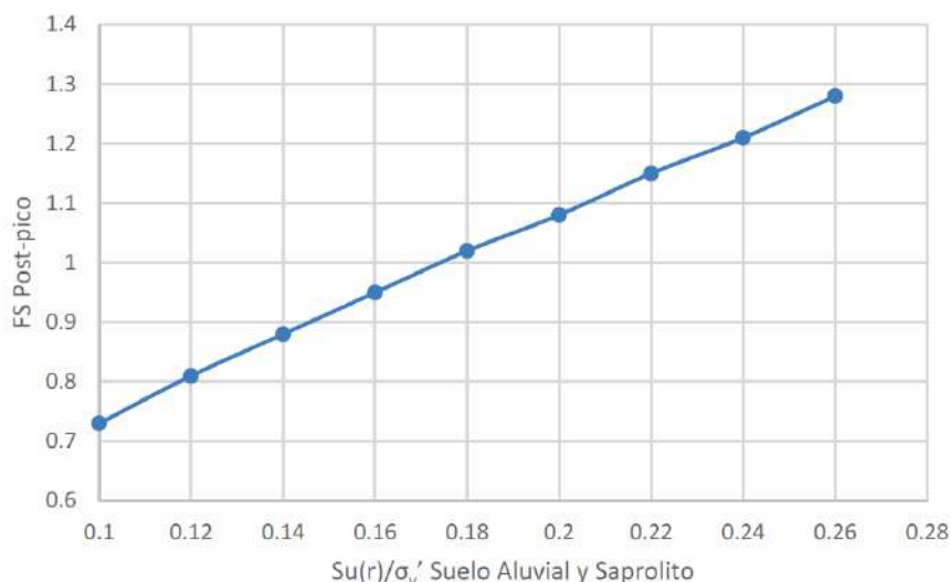
Figura 5.5.1.7.195 Análisis de sensibilidad post-pico – Presa Sedimentador San Antonio
