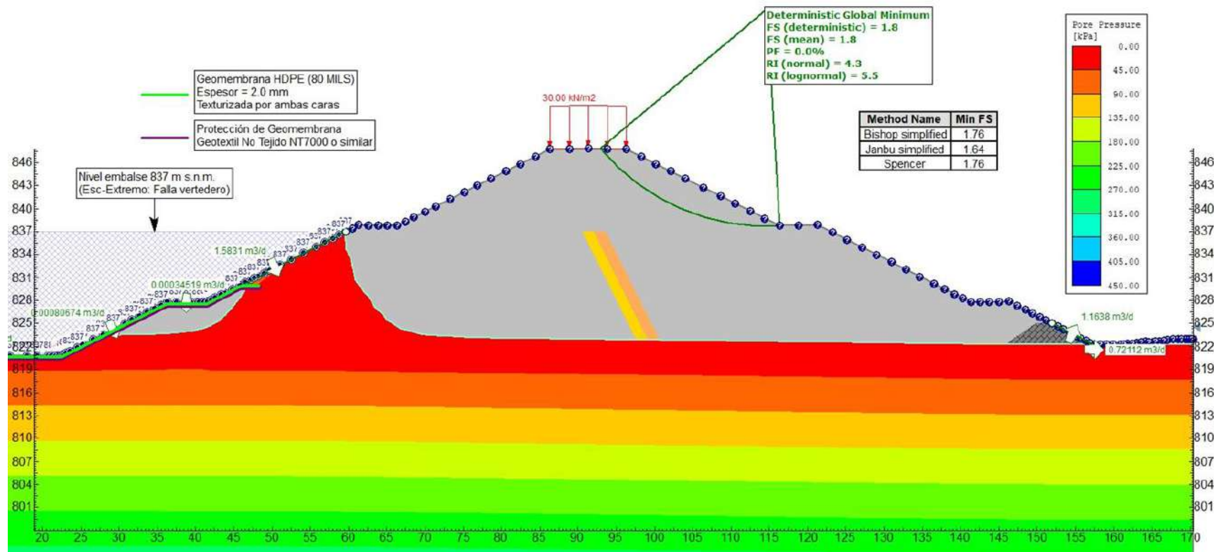
Figura 5.1.7.117 Comportamiento hidráulico de la presa del sedimentador La Colorada. Presiones de poros y condición de estabilidad espaldón aguas abajo. Condición extrema: fallo del vertedero de excesos. Sección B – km 0+820
