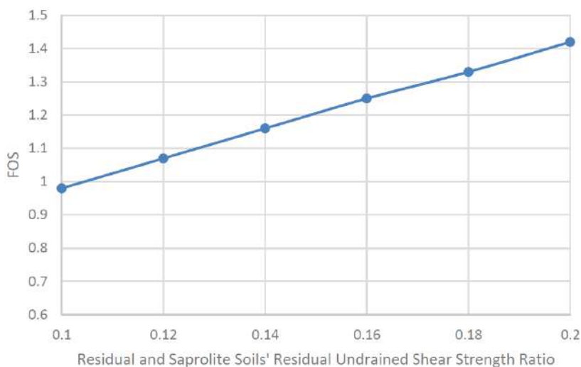
Figura 5.5.1.7.197 Análisis de sensibilidad post-pico al cierre – Depósito San Antonio
