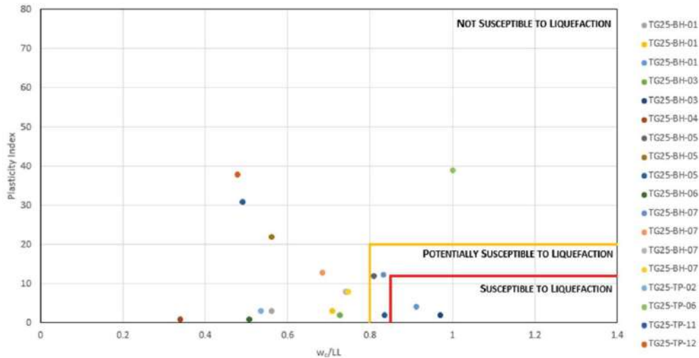
Figura 5.1.7.73 Análisis de licuación o licuefacción de muestras de suelo residual – El Balsal. Método de Bray y Sancio (2006)
