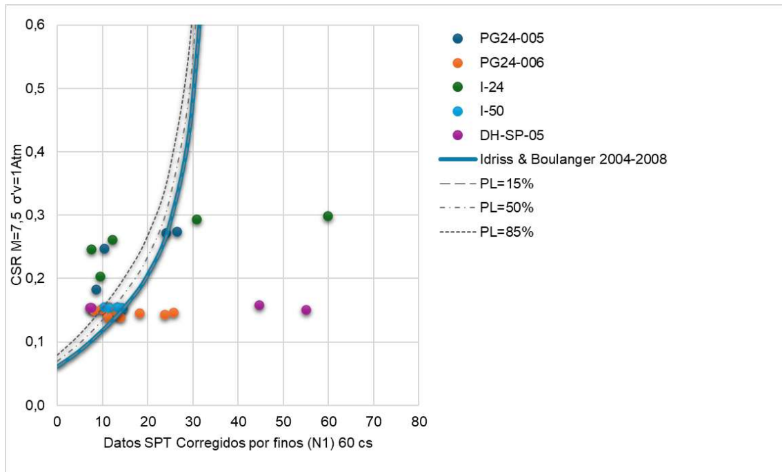
Figura 5.1.7.30 Análisis de licuación o licuefacción de muestras de suelo – Sedimentador La Colorada. Método de Idriss y Boulanger (2010-2012) basado en el ensayo SPT
