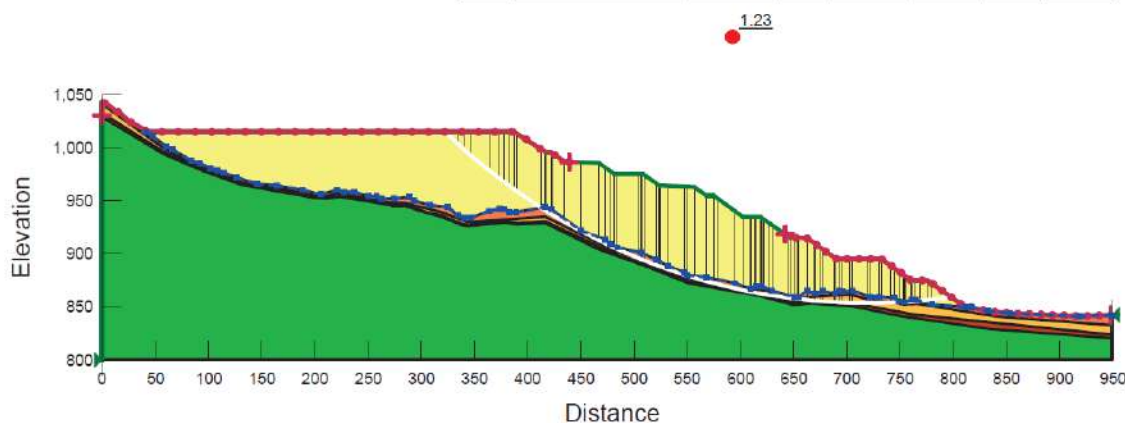
Figura 5.5.1.7.182 Análisis de estabilidad en condición post-pico de la Sección B – Depósito El Balsal, etapa de operación máxima
