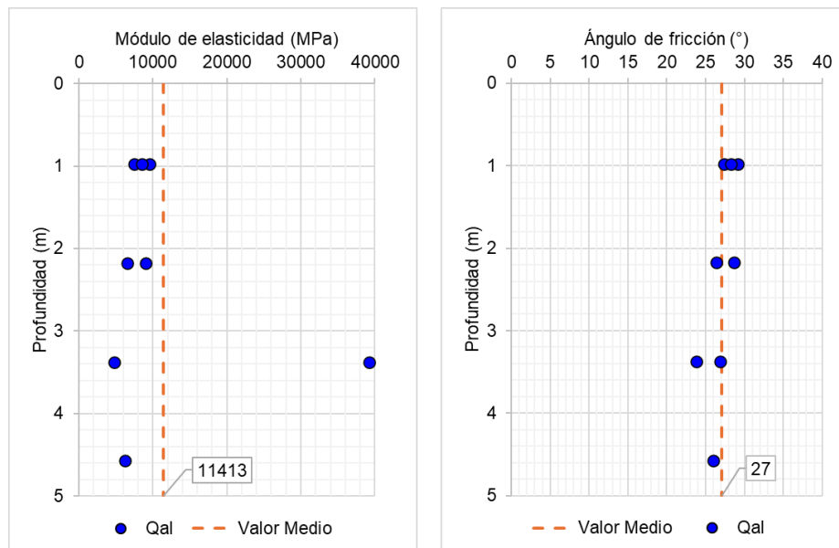
Figura 5.1.7.68 Depósito Aluvial: Análisis de las correlaciones entre el SPT y el módulo de elasticidad (izquierda); SPT y el ángulo de fricción (derecha)
