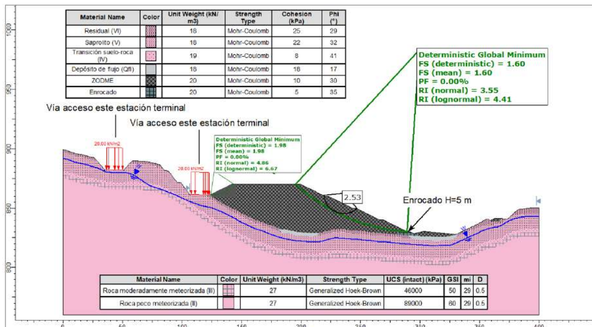
Figura 5.1.7.162 Análisis de estabilidad en condición estática con nivel freático normal de la Sección A – Depósito O
