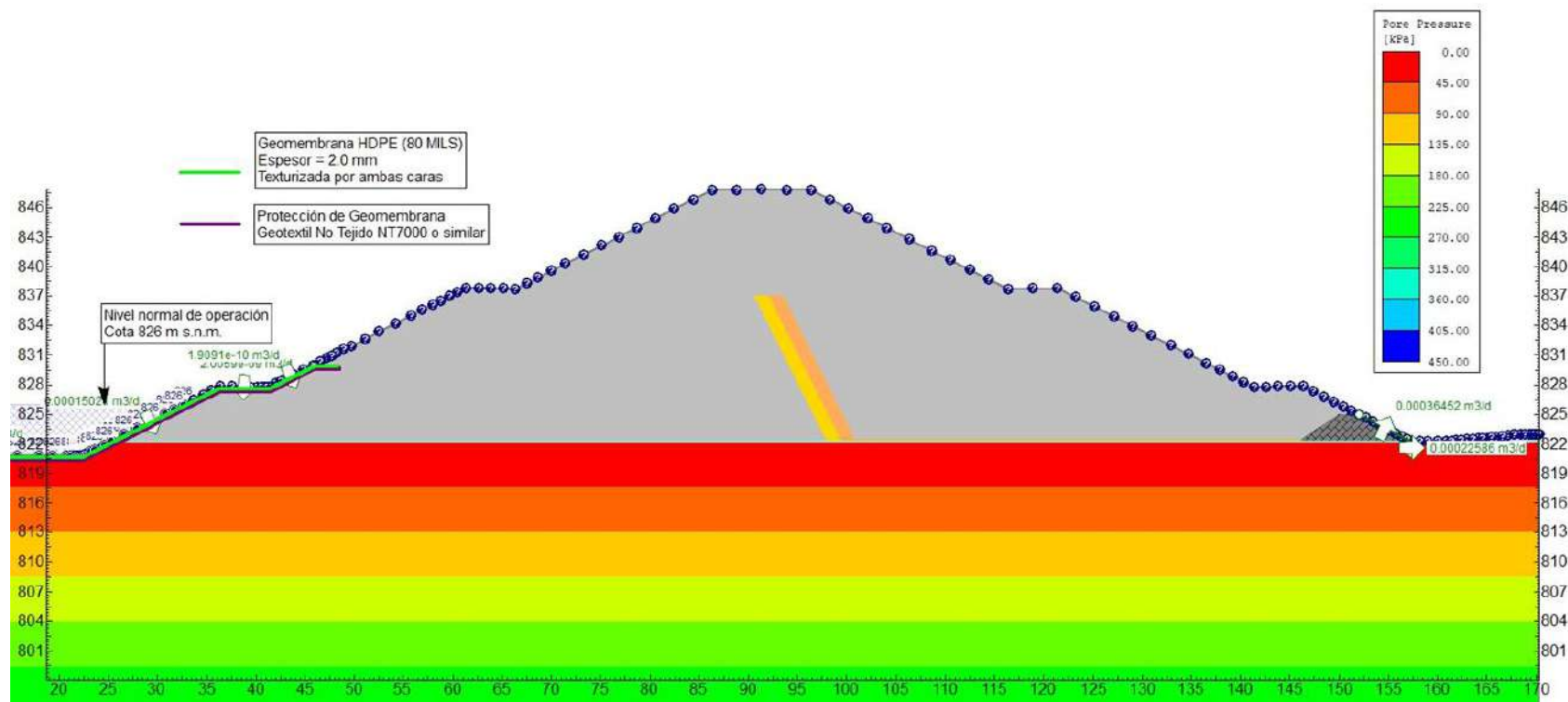
Figura 5.1.7.114 Comportamiento hidráulico de la presa del sedimentador La Colorada. Presiones de poros. Condición nivel normal de operación del embalse. Sección B – km 0+820
