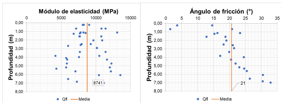
Figura 5.1.7.36 Depósito de flujo: Análisis de las correlaciones entre el SPT y el módulo de elasticidad (izquierda); el SPT y el ángulo de fricción (derecha).
