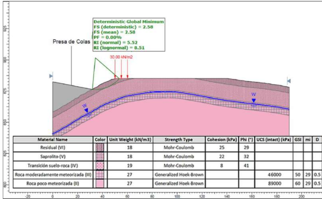
Figura 5.1.7.137 Análisis de estabilidad en condición estática con nivel freático normal de la plataforma de la Estación de Regulación
