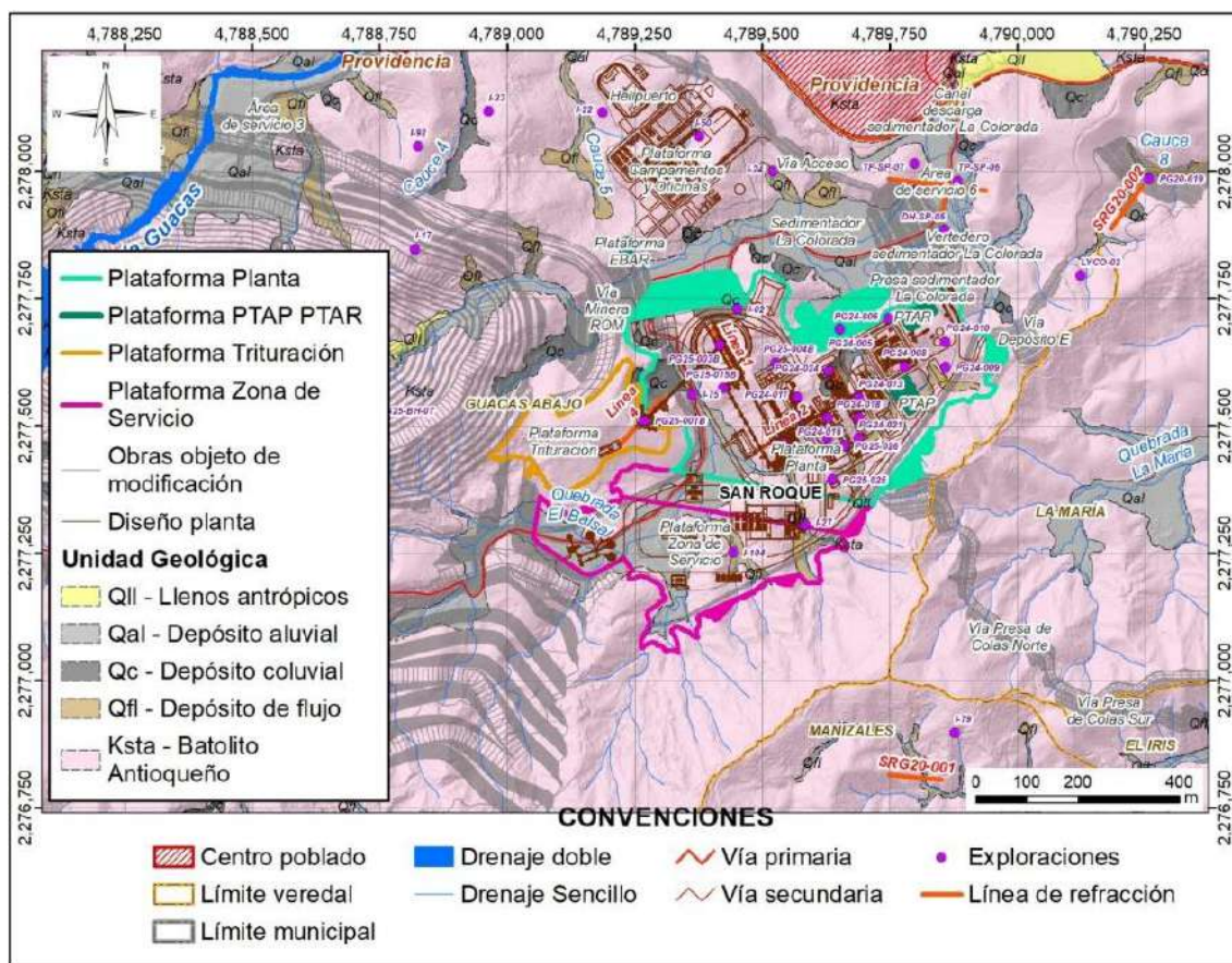
Figura 5.1.7.39 Localización en planta de la Plataforma Principal del proyecto Gramalote
