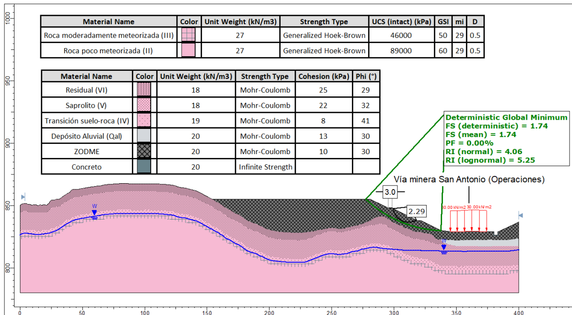
Figura 5.1.7.169 Análisis de estabilidad en condición estática con nivel freático normal de la Sección A – Depósito Guacas WRF
