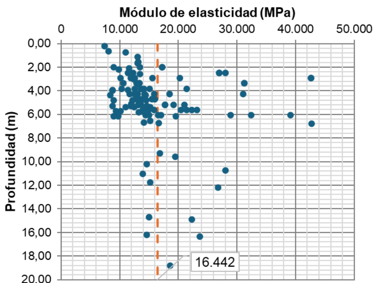
Figura 5.1.7.59 Horizonte V: Análisis de las correlaciones entre el SPT y el módulo de elasticidad
