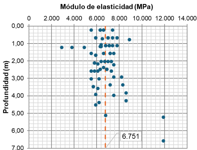
Figura 5.1.7.58 Horizonte VI: Análisis de las correlaciones entre el SPT y el módulo de elasticidad
