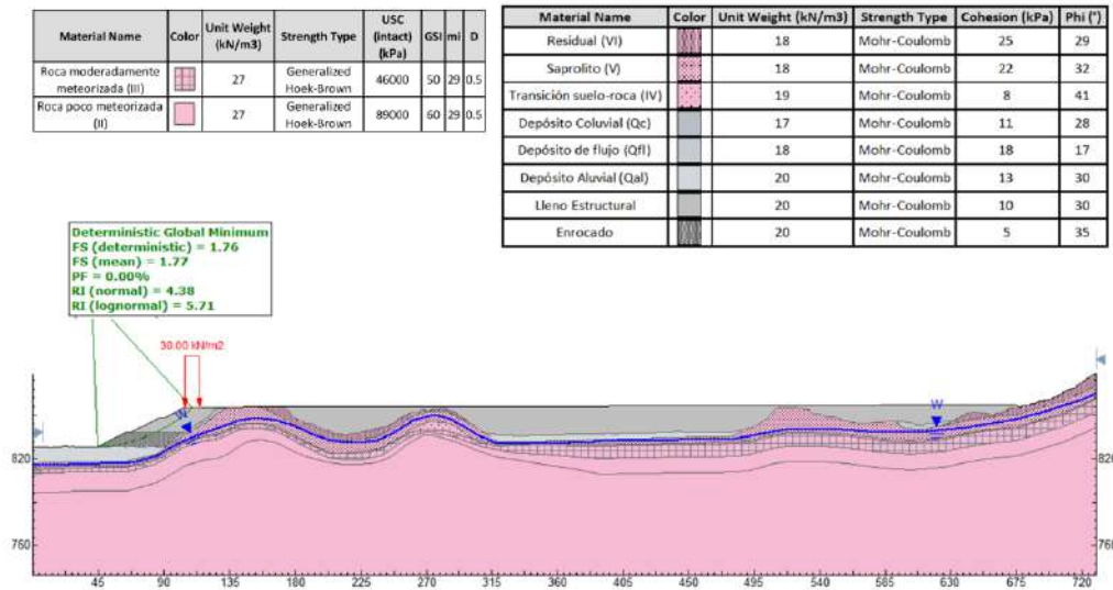
Figura 5.1.7.124 Análisis de estabilidad en condición estática con nivel freático extremo de la sección E
