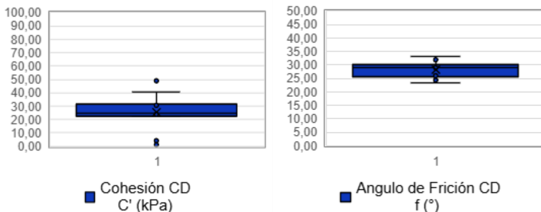
Figura 5.1.7.85 Horizonte VI: Análisis del ángulo de fricción y cohesión en la base de datos general. Número de datos 8
