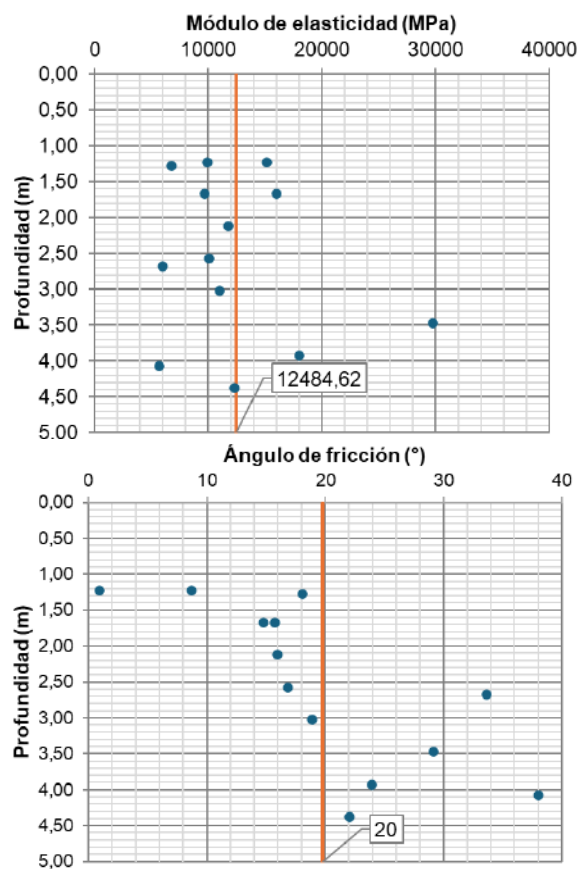
Figura 5.1.7.61 Depósito Coluvial: Análisis de las correlaciones entre el SPT y el módulo de elasticidad (izquierda); el SPT y el ángulo de fricción (derecha)
