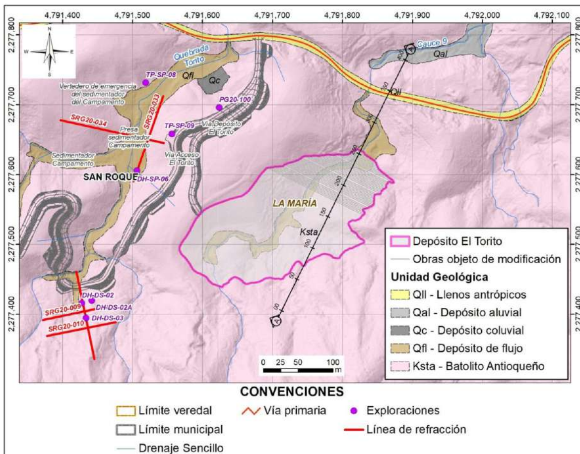
Figura 5.1.7.170 Localización en planta del depósito El Torito con la sección de interés para el análisis geotécnico
