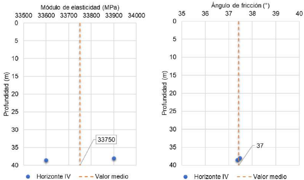
Figura 5.1.7.26 Horizonte IV (transición suelo-roca): Análisis de las correlaciones entre el SPT y el módulo de elasticidad (izquierda); el SPT y el ángulo de fricción (derecha)
