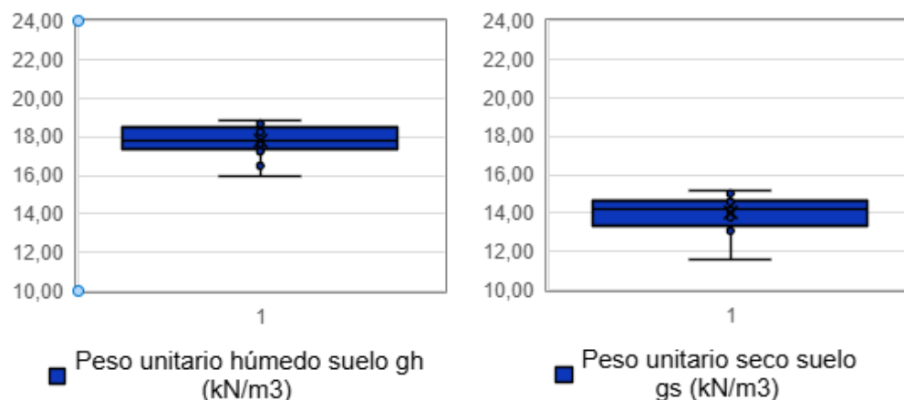
Figura 5.1.7.83 Horizonte VI: Análisis de los pesos unitarios reportados en la base de datos general. Número de datos 14 para el húmedo y 13 para el seco
