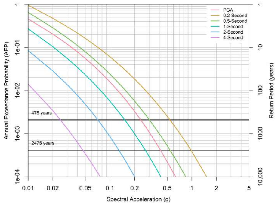
Figura 5.1.7.18 Curvas de amenaza media (5% de amortiguamiento) para los periodos espectrales seleccionados en el sitio de la mina Gramalote. El valor de Vs30 usado es de 800 m/s
