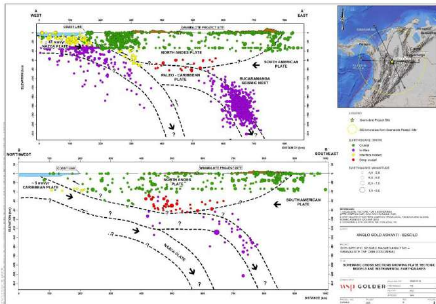
Figura 5.1.7.15 Secciones transversales esquemáticas que ilustran las principales características tectónicas y los hipocentros de los sismos históricos.
