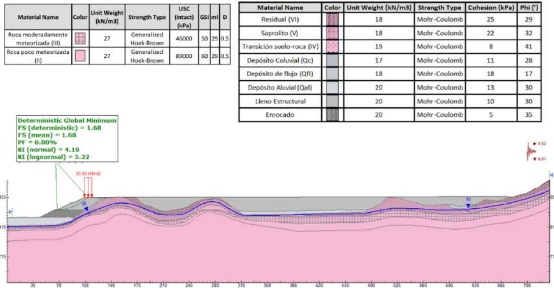
Figura 5.1.7.125 Análisis de estabilidad en condición seudo estática para un periodo de retorno de 50 años de la sección E
