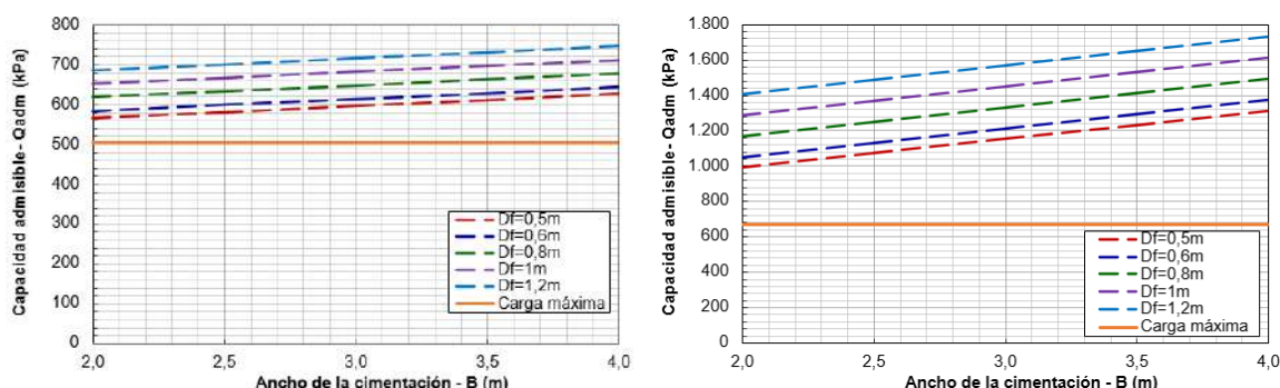
Figura 5.1.7.200 Ábaco capacidad de soporte admisible – Vertedero de excesos de la presa del sedimentador La Colorada – Servicio para el horizonte V (izquierda) y IV (derecha)
