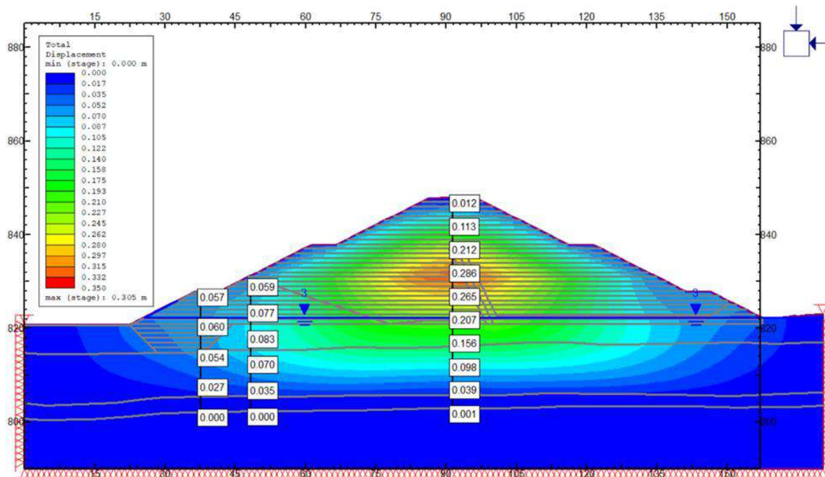
Figura 5.1.7.113 Desplazamientos totales – Sobrecarga vehicular. Presa del sedimentador La Colorada. Sección B – km 0+820
