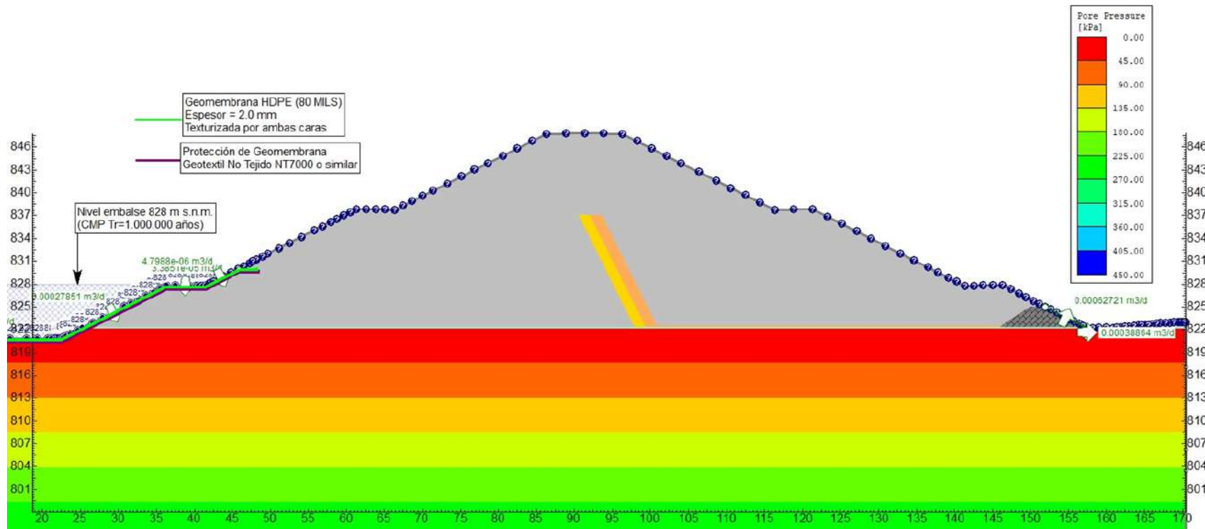
Figura 5.1.7.115 Comportamiento hidráulico de la presa del sedimentador La Colorada. Presiones de poros. Condición nivel del embalse ante crecienta máxima probable de diseño (CMP). Sección B – km 0+820
