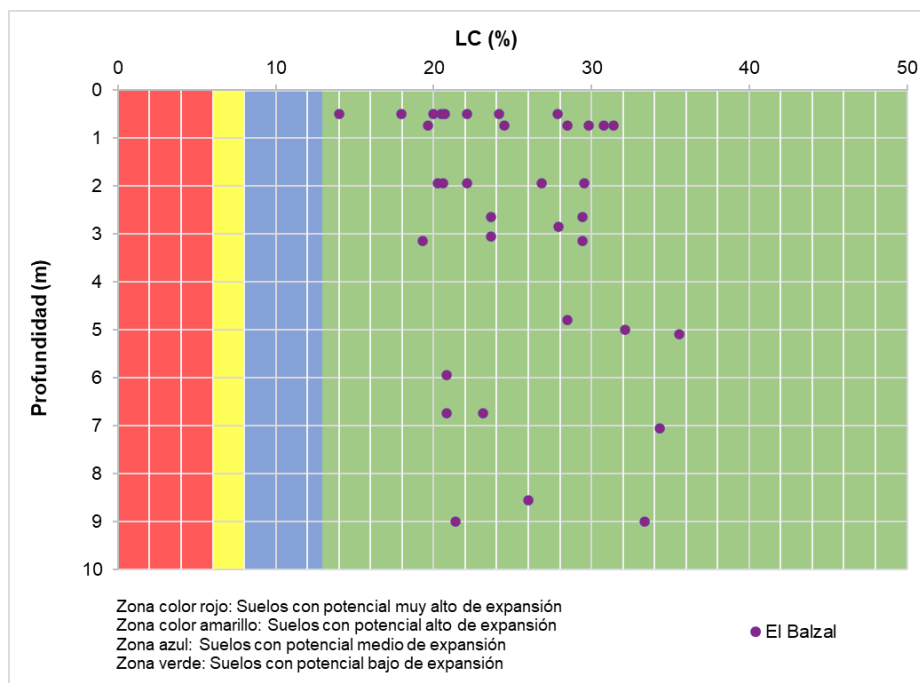
Figura 5.1.7.71 Resultados límites de contracción zona del Valle El Balsal
