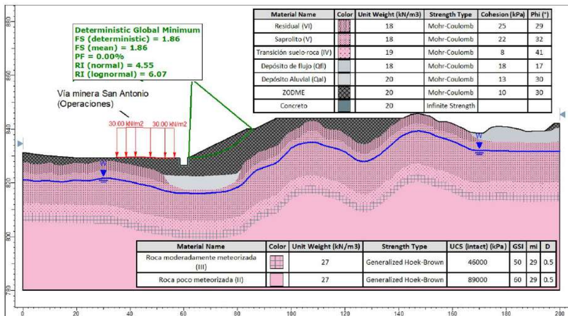
Figura 5.1.7.167 Análisis de estabilidad en condición estática con nivel freático normal de la Sección A – Depósito W
