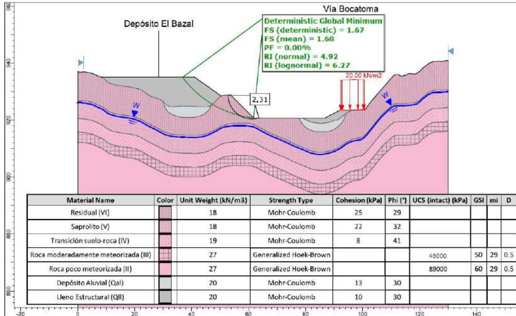
Figura 5.1.7.144 Análisis de estabilidad izquierdo en condición estática con nivel freático normal de la plataforma Polvorín
