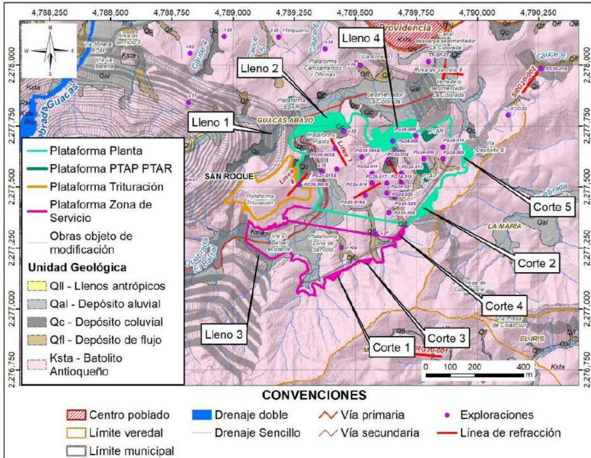
Figura 5.1.7.121 Localización en planta de la Plataforma Principal con la numeración de los taludes de corte y llenos analizados
