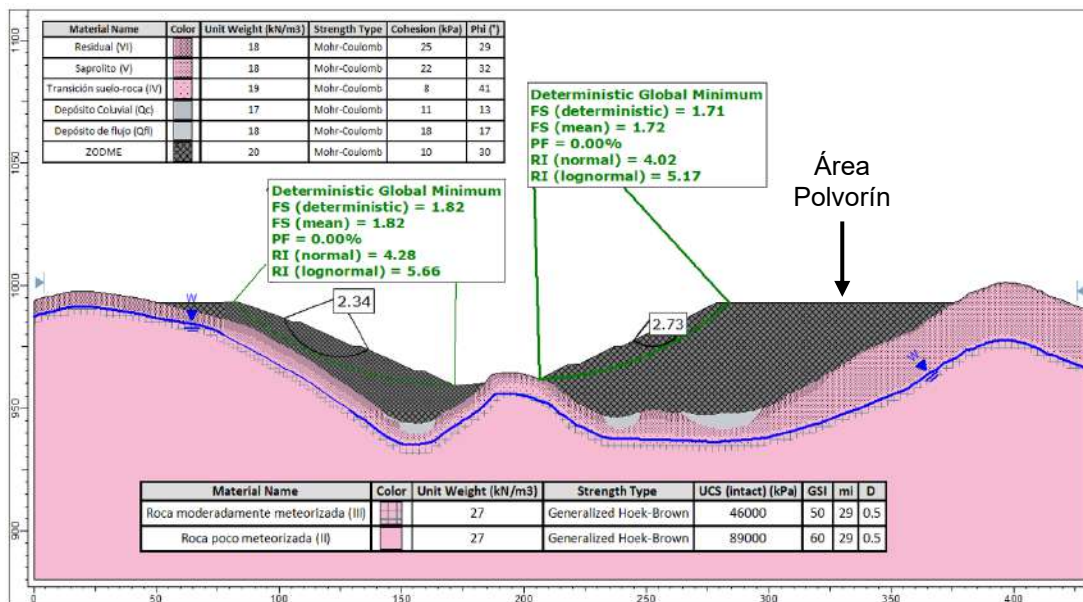
Figura 5.1.7.156 Análisis de estabilidad en condición estática con nivel freático normal de la Sección C – Depósito K (a la derecha se observa la terraza del depósito la cual será utilizada como “Área Polvorín”)
