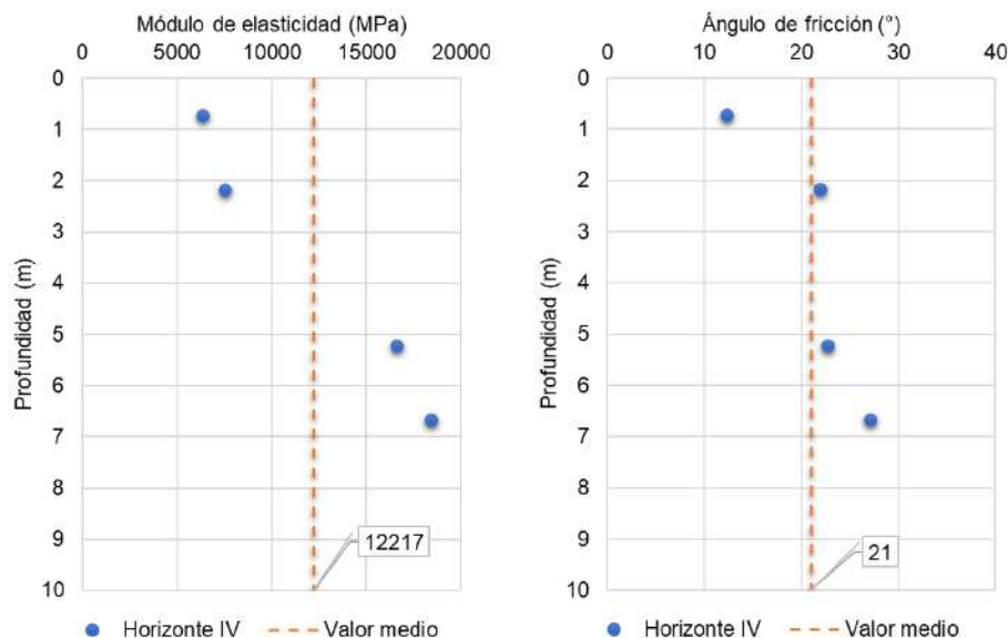
Figura 5.1.7.44 Depósito Aluvial: Análisis de las correlaciones entre el SPT y el módulo de elasticidad (izquierda); el SPT y el ángulo de fricción (derecha)
