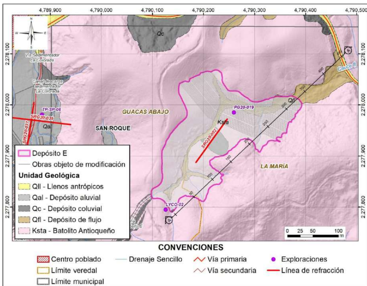
Figura 5.1.7.148 Localización en planta de la depósito E con la sección de interés para el análisis geotécnico
