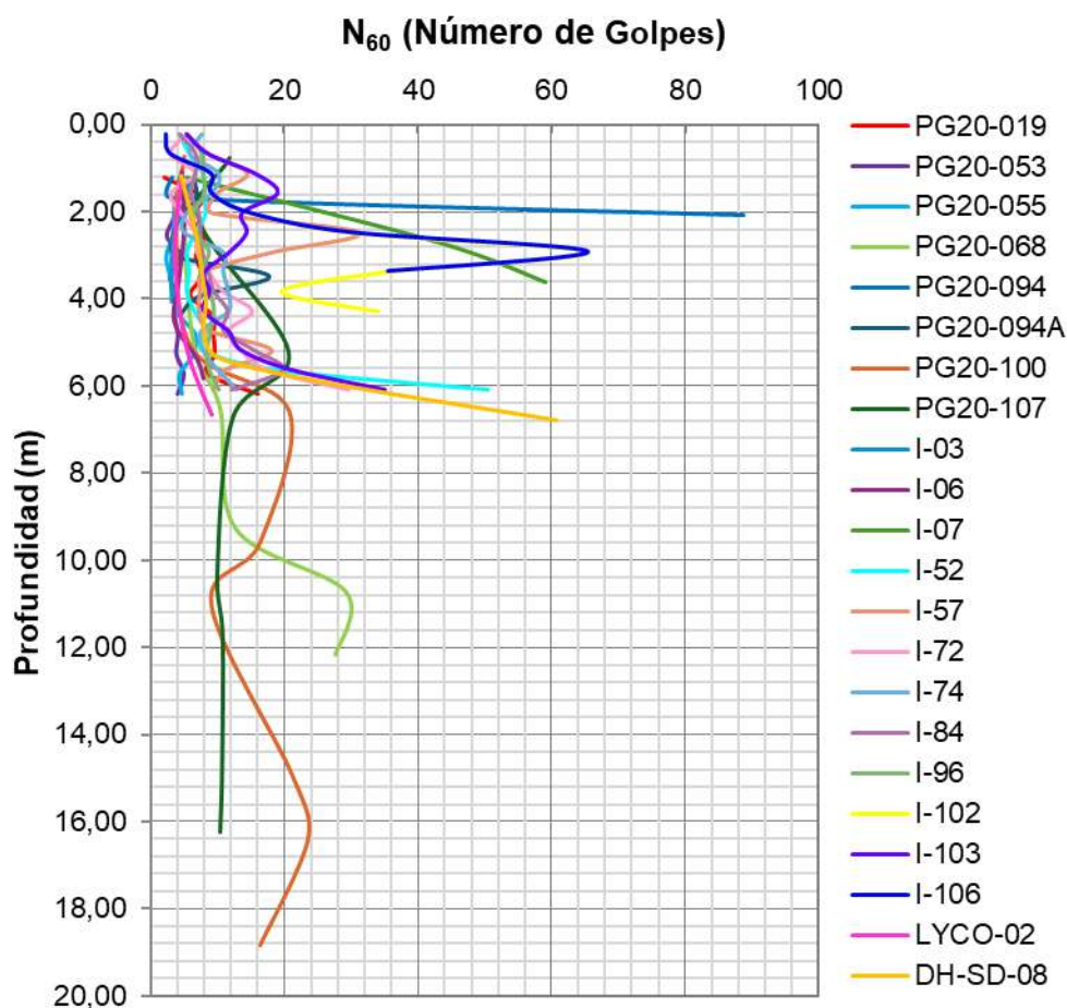
Figura 5.1.7.57 Análisis para las pruebas in situ SPT realizadas en las zonas de los depósitos
