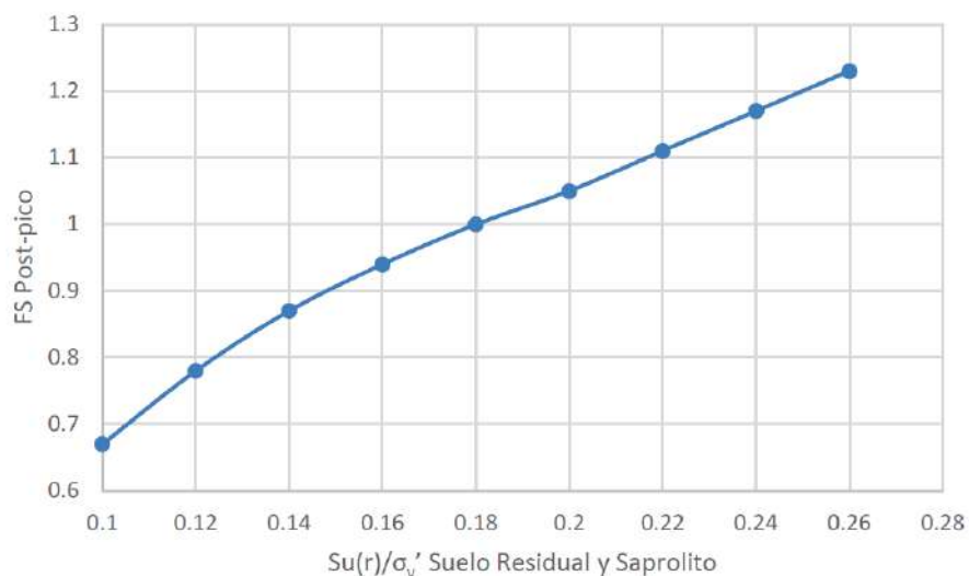
Figura 5.5.1.7.194 Análisis de sensibilidad post-pico – Depósito El Balsal
