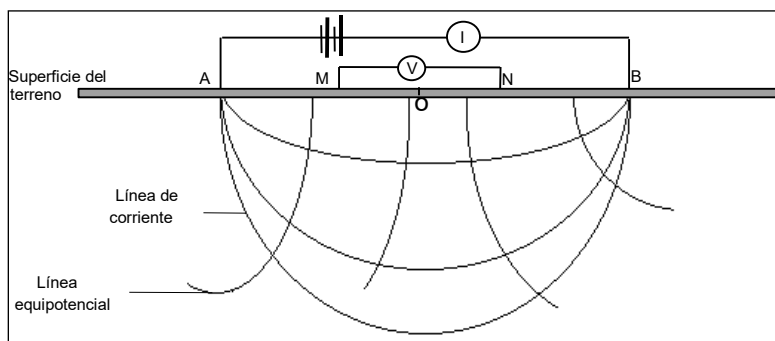
Figura 2.19 Esquema de la Configuración Electrónica Tipo Schlumberger para Ejecución de Sondeos Eléctricos Verticales – SEV
