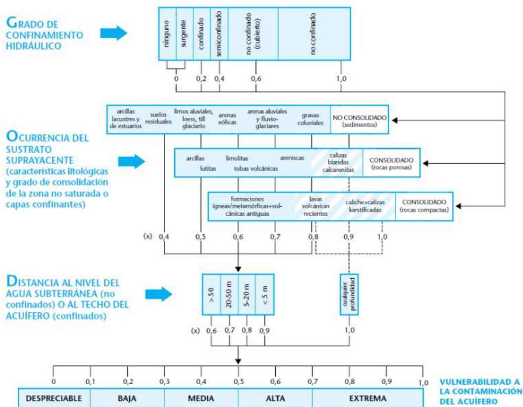
Figura 2.20 Método GOD para la evaluación de la vulnerabilidad intrínseca
