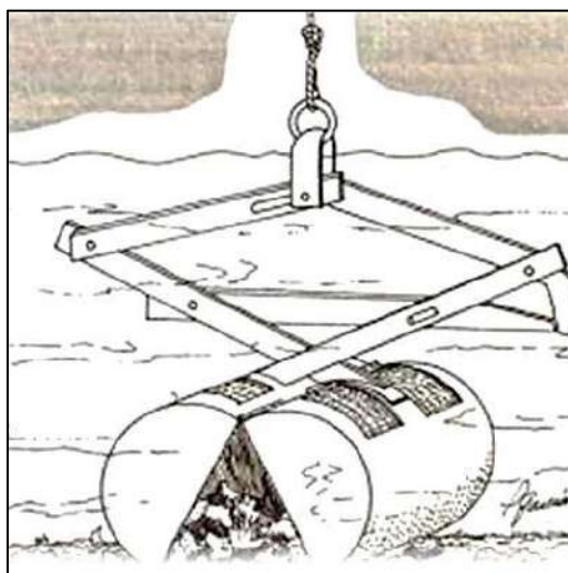
Figura 2.18 Esquema Dragas tipo Petersen
