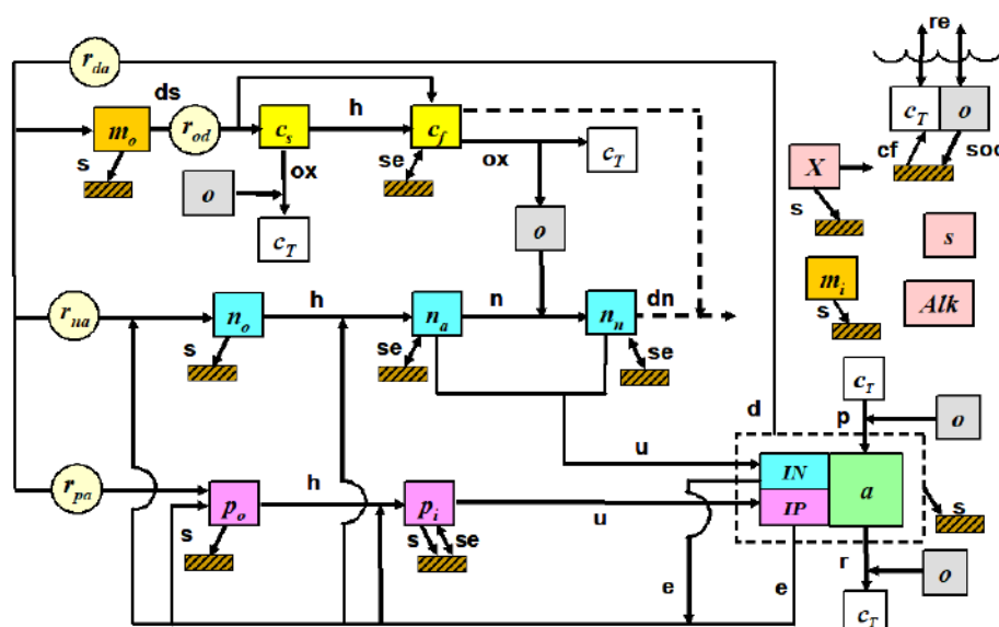
Figura 2.55 Modelos cinéticos y procesos de transferencia de masa
